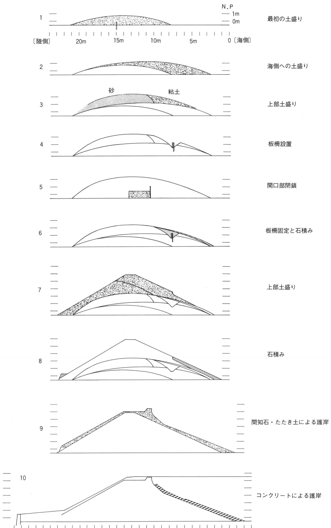
第16図 堤防構築模式図
