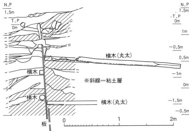
第10図 B区北面底辺板柵
