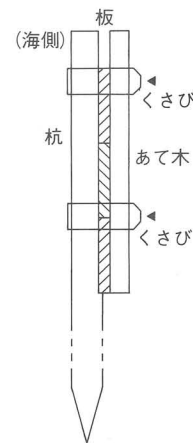
第7図 板柵の杭・あて木断面模式図
