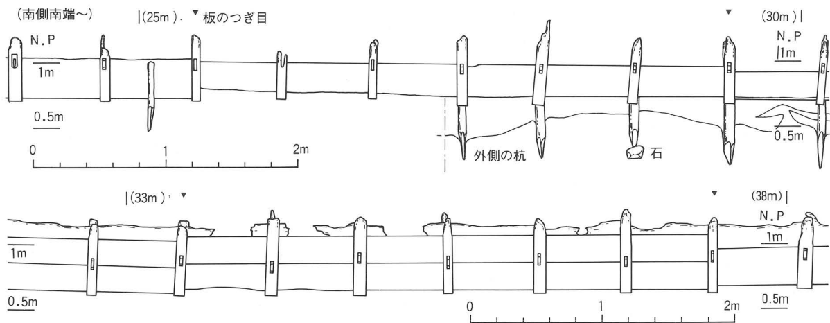
第6図 A区北側西区板柵列実測図
