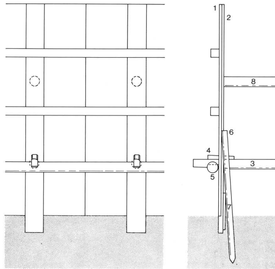
第11図 B区北面底辺板柵構造模式図
