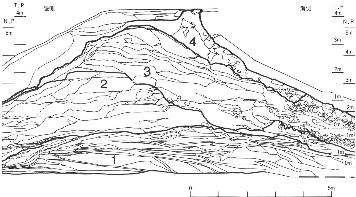
第12図 C区南面層序ブロック図
