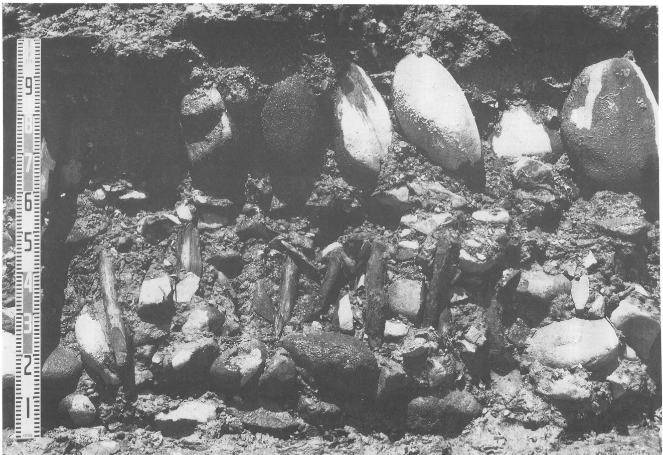
C区石積み下端（東から西を望む）
