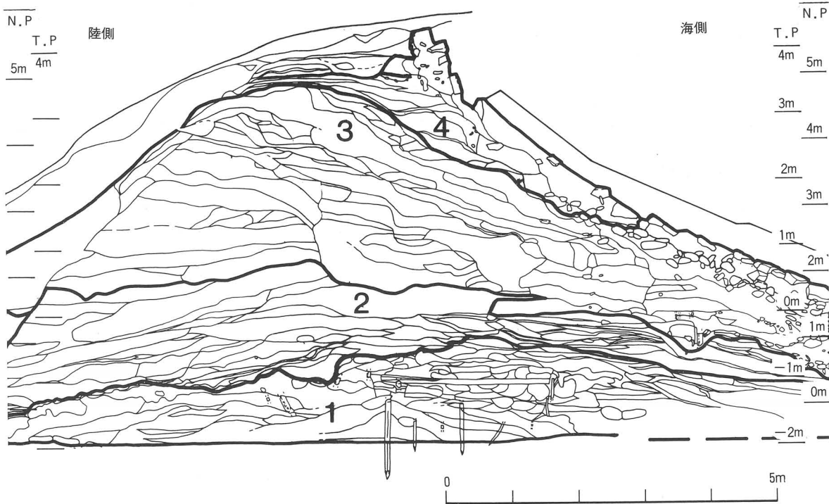
第9図 B区南面層序ブロック図
