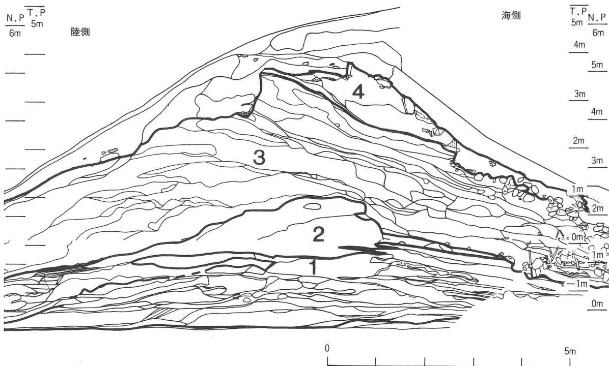
第5図 A区南面層序ブロック図
