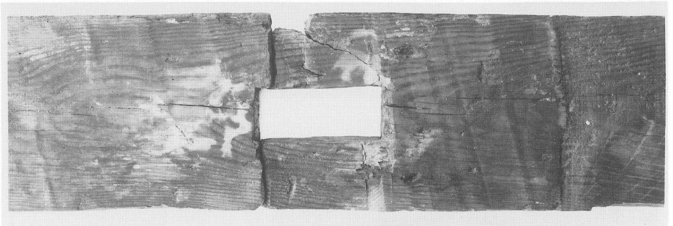
B区北面底辺板柵縦板のほぞ穴
