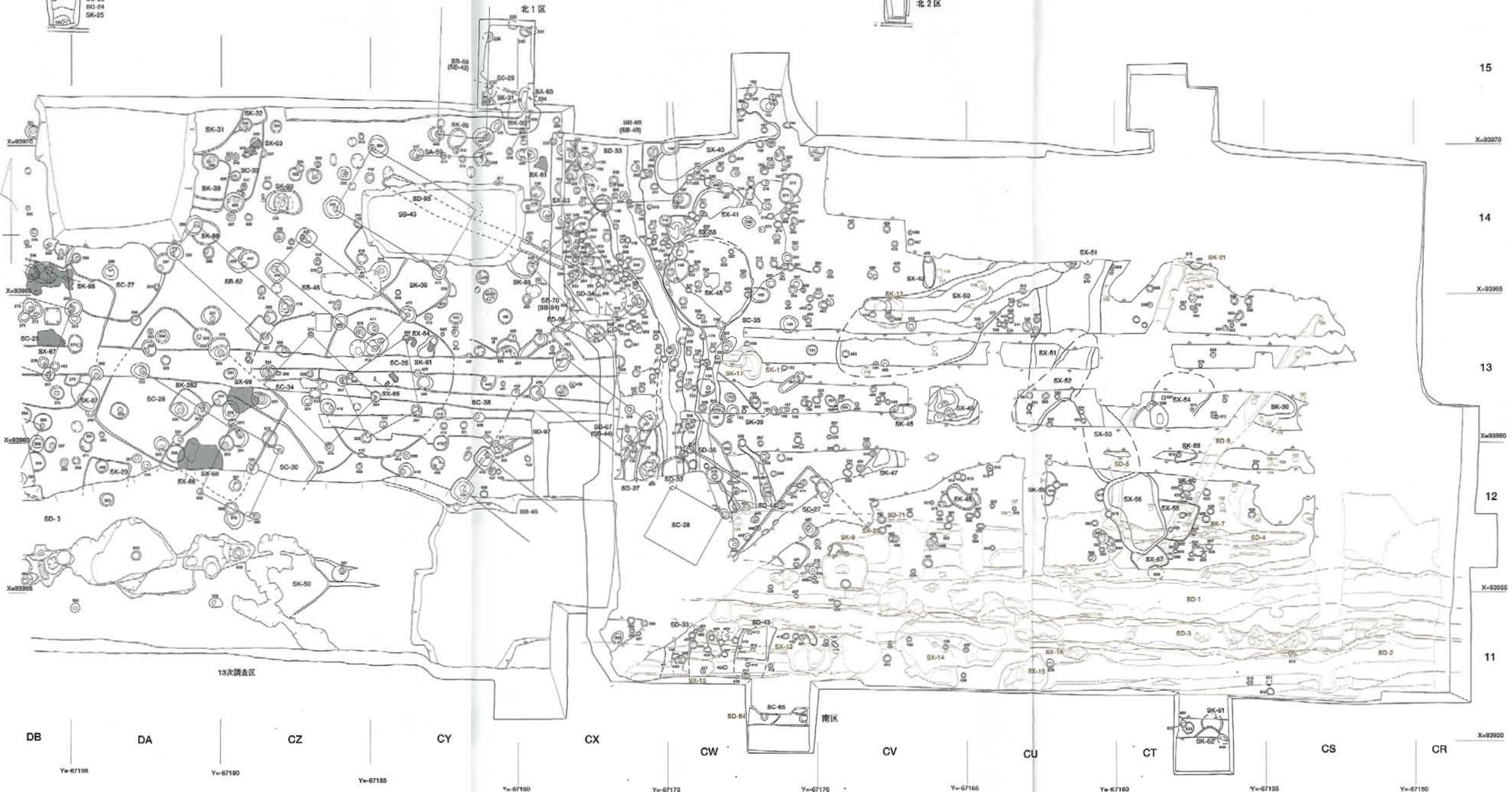
付図 文京遺跡20次調査遺構配置図 (縮尺1/100)
