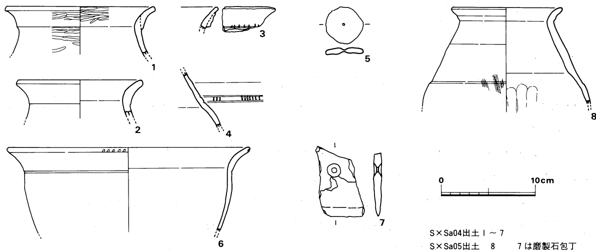
第40図 弥生時代前期包含層出土遺物
