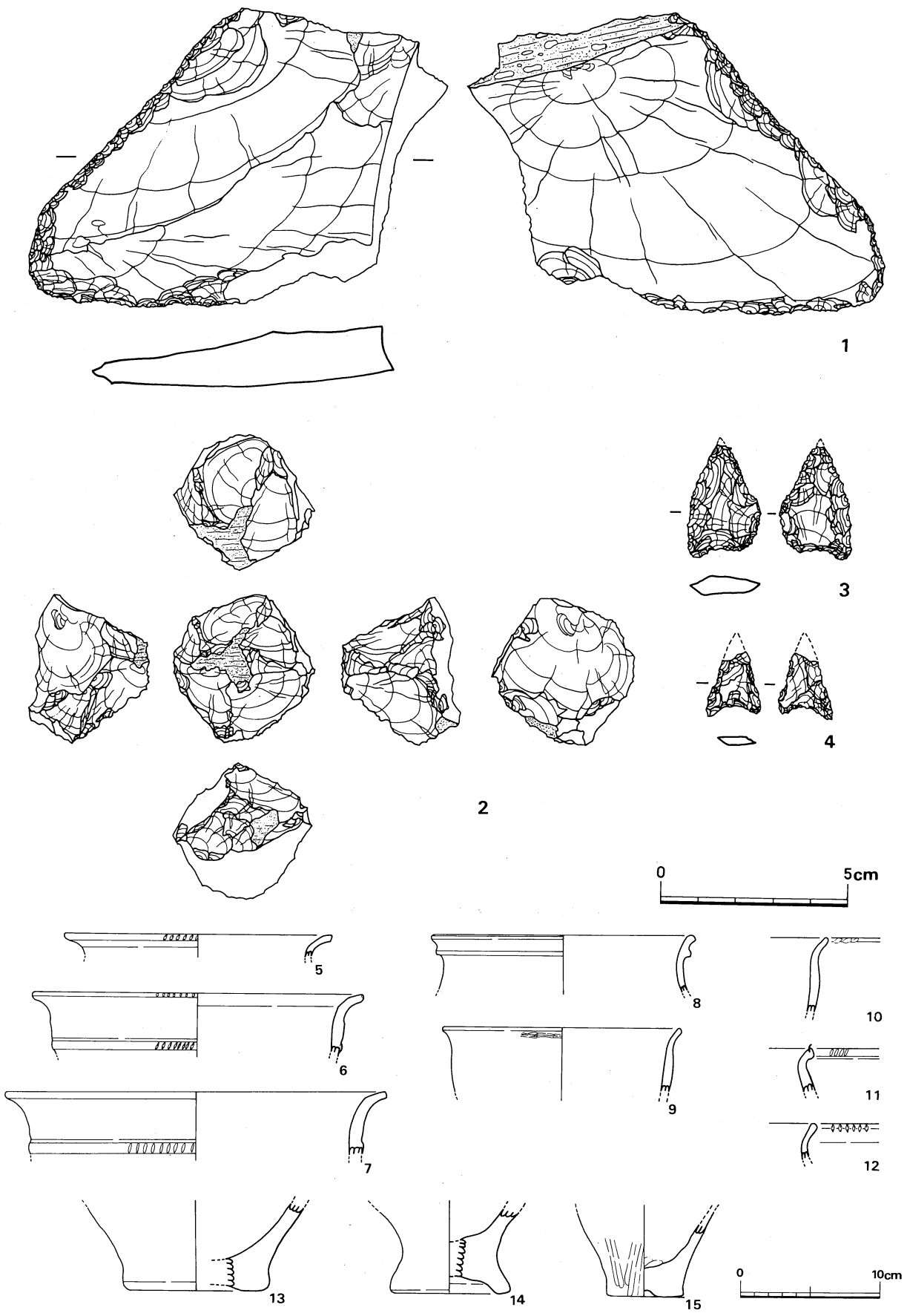
第39图 SXSa24 出土遺物実測図
