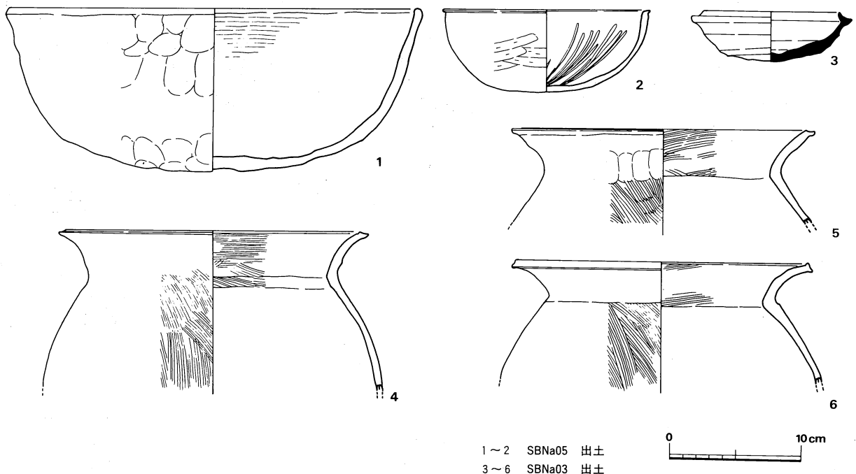
第23図 住居址出土遺物実測図(6)
