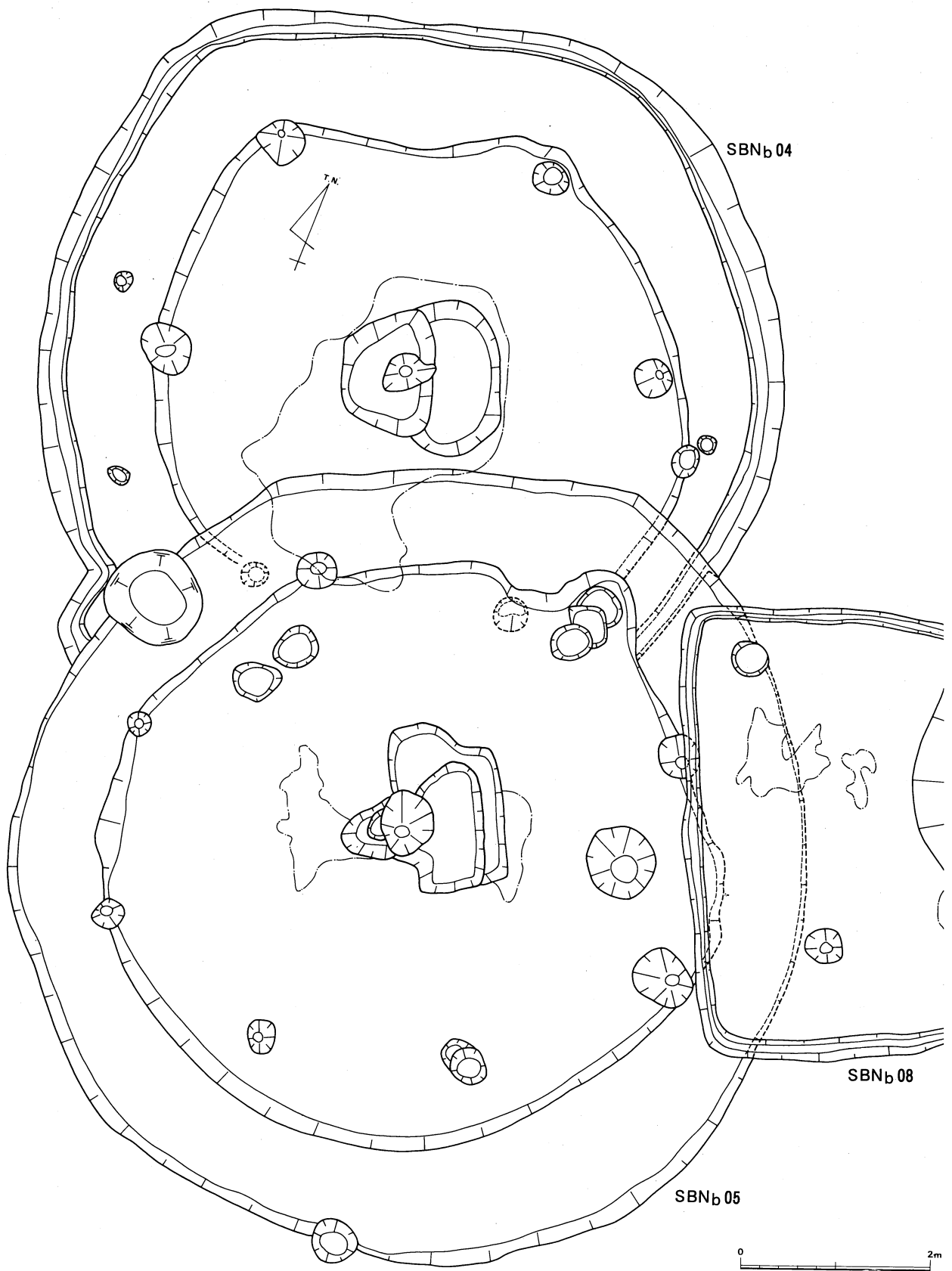
第 8 图 SBNb04·SBNb05·SBNb08 平面图
