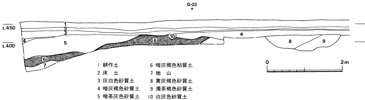
第38図 F・G-22 南壁土層図
