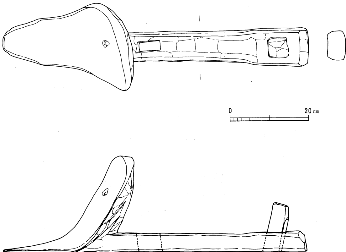
第47図 犁実測図
