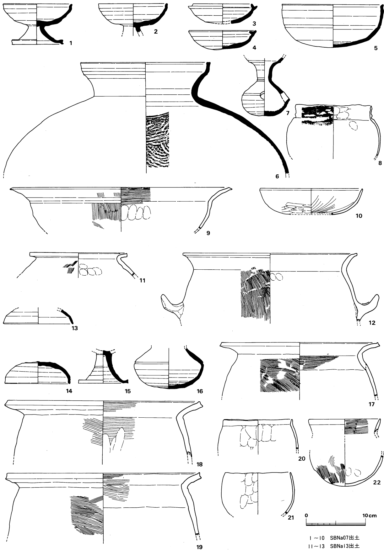
第22図 住居跡出土遺物実測図(5)
