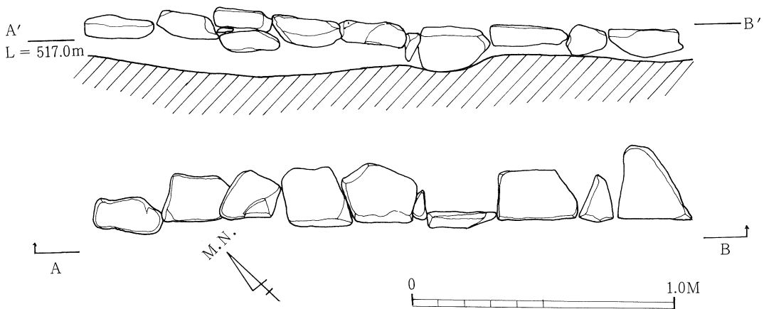
第12図 第2調査区石列実測図
