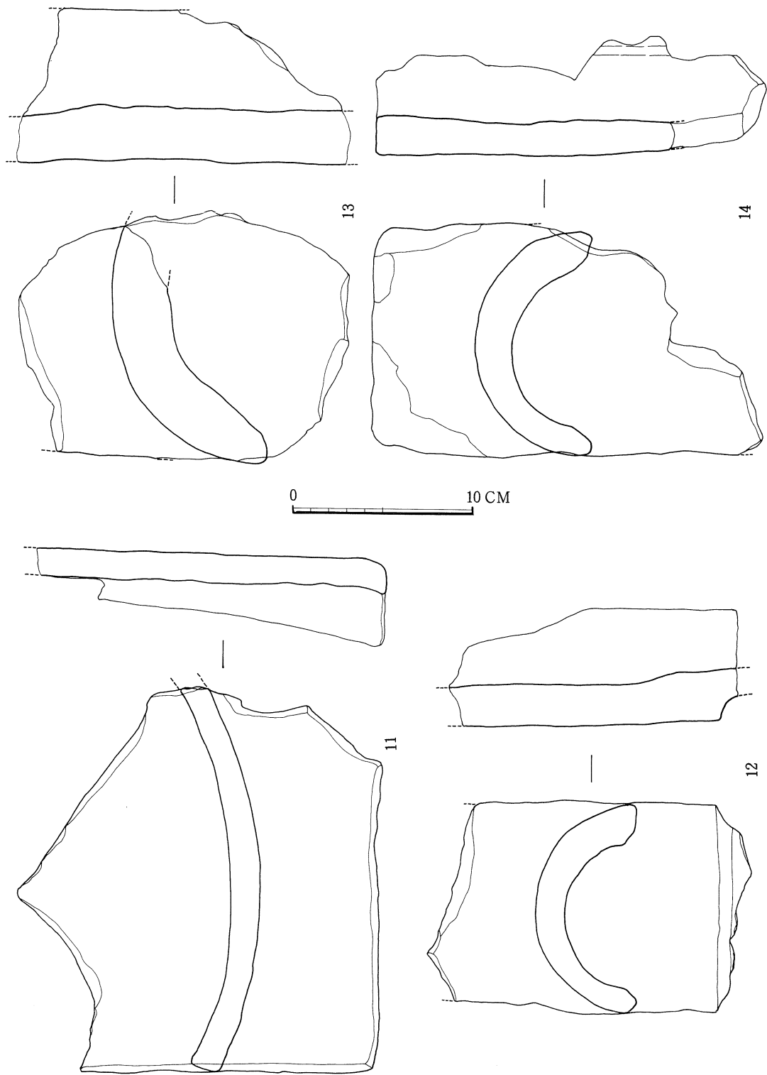
第21图 平瓦・丸瓦实测图
