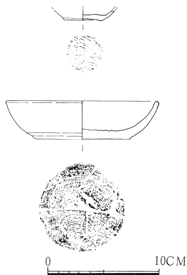
第23図 糸切り土器拓影・実測図
