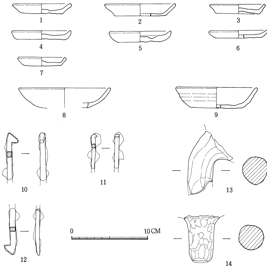
第13図 1区出土遺物実測図
