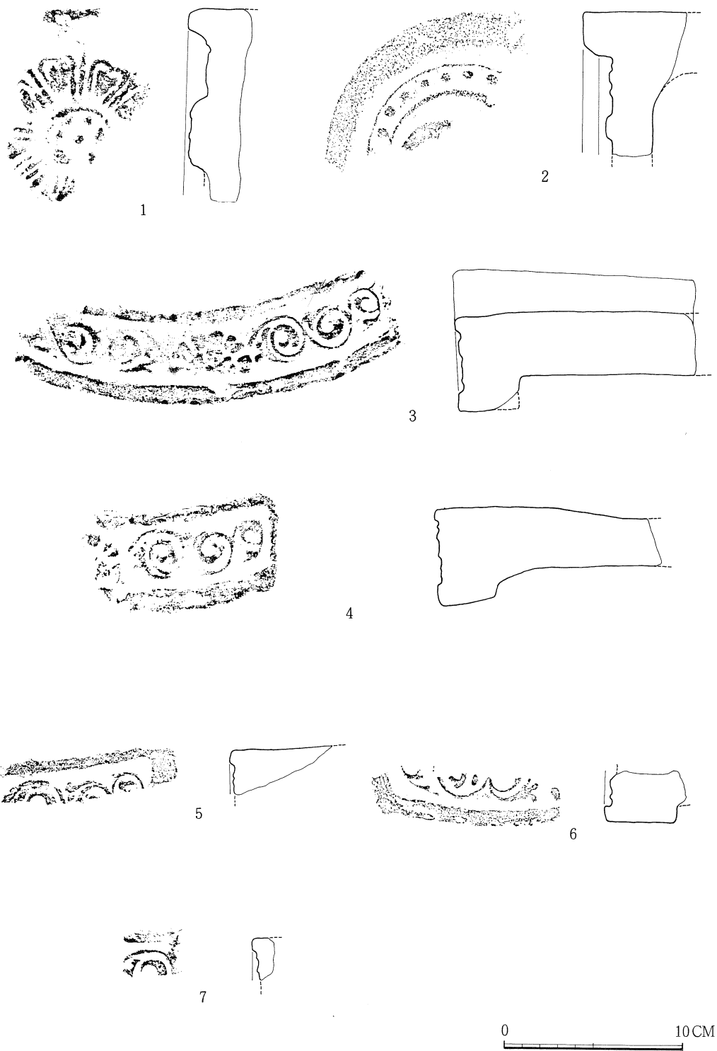
第19図 軒丸・軒平瓦拓影及実測図
