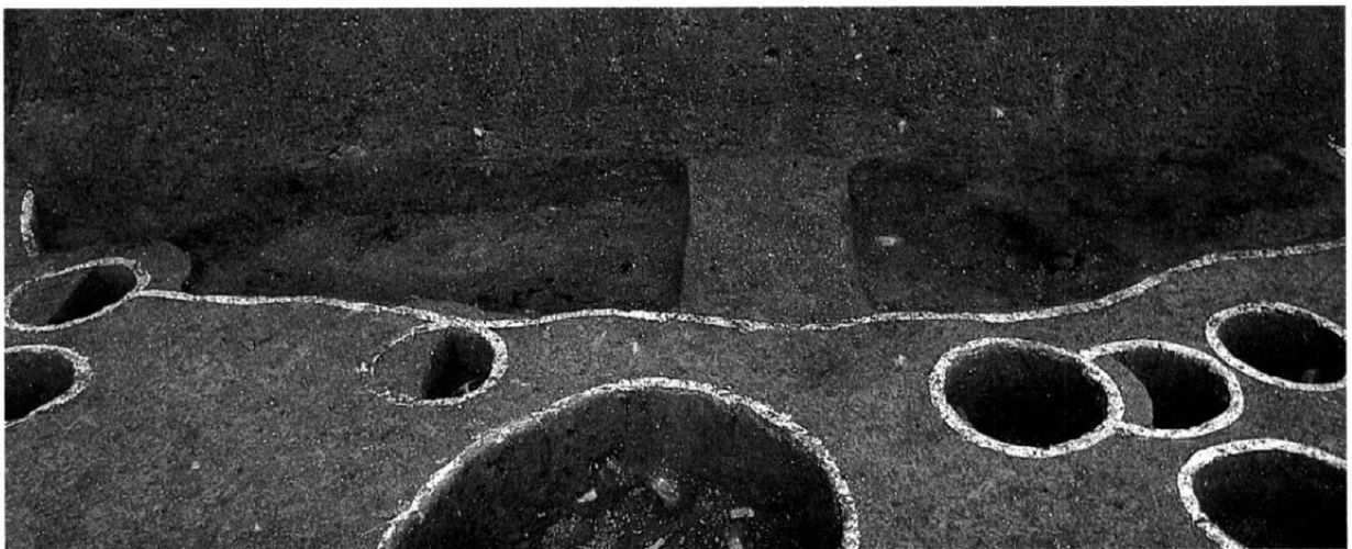
3. II区第2面SH02炭化材検出状況(東から)
