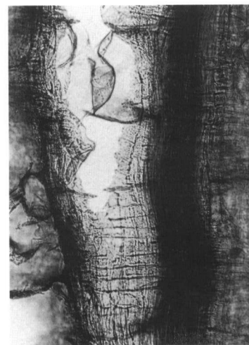
柱目 100倍
