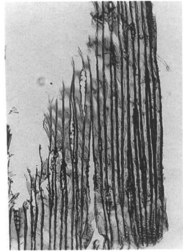
板目 50倍
