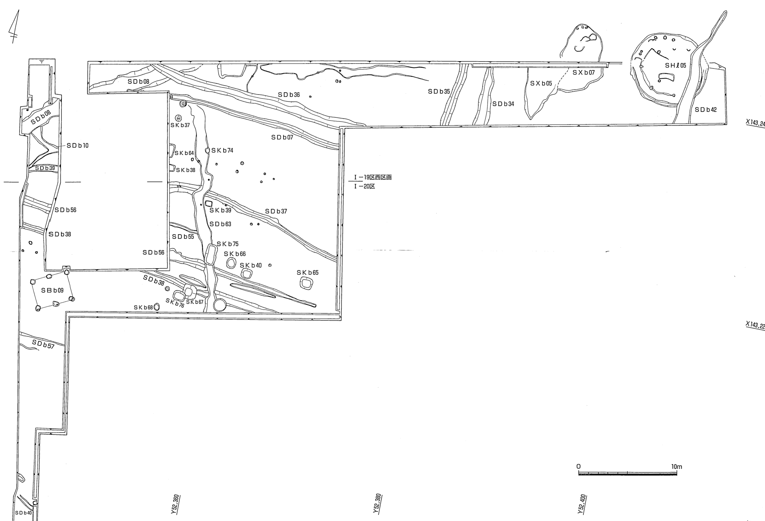
付图3 空港跡地遺跡B区 I-19区西区画・I-20区遺構図(1/200)
