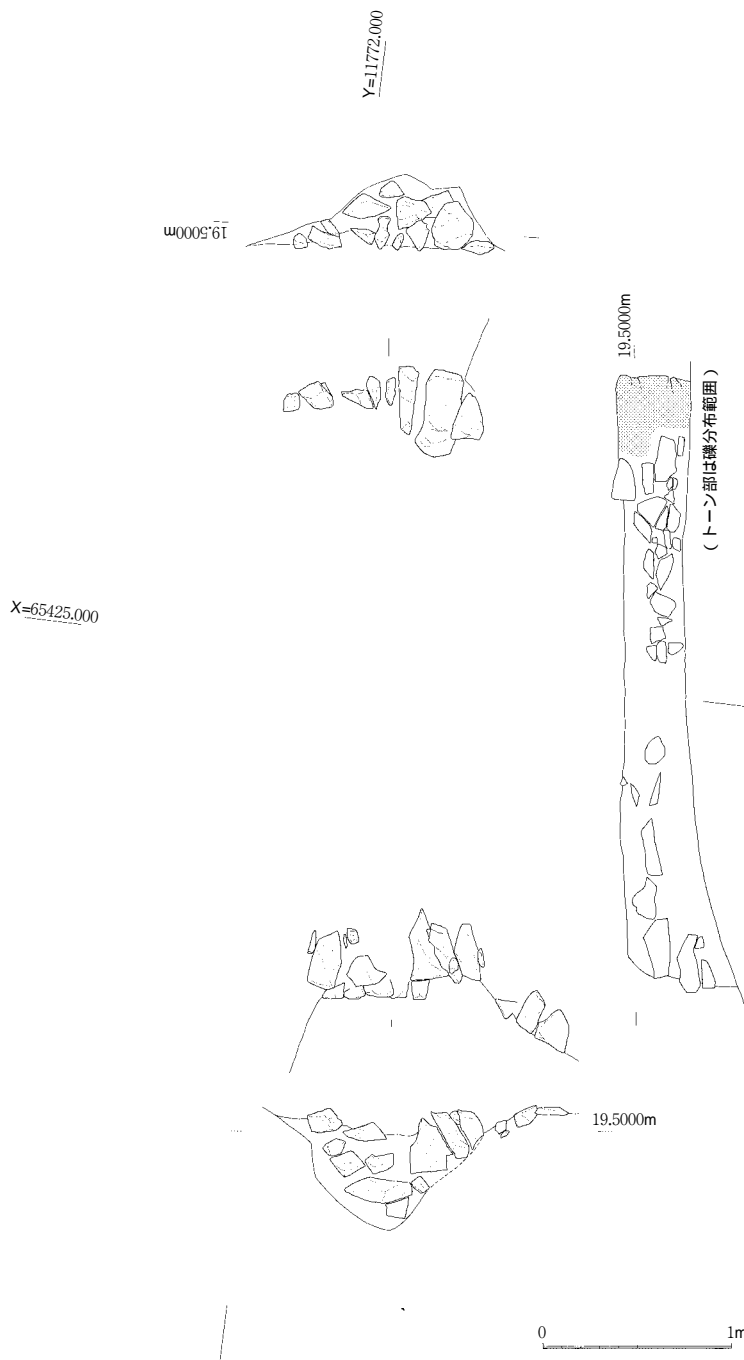
Fig.16 土橋 1 平面図・断面図
