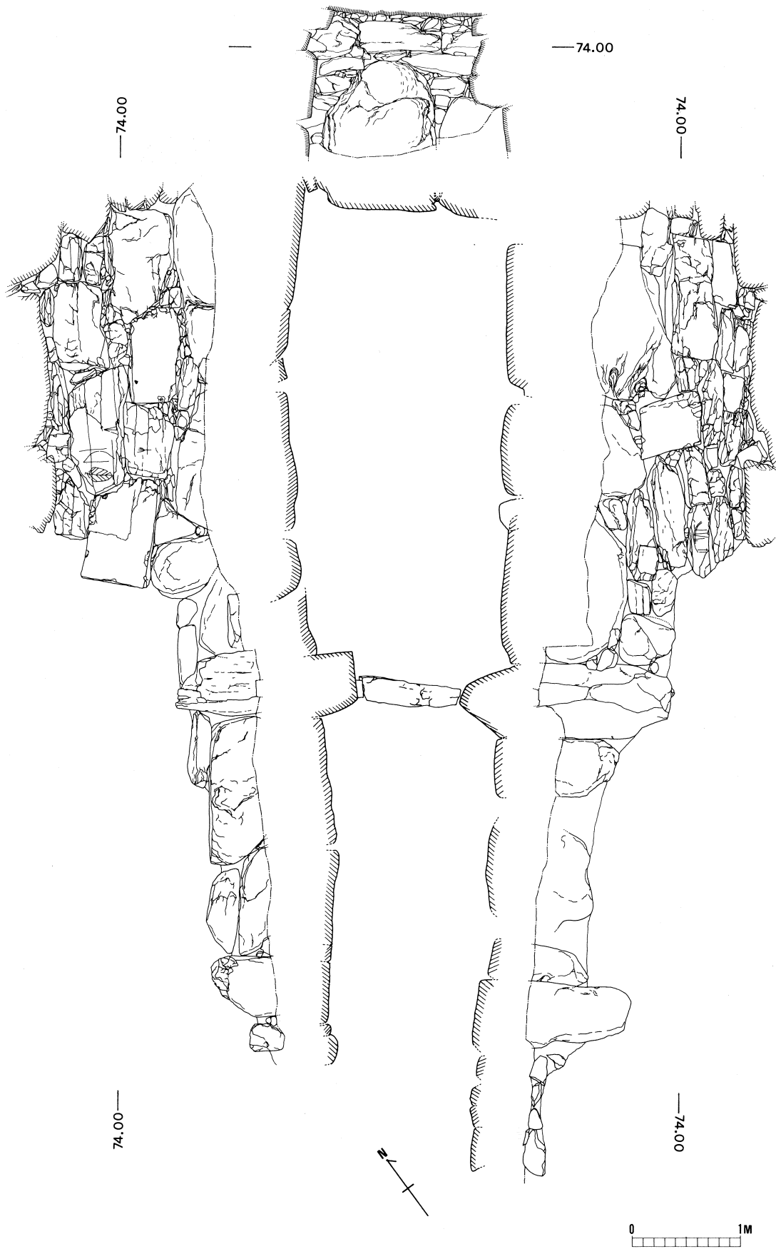
興昌寺山1号古墳石室実測図
