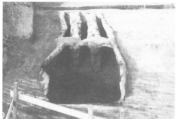
第4図 2号窯 (南から)
