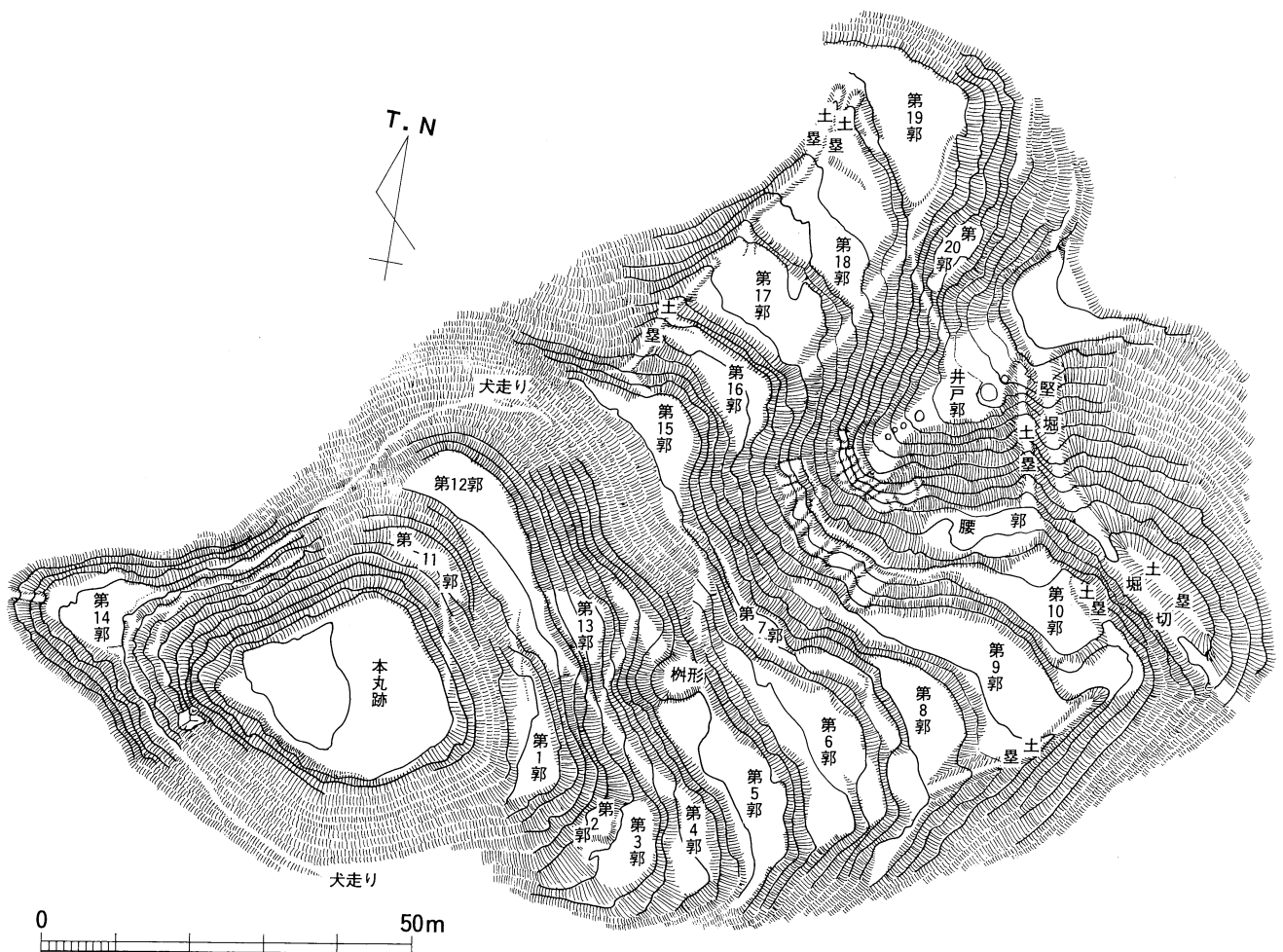
第2図 西長尾城跡測量図 (S = 1 : 1,000)
