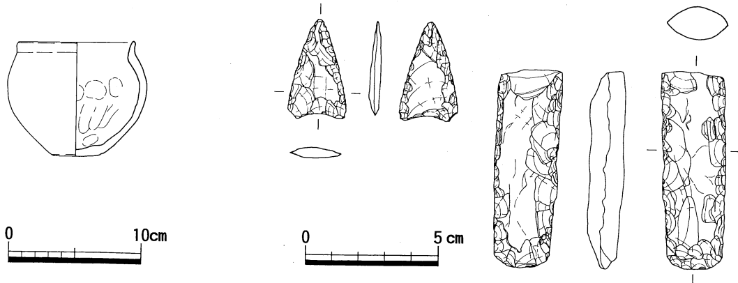
第5図 出土遺物実測図
