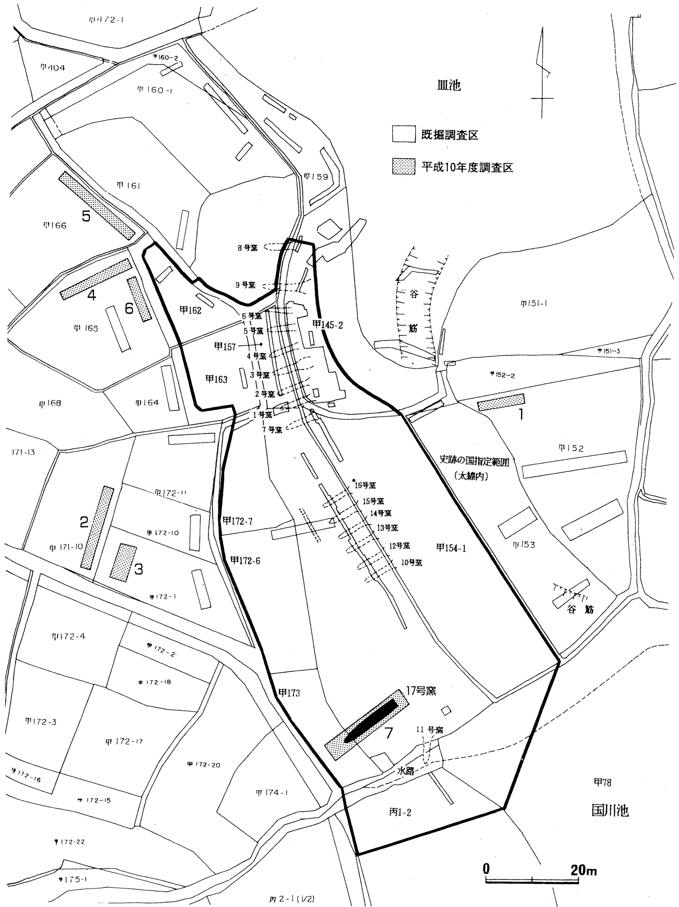
第4図 トレンチ配置図 (1 : 800)
