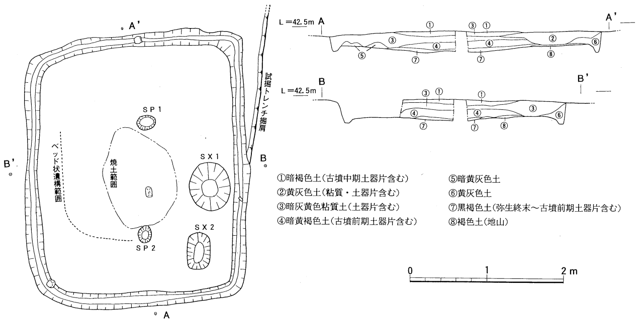
第4図 竪穴住居平面・土層実測図
