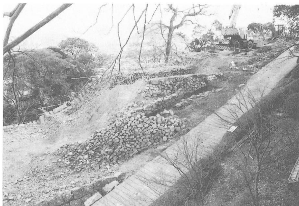
第2図 安山岩の石積み・腰巻石垣・グリハ積みの石積み（奥）
