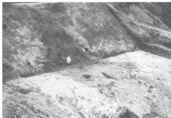
第3図 同煙道部～焼成部検出状況
