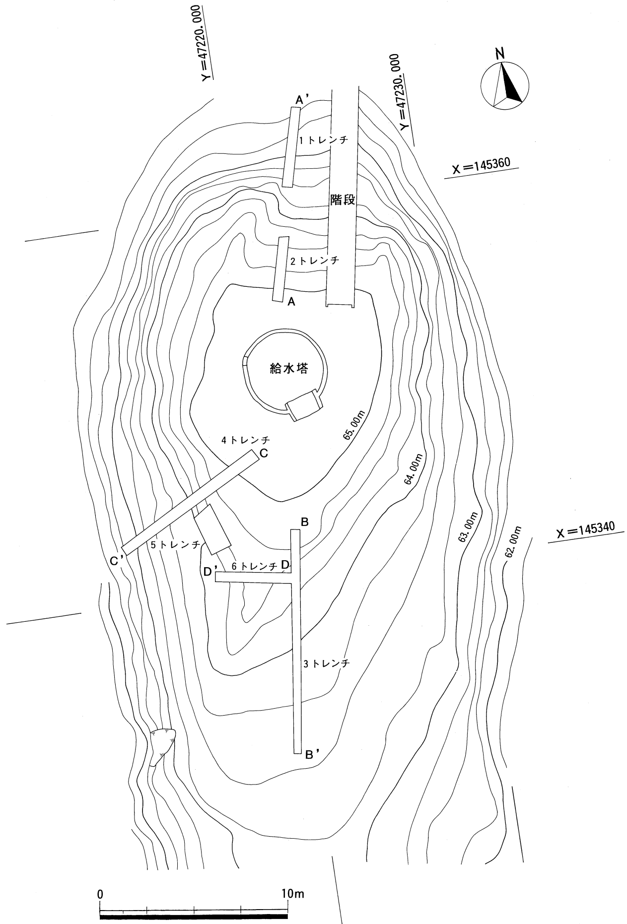
第3図 亀塚墳丘測量図
