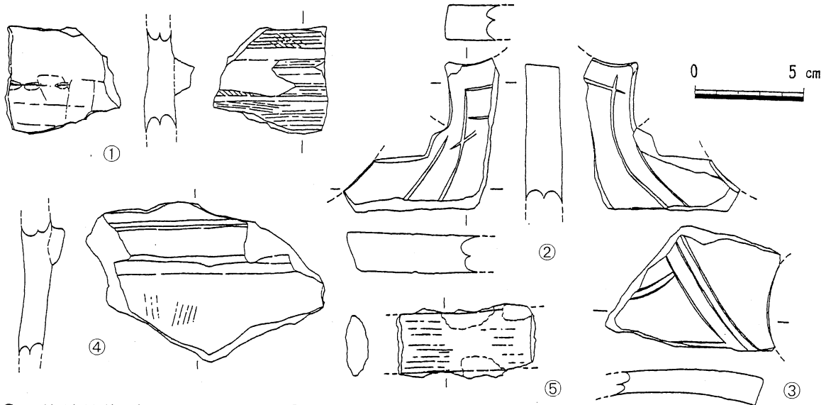
第4図 出土遺物実測図
