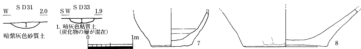
第7図 SD31・33断面 (1/50) 及び出土遺物 (1/4)
