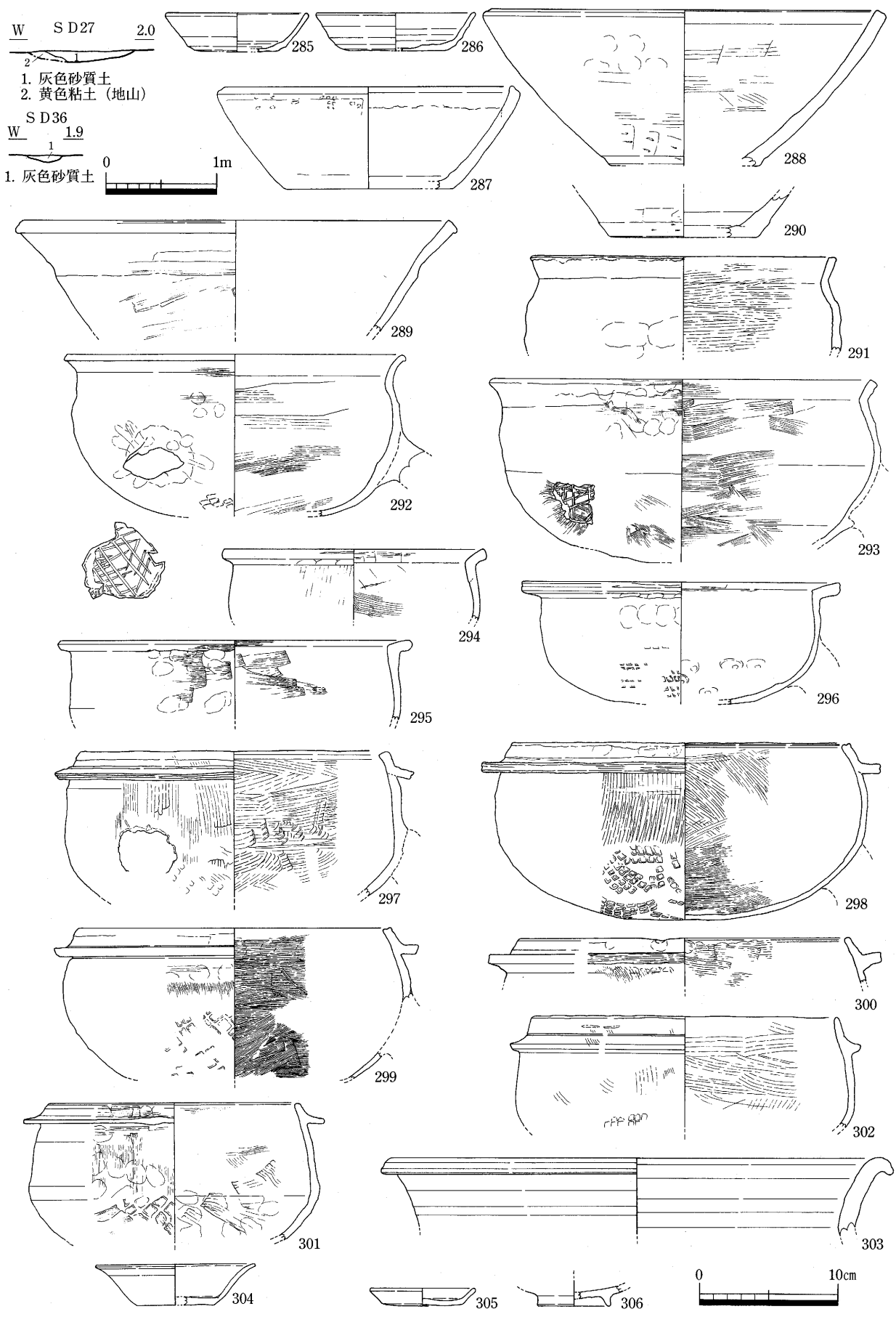
第25図 S D 27 · 36 断面 (1/50) 及び S D 29 · 32 出土遺物 (1/4)
