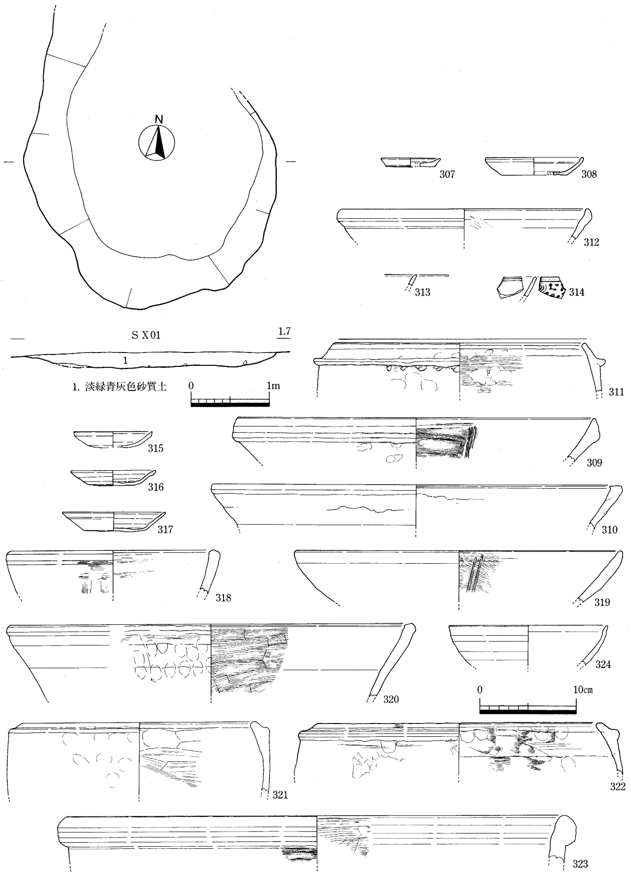
第28図 SX01平・断面 (1/50) 及びSX01・03出土遺物 (1/4)
