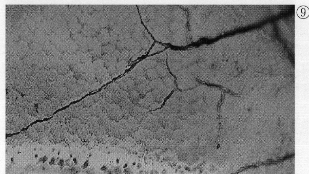
第150図 椀形鍛冶滓の顕微鏡組織
