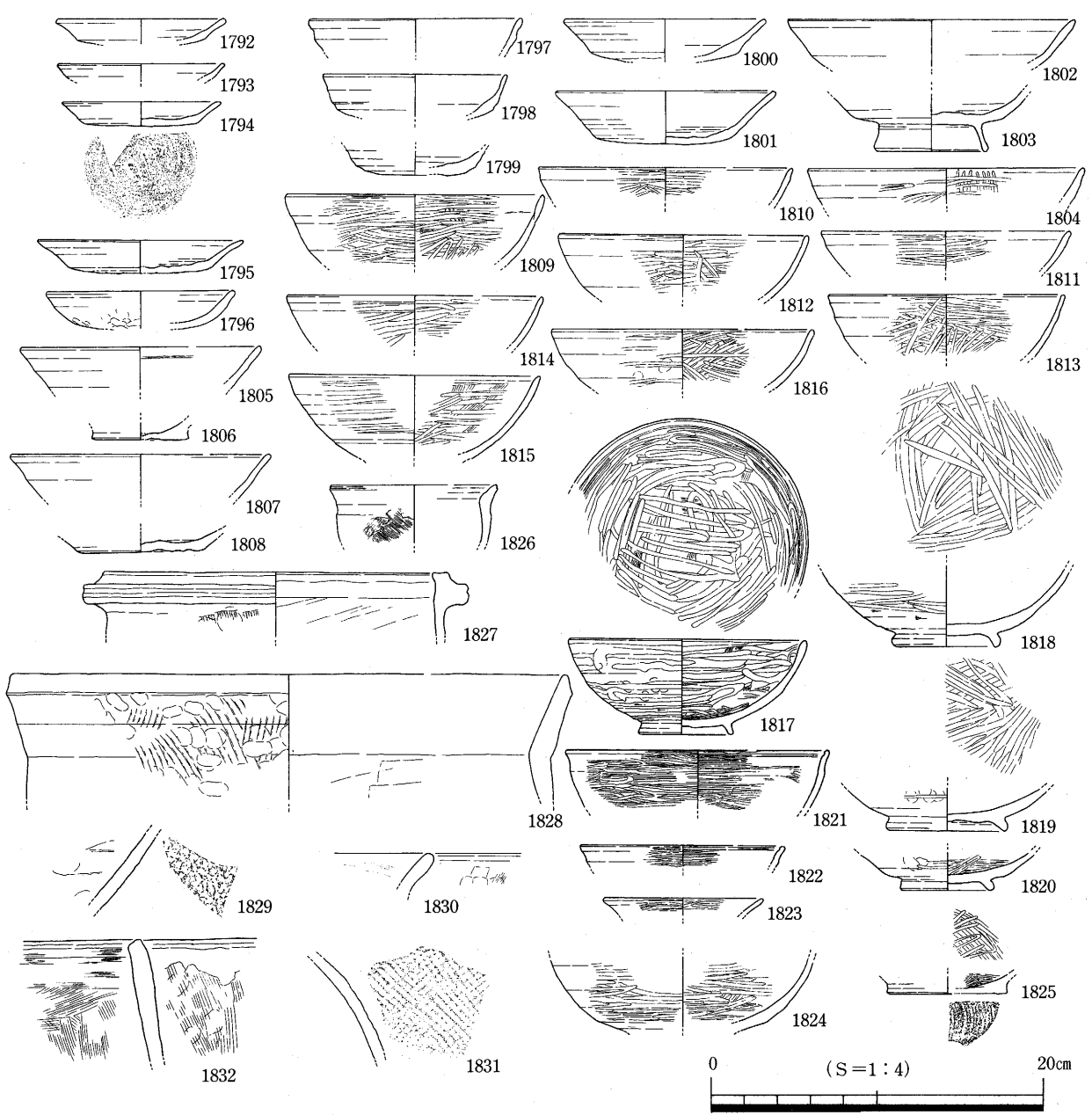
第94図 SK01平・断面 SD08出土遺物
