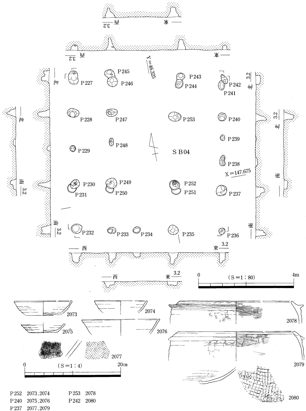
第106図 SB04 平・断面及び出土遺物
