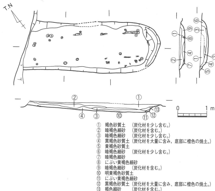
第50図 SX03平・断面図(1/80)
