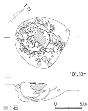
第47図 ST02平・断面図（1/40）
