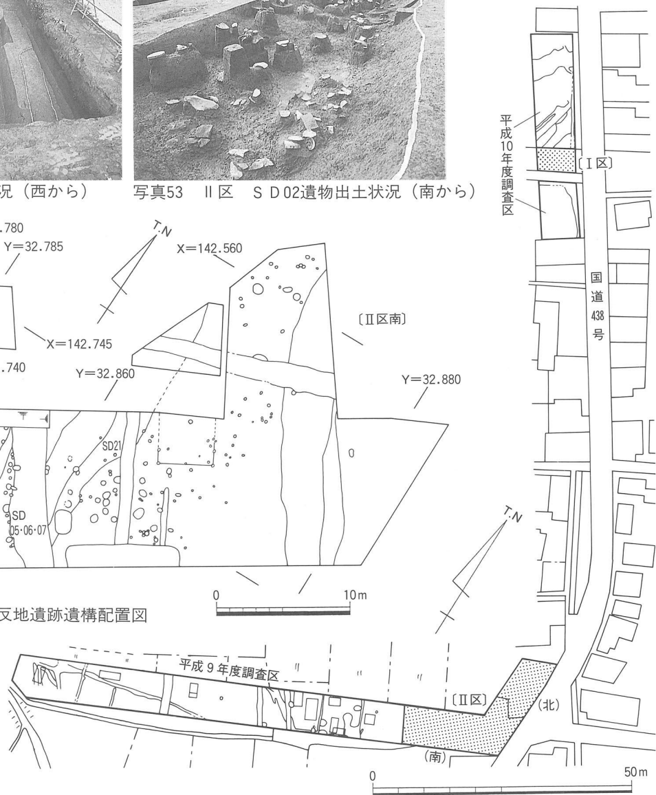
第44図 川津六反地遺跡調査区割図
