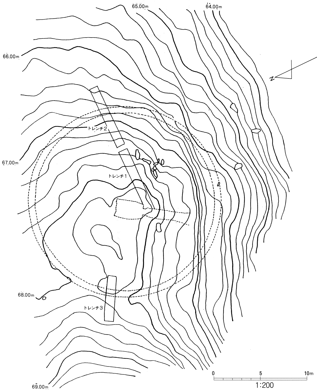
久米塚古墳地形測量図・トレンチ配置図 (石室と墳丘推定範囲は点線で示した。)
