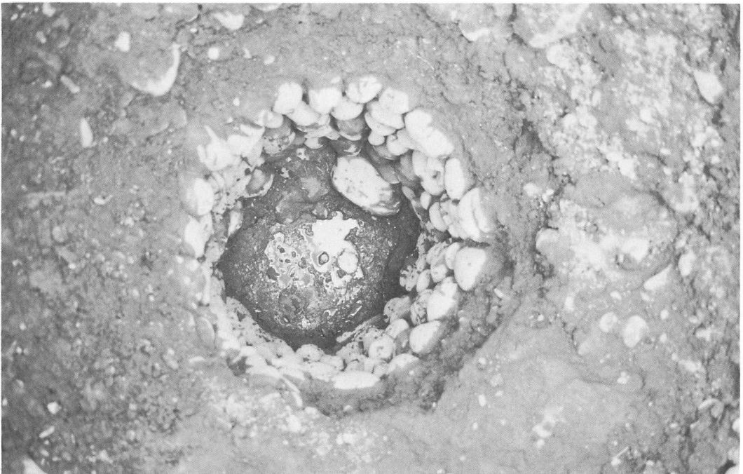
SEI (東より)
