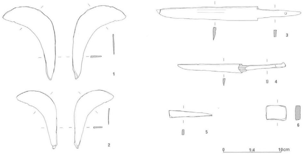
第11図 H2号住居址出土遺物実測図(鉄製品)
