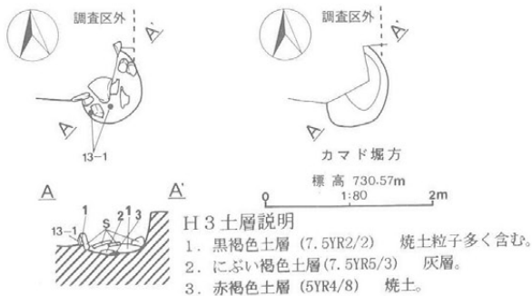
第12図 H3号住居址実測図
