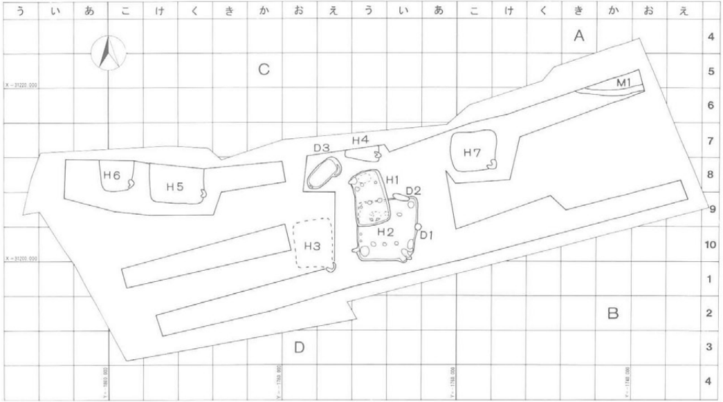
第15図 下穴虫遺跡Ⅰ全体図 (1 : 600)
