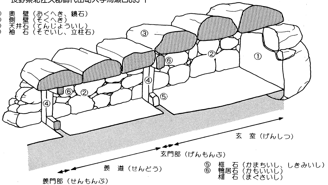
横穴式石室模式図
