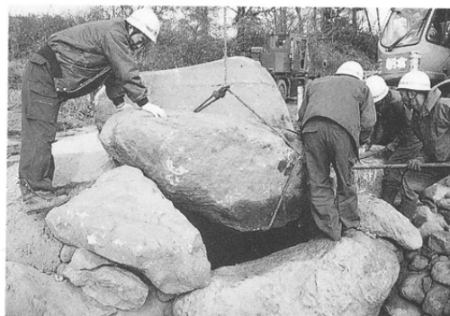
写33 微調整
