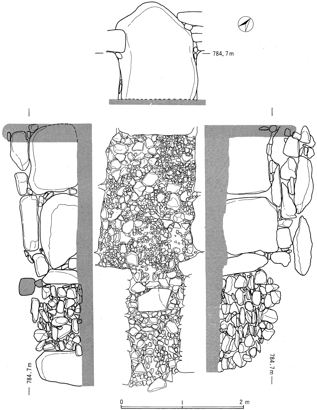
第4図 I号墳石室展開図 (1 : 60)
