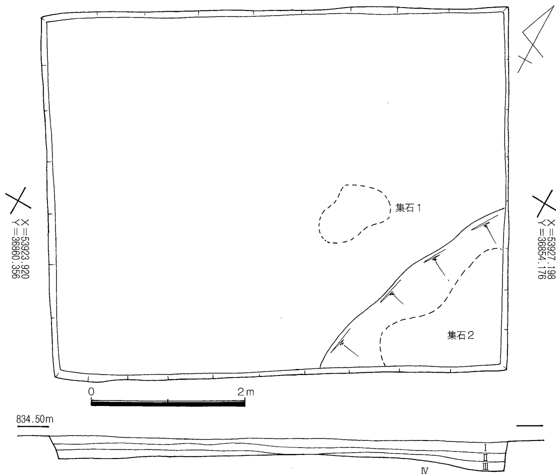
第3図 全体図と土層断面図（1：50）
