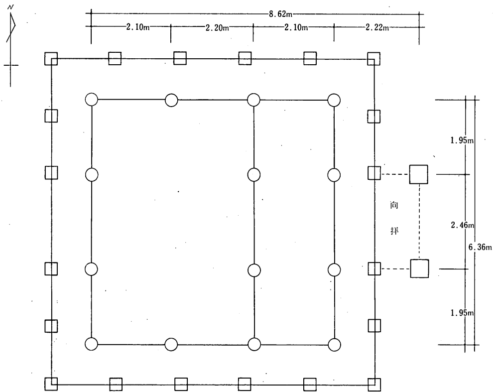
平面图
