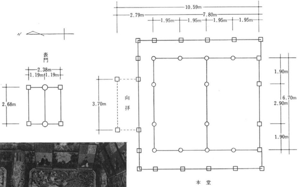
本堂 平面図
