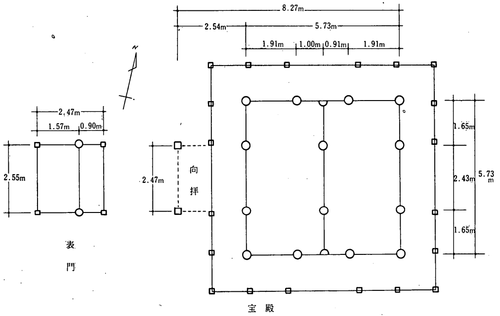
平面图
