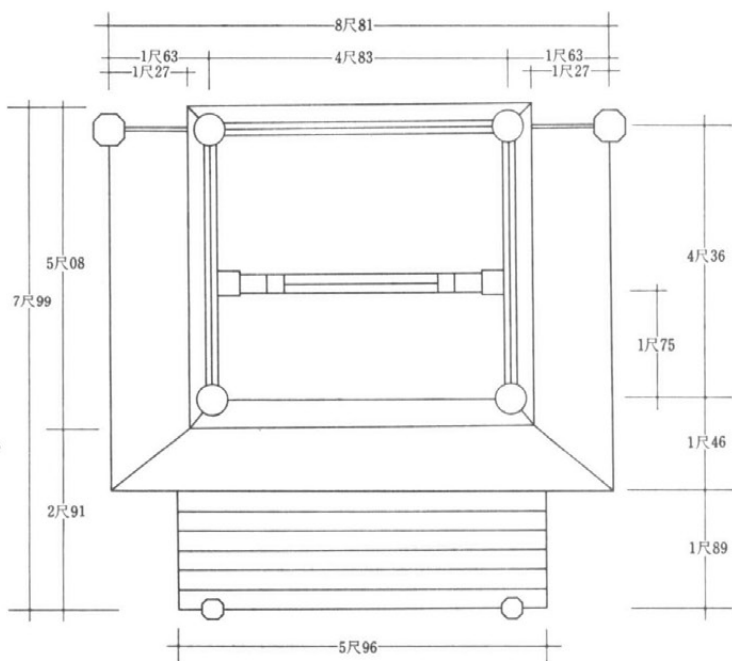
平面图
