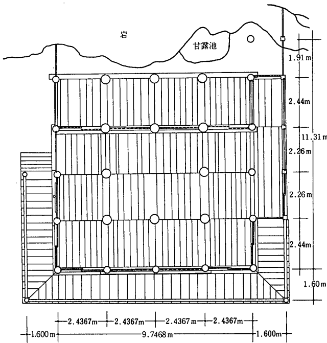
復元修理後平面図
