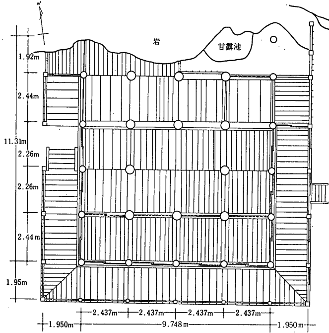
修理前平面図
