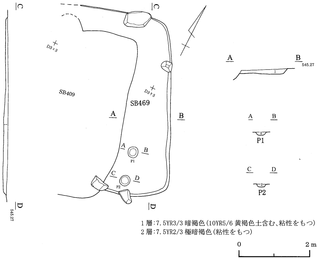
第222図 469号住居跡
