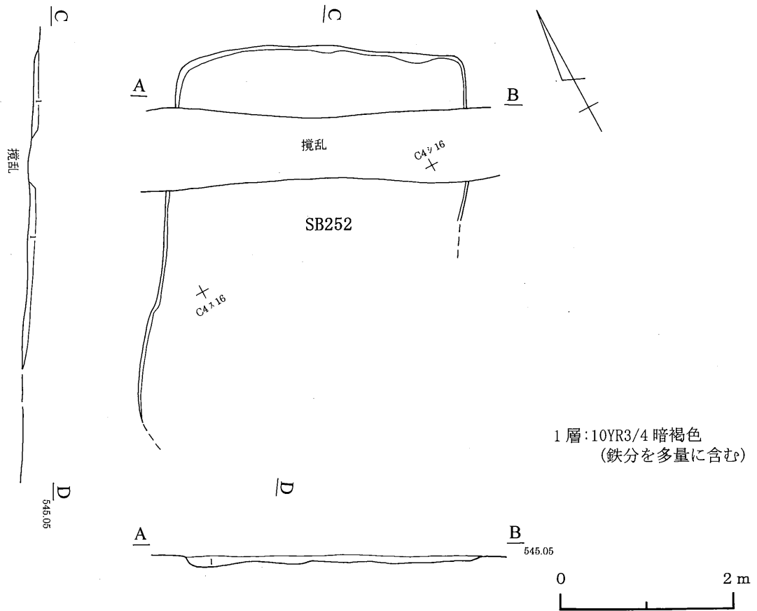
第17図 252号住居跡
