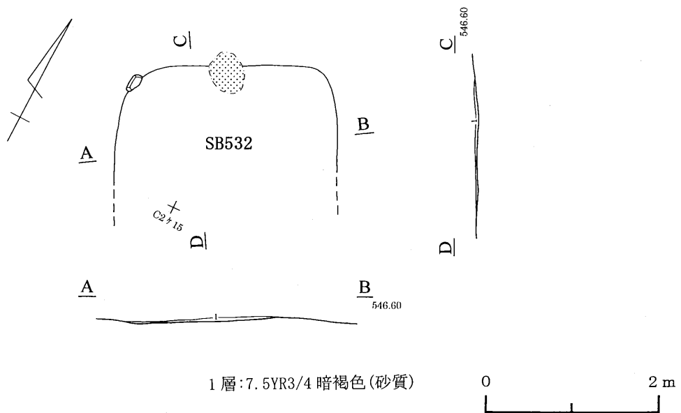
第232図 532号住居跡
