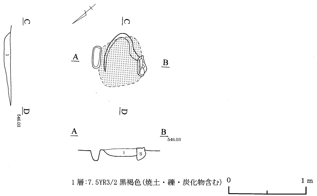
第221図 423号住居跡
