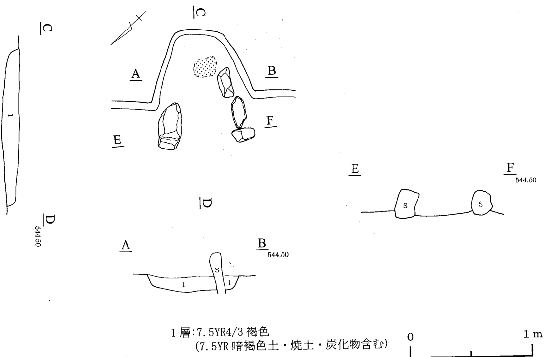
第34図 312号住居跡
