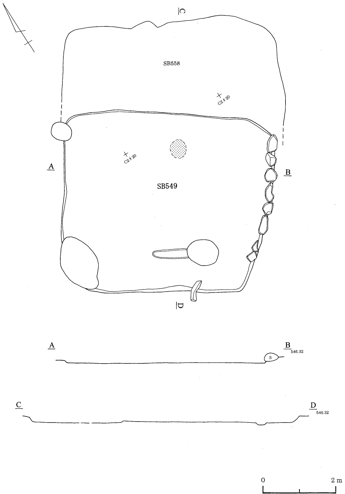
第124図 549号住居跡
