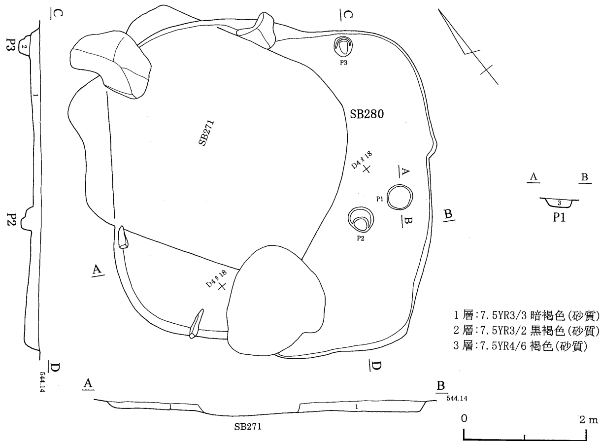
第190図 280号住居跡
