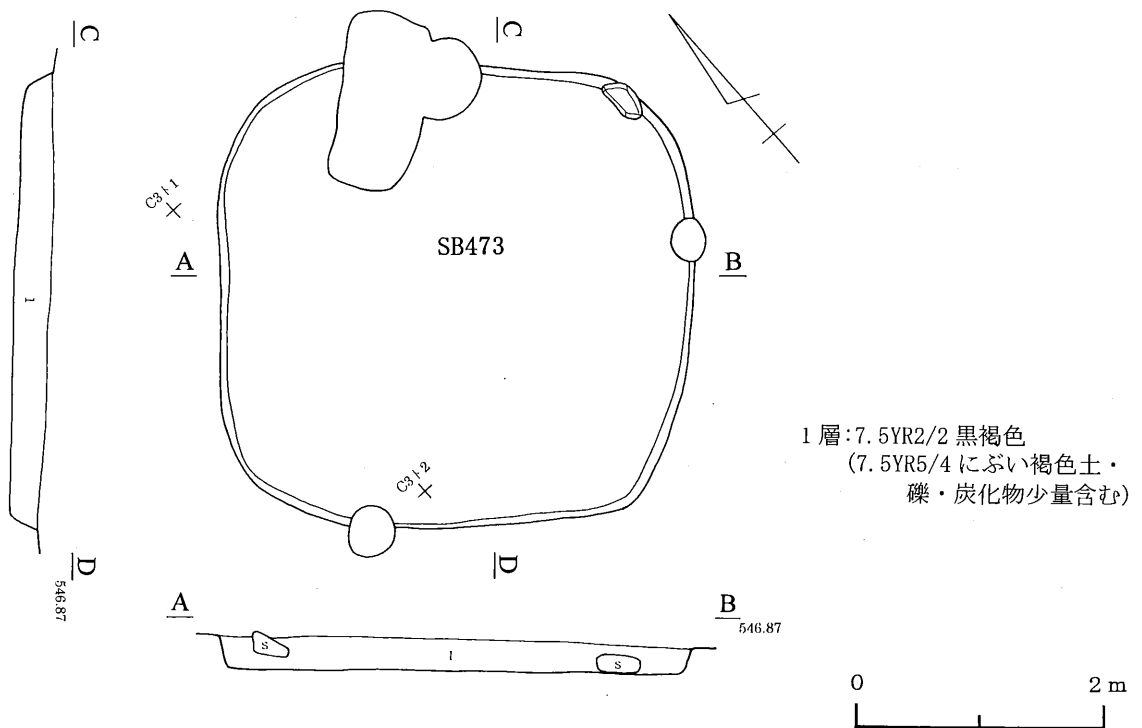
第223図 473号住居跡
