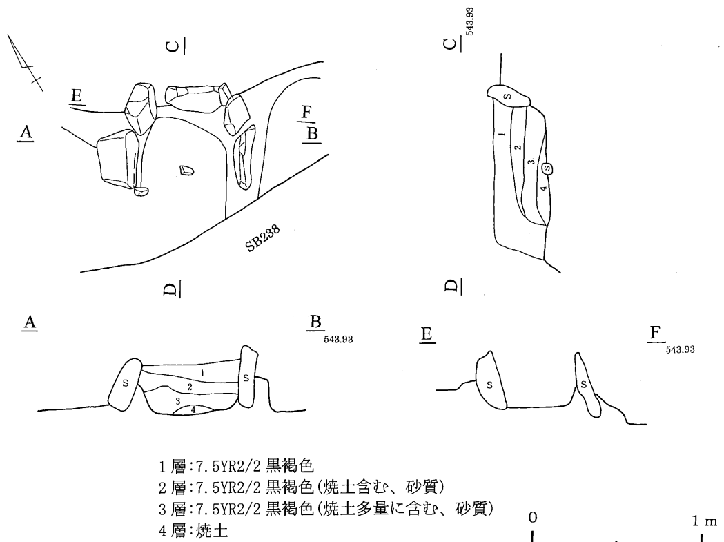
第11図 237号住居跡
