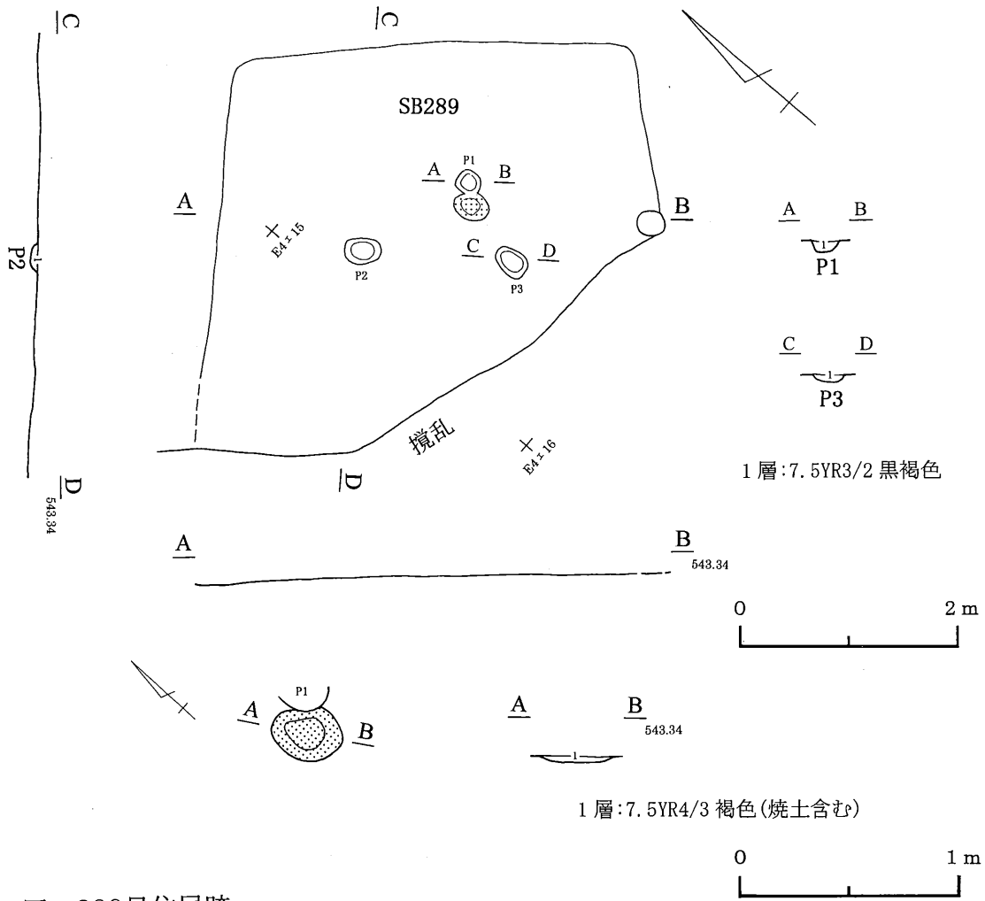
第194図 289号住居跡
