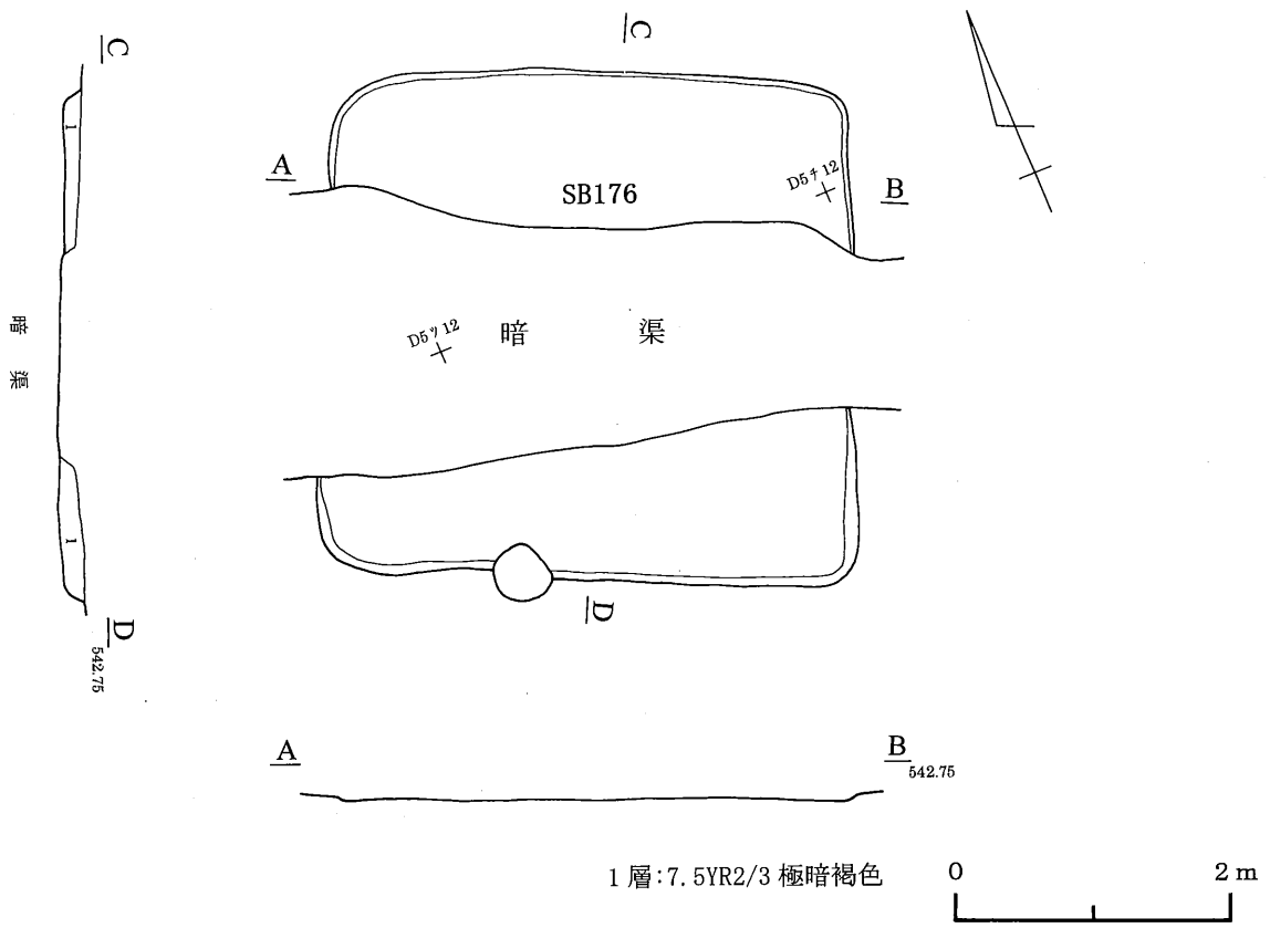
第171図 176号住居跡
