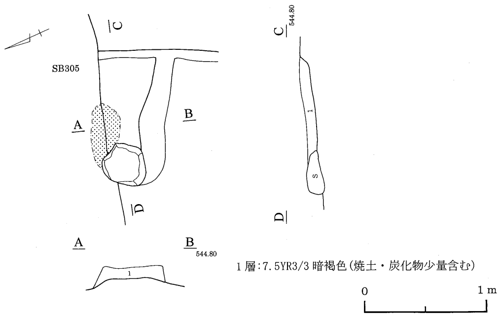
第35図 316号住居跡
