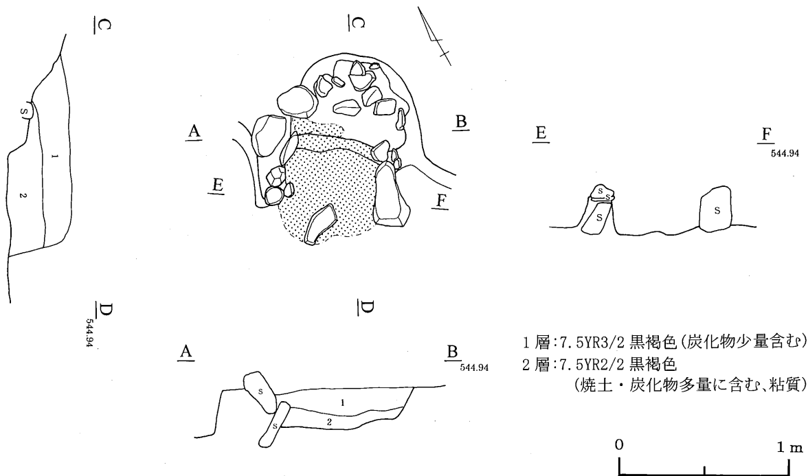
第45図 341号住居跡
