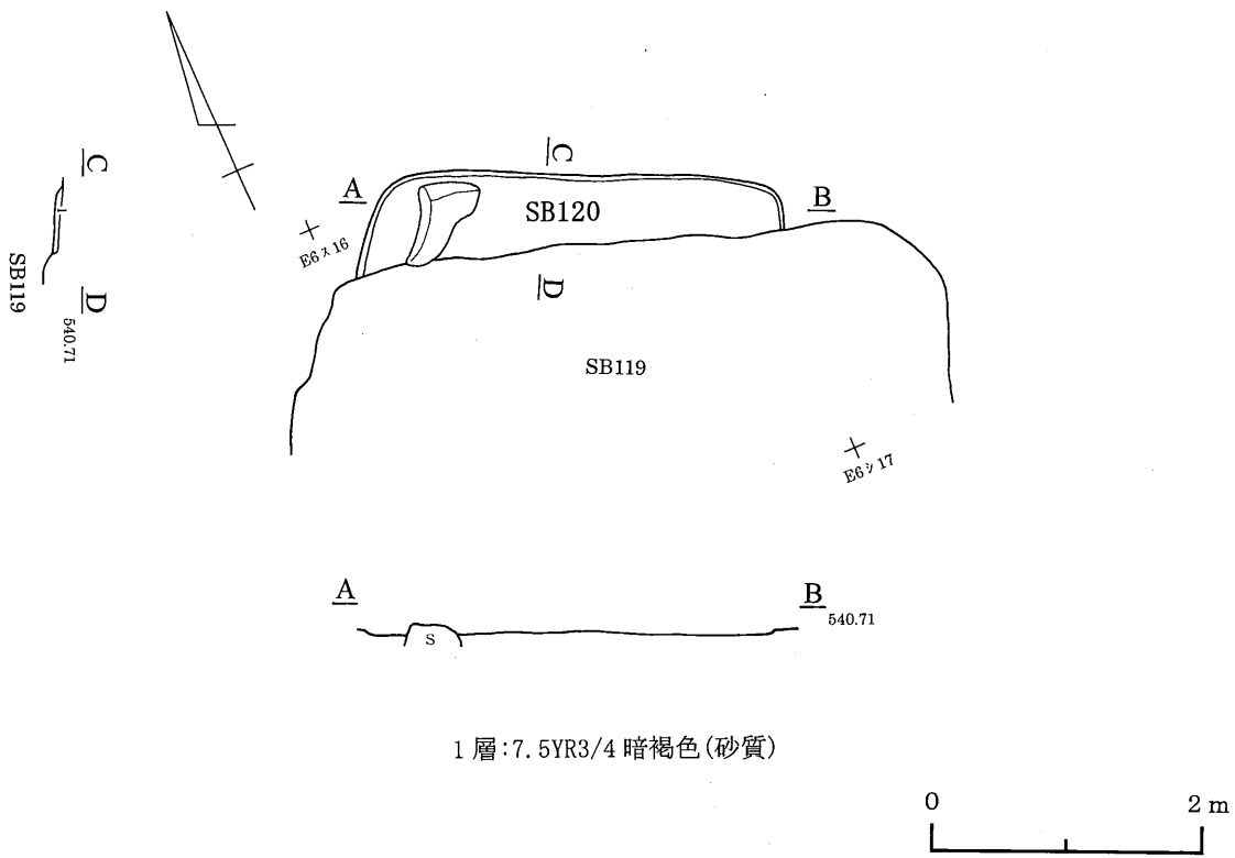
第158図 120号住居跡
