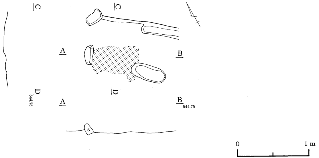
第43図 340号住居跡② (カマド)
