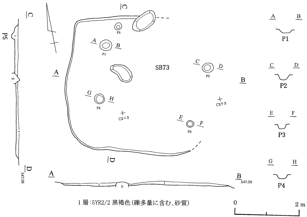
第145図 73号住居跡
