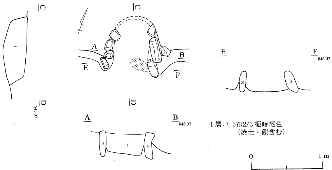
第72図 409号住居跡
