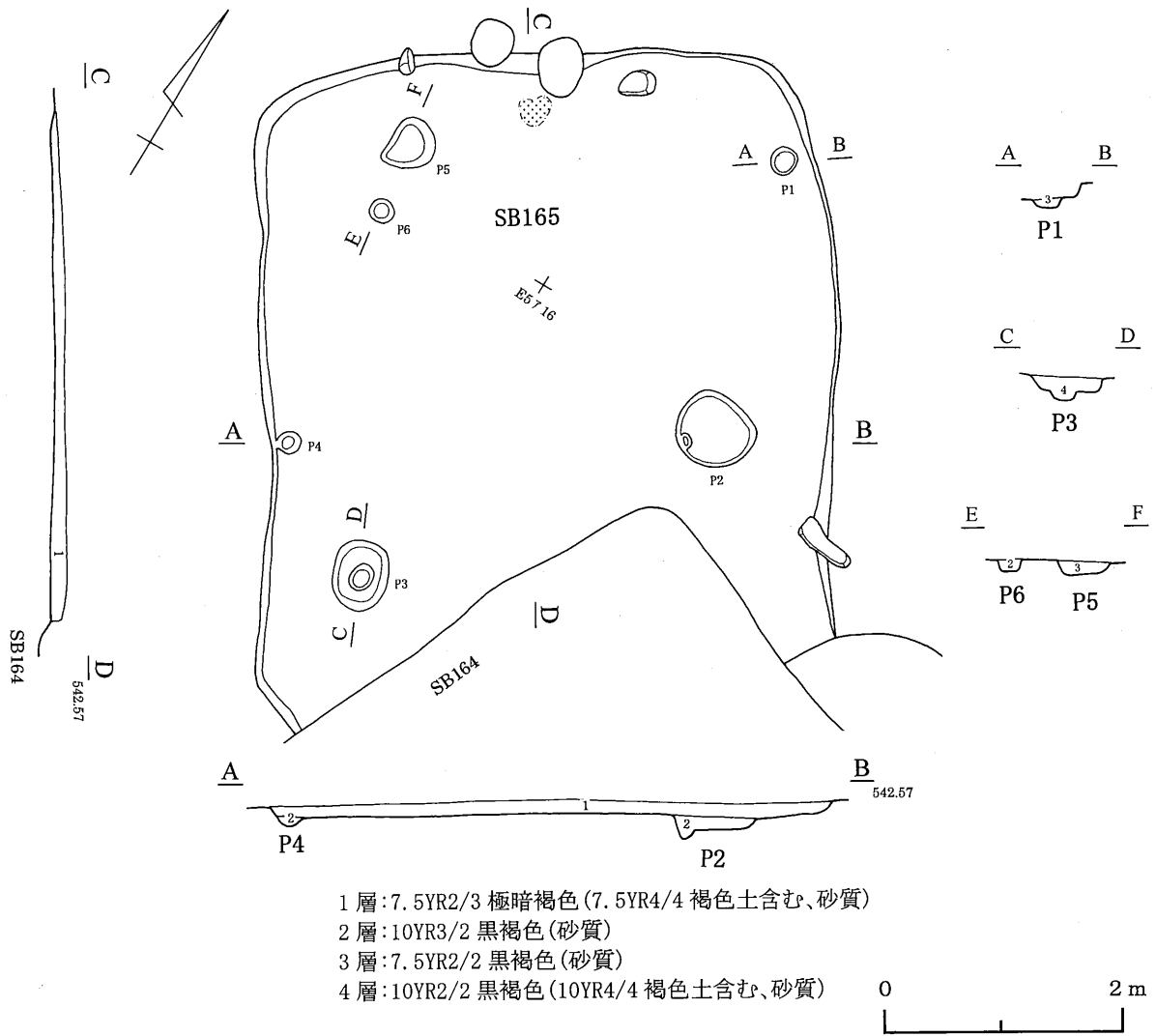
第166図 165号住居跡
