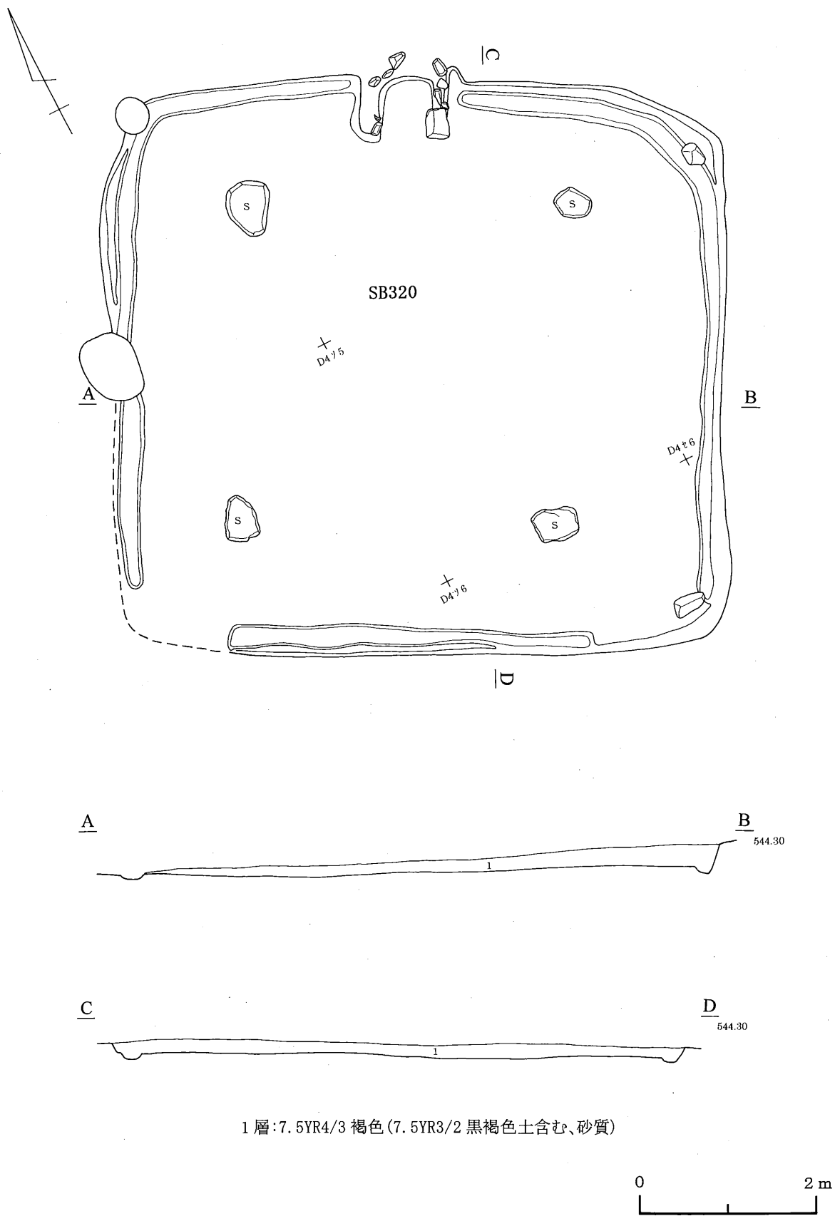
第37図 320号住居跡①
