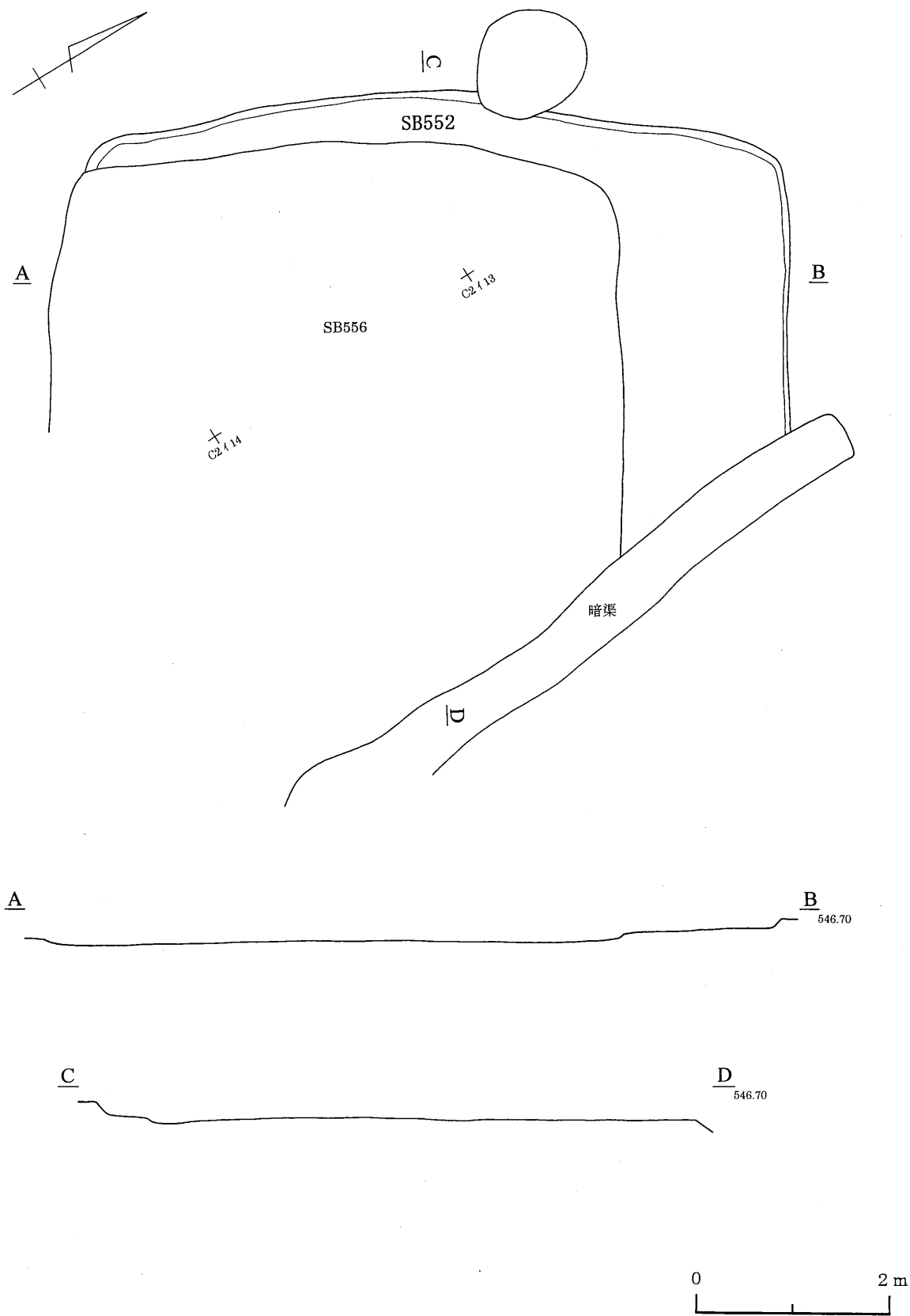
第125図 552号住居跡
