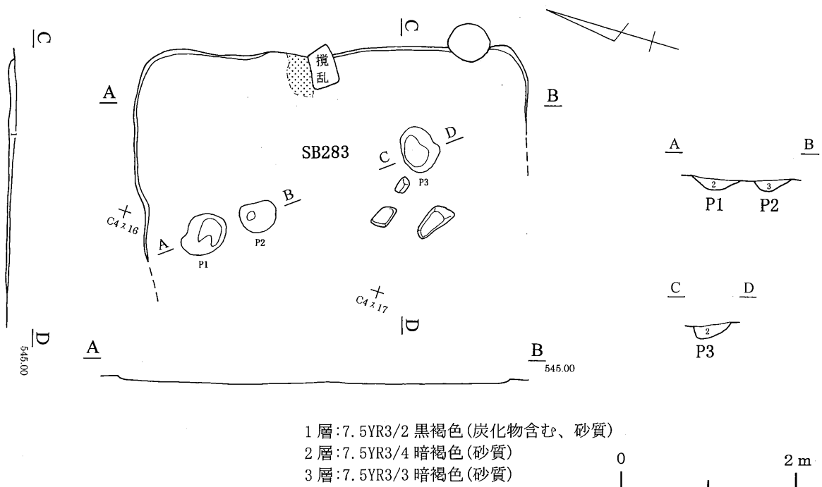
第24図 283号住居跡
