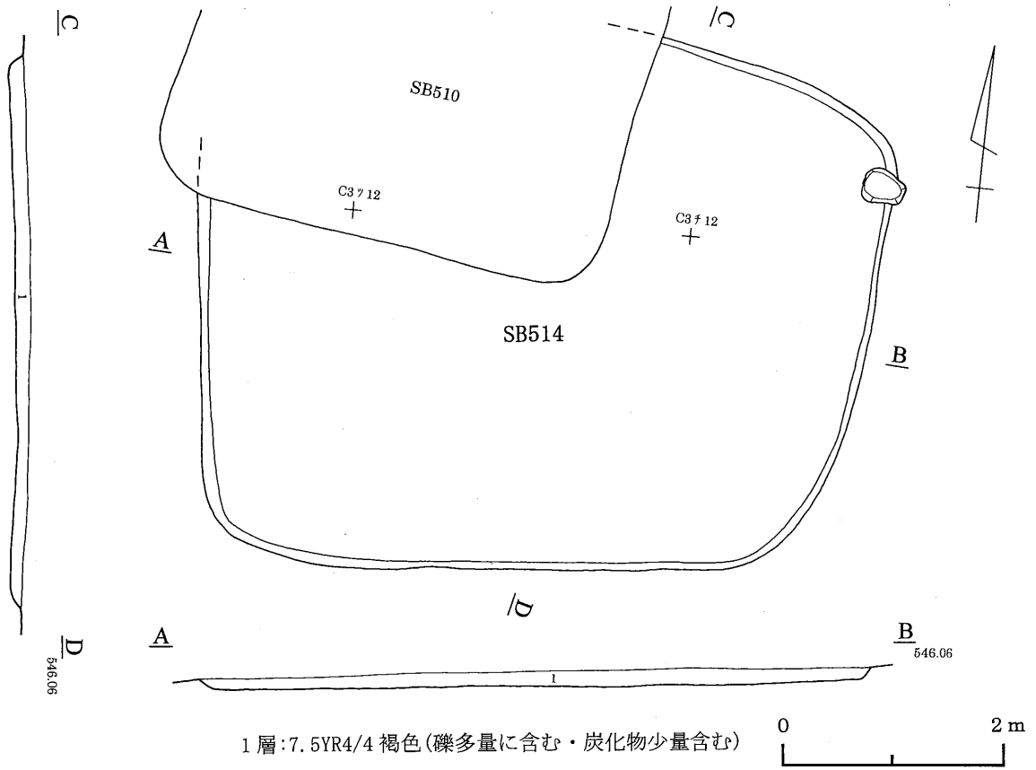
第116図 514号住居跡
