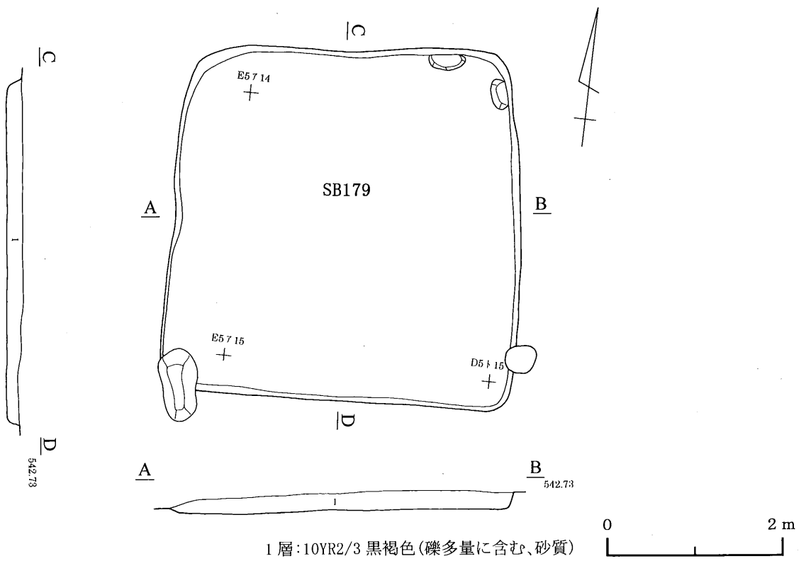
第174図 179号住居跡
