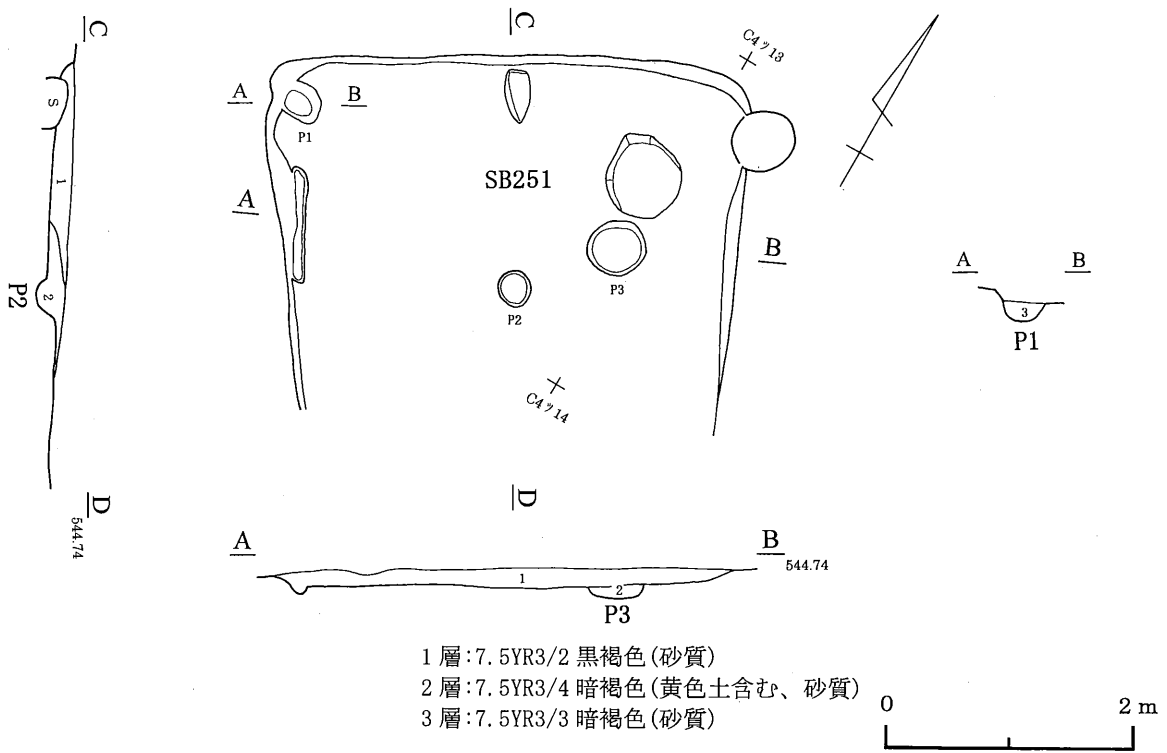
第16図 251号住居跡
