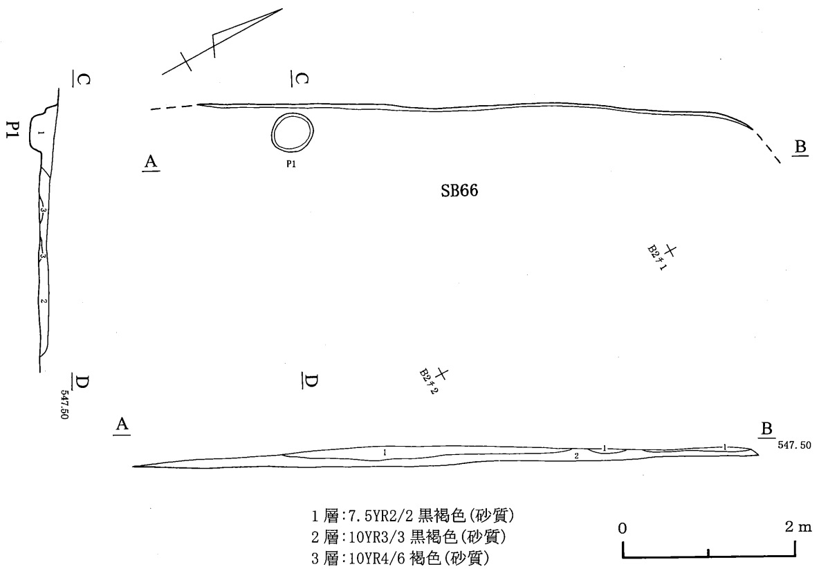
第142図 66号住居跡
