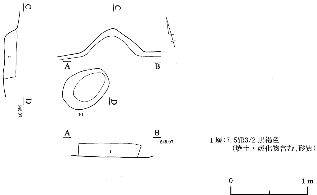
第224図 474号住居跡
