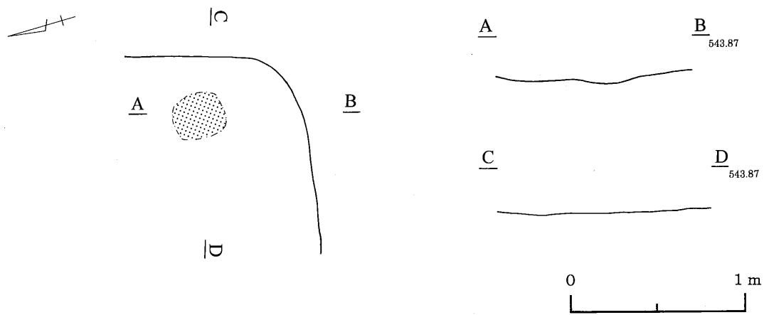
第27図 294号住居跡
