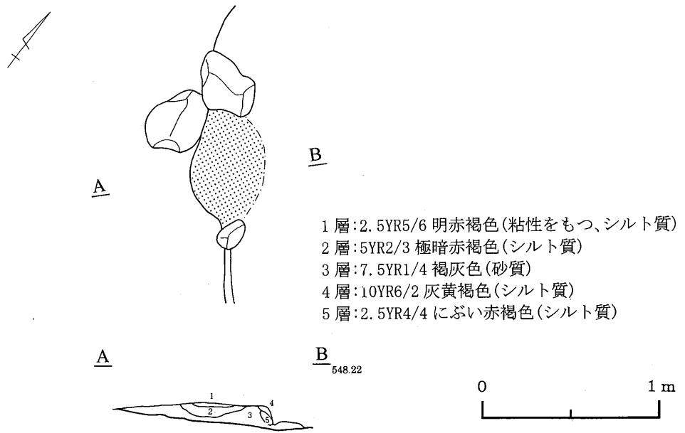
第129図 13号住居跡② (カマド)
