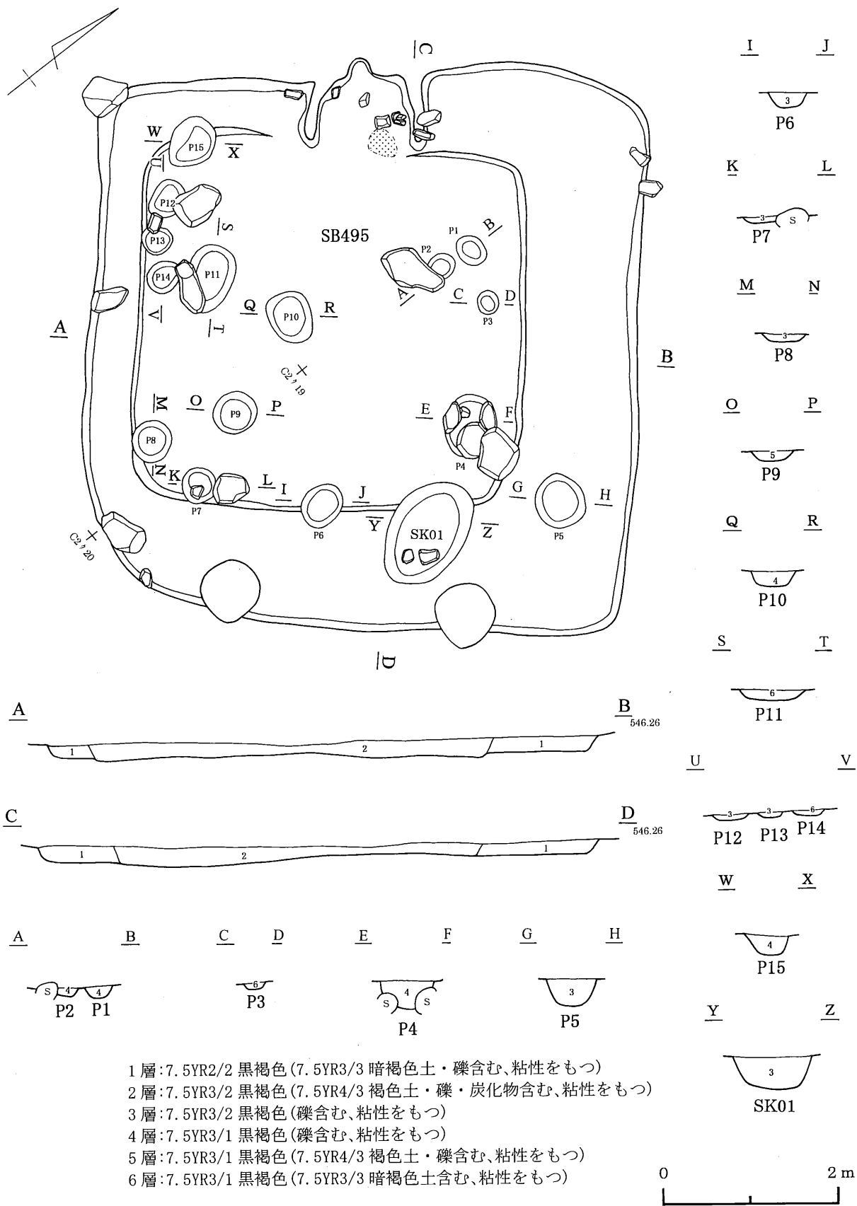
第103図 495号住居跡①
