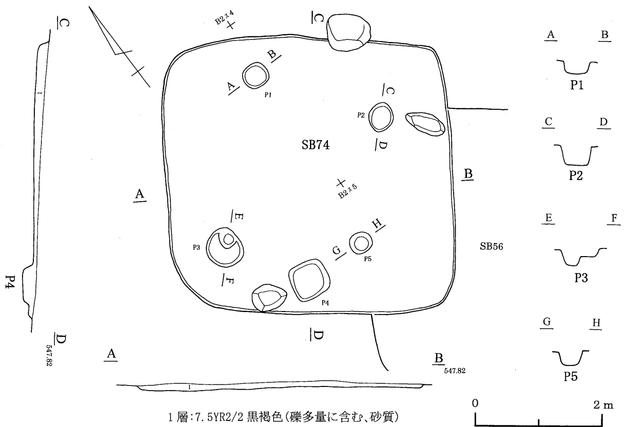
第146図 74号住居跡
