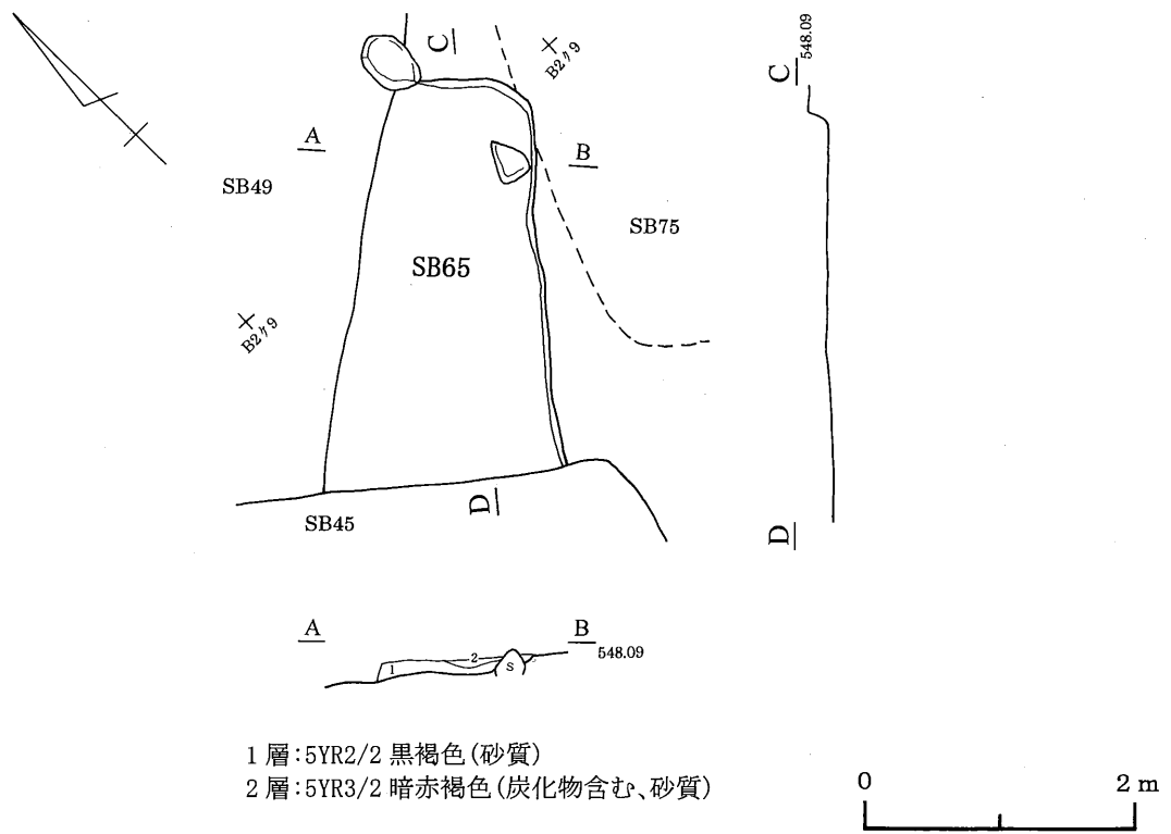
第141図 65号住居跡
