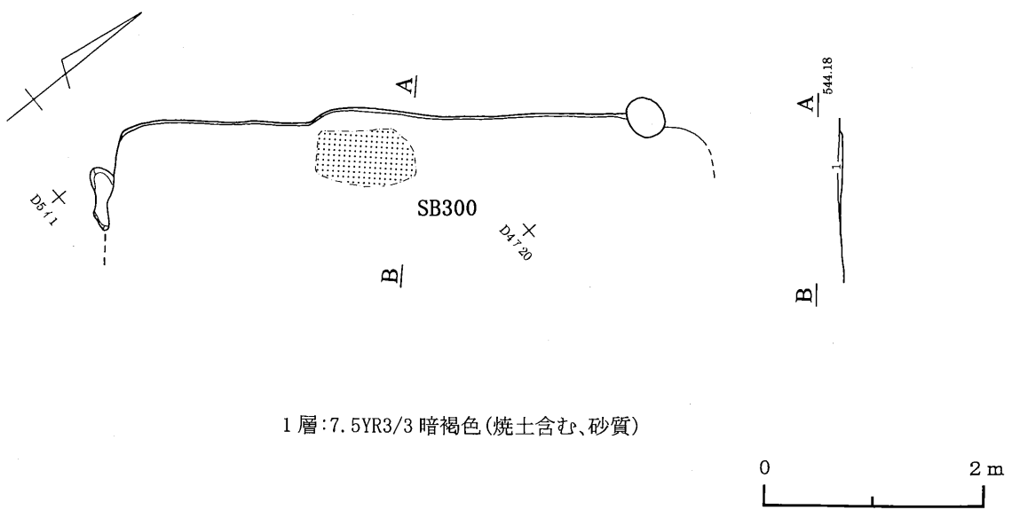
第198図 300号住居跡
