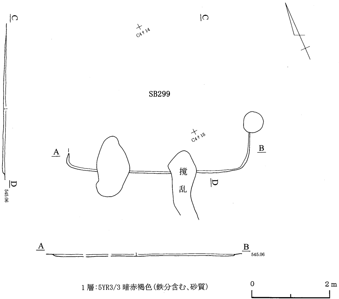
第197図 299号住居跡
