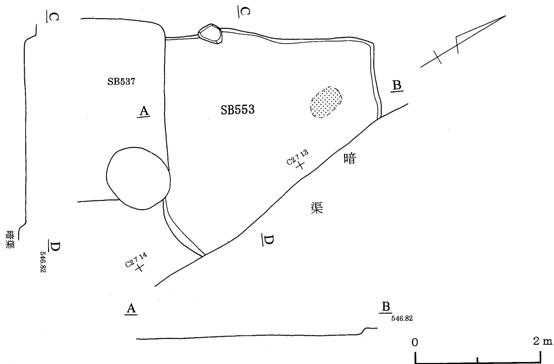
第123図 553号住居跡
