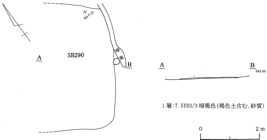
第195図 290号住居跡
