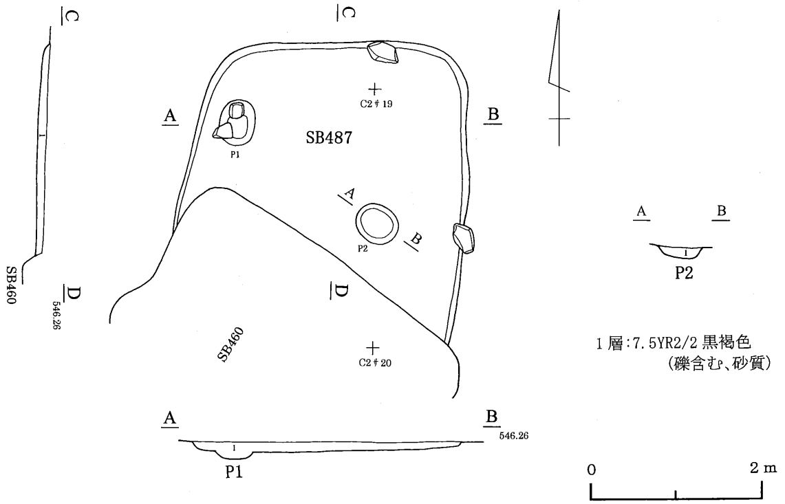
第225図 487号住居跡
