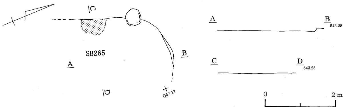
第186図 265号住居跡
