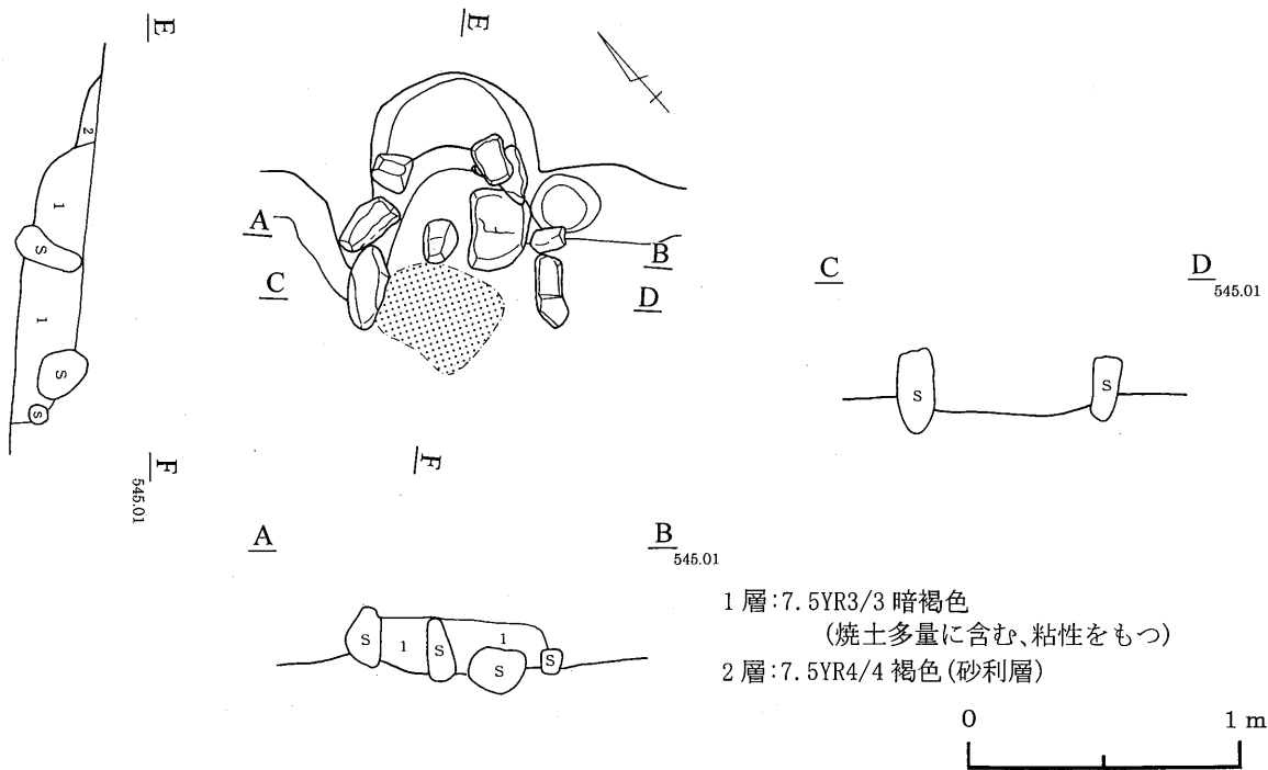
第54図 374号住居跡
