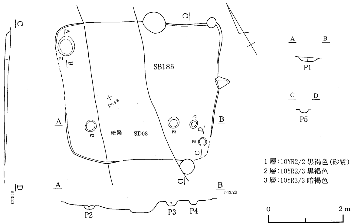
第176図 185号住居跡
