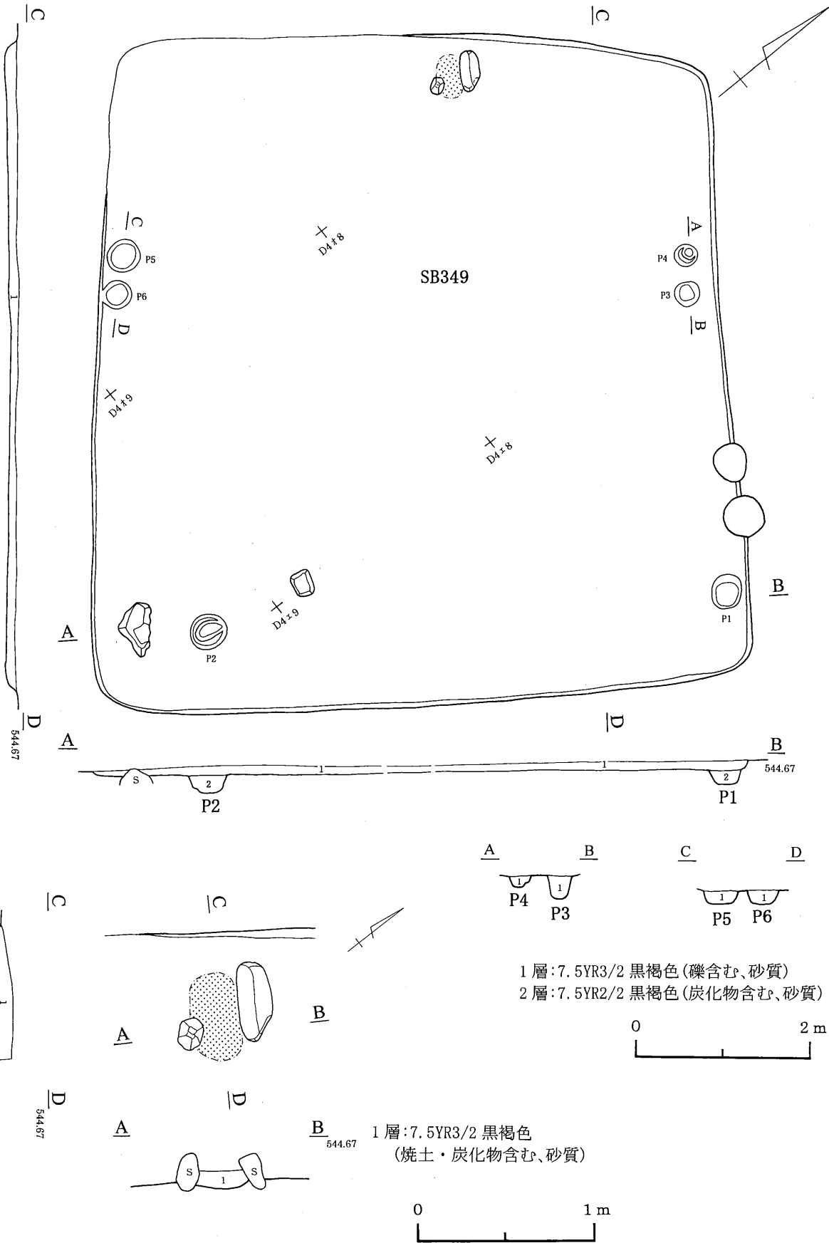
第46図 349号住居跡
