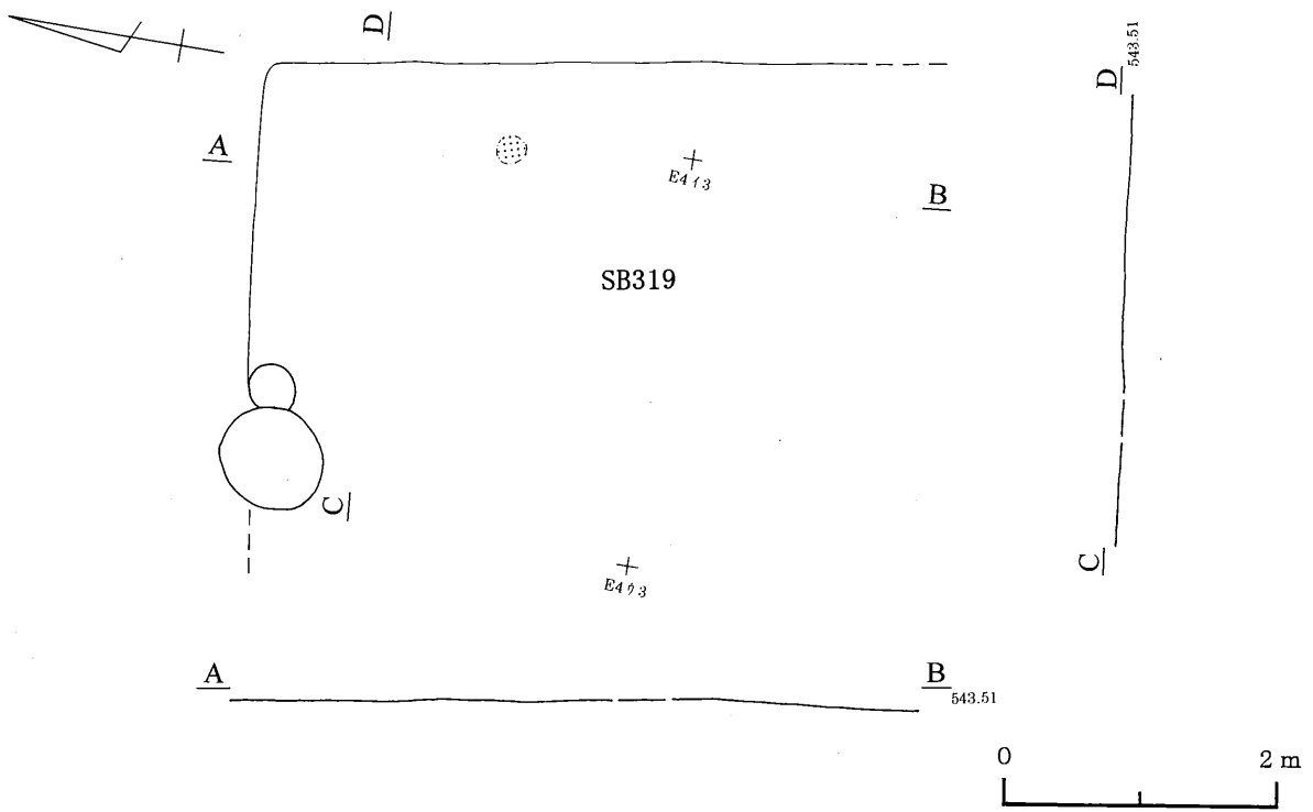
第203図 319号住居跡
