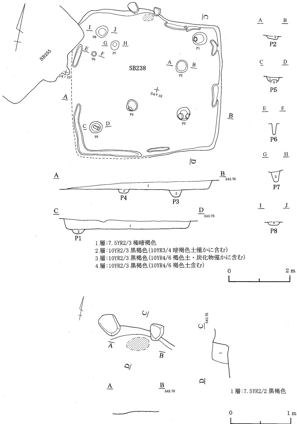
第12図 238号住居跡
