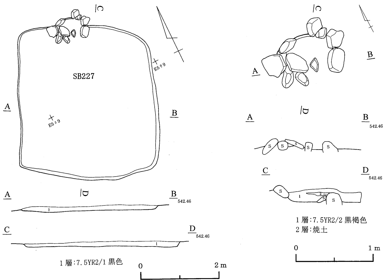
第5図 227号住居跡
