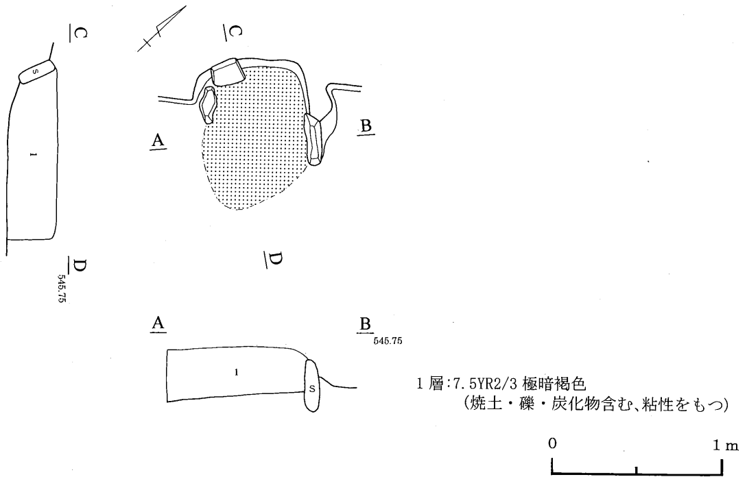
第77図 420号住居跡
