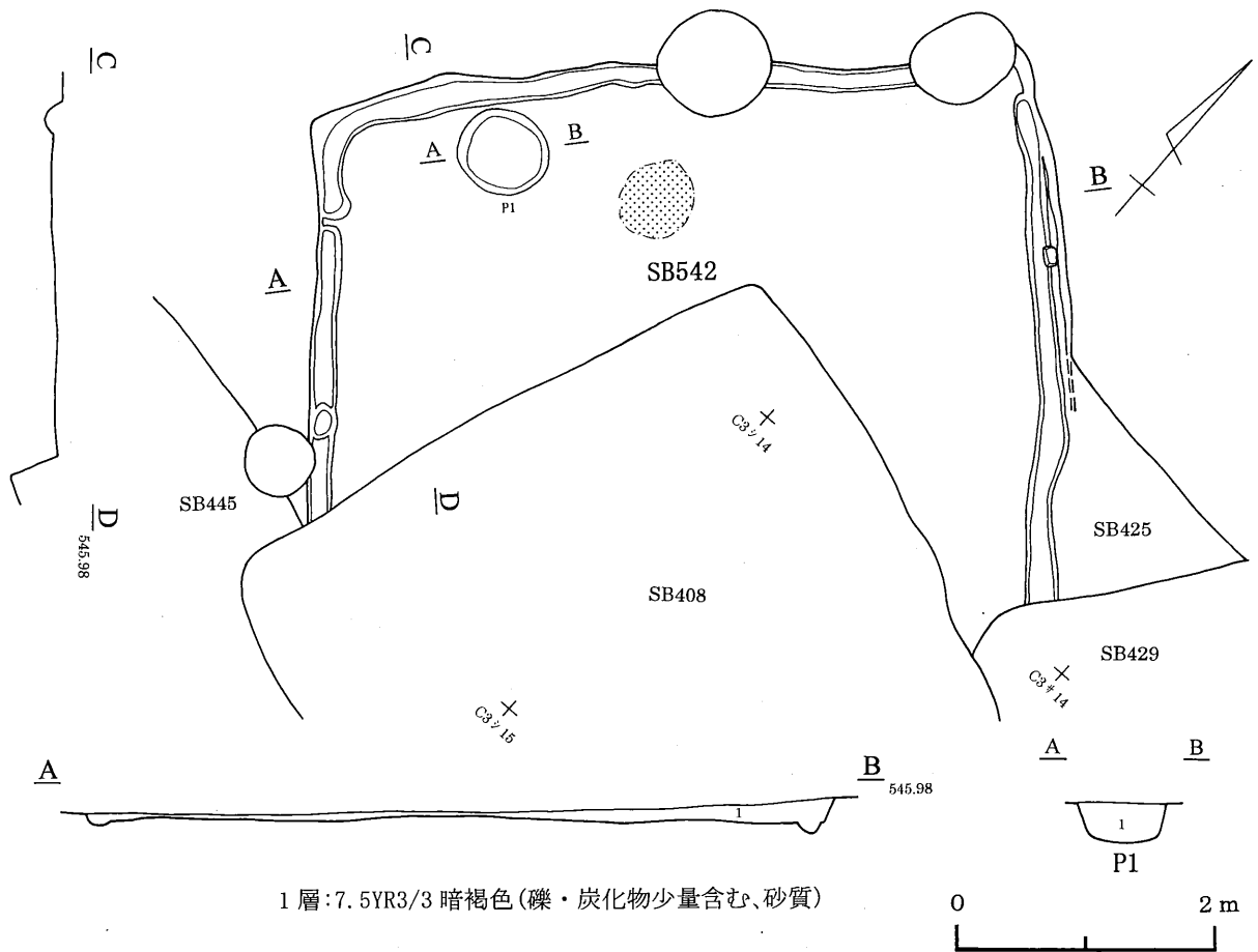
第235図 542号住居跡
