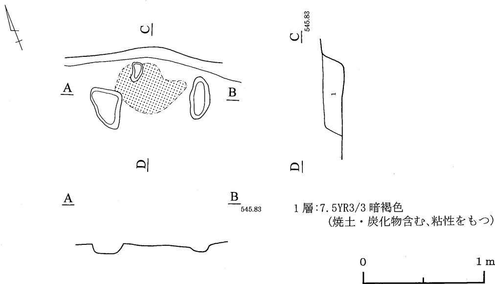
第93図 458号住居跡
