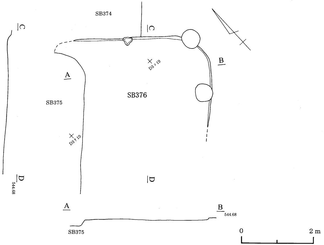
第215図 376号住居跡
