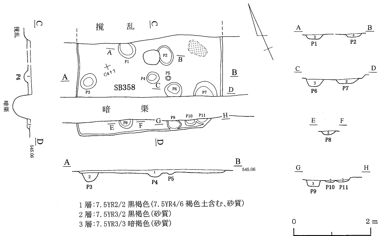
第47図 358号住居跡
