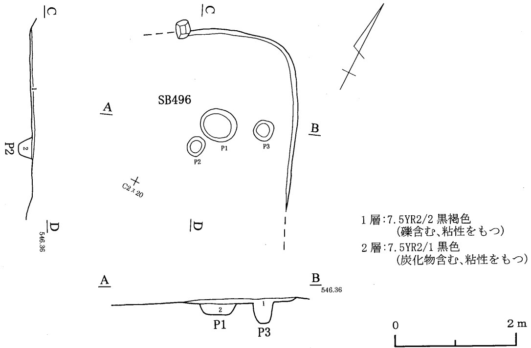
第227図 496号住居跡
