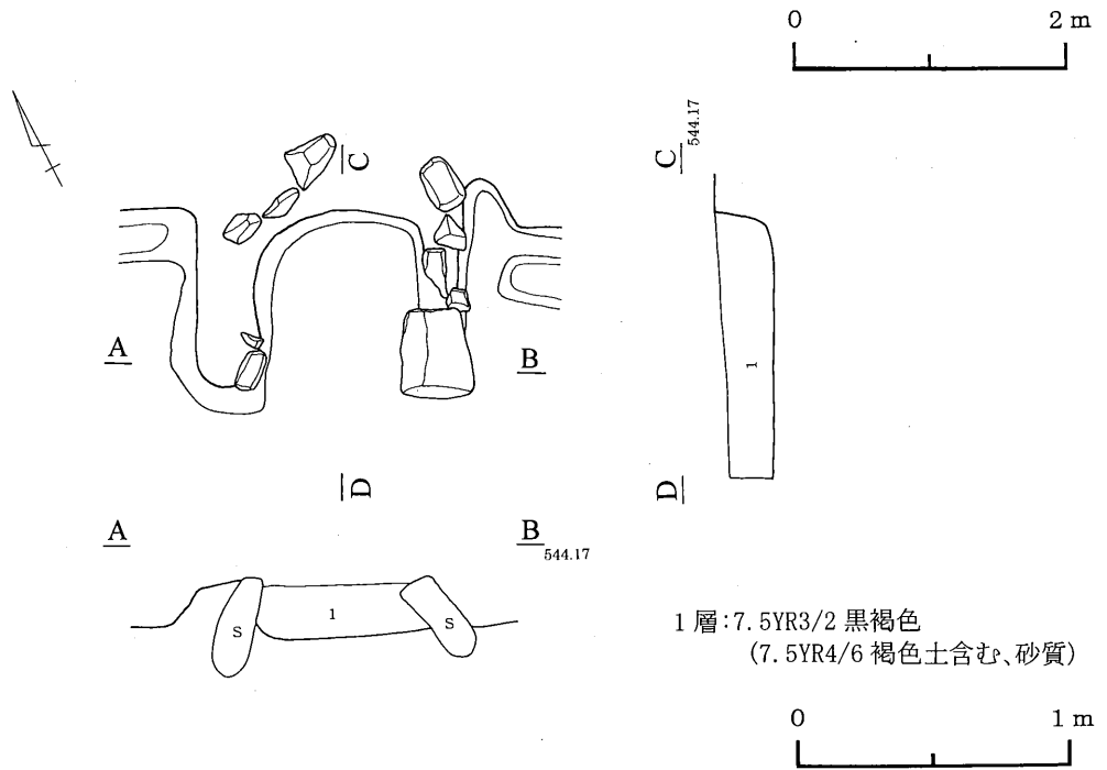
第38図 320号住居跡② (カマド)
