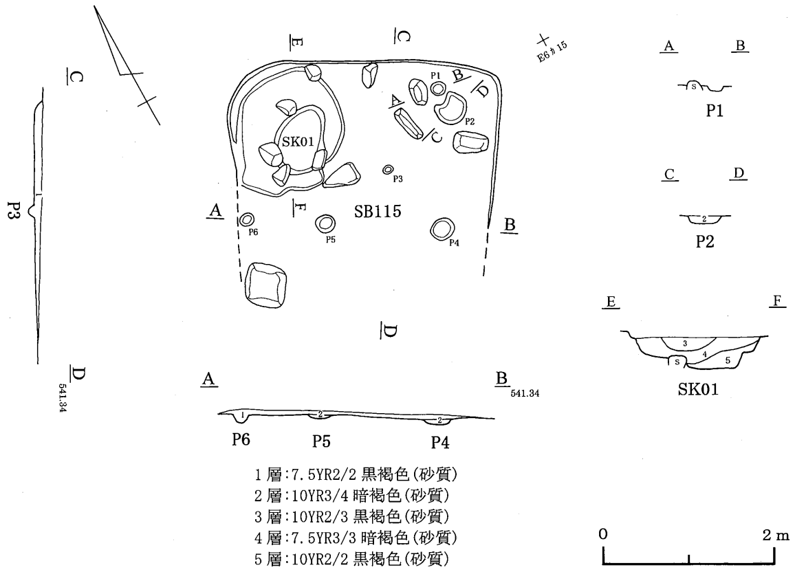
第156図 115号住居跡
