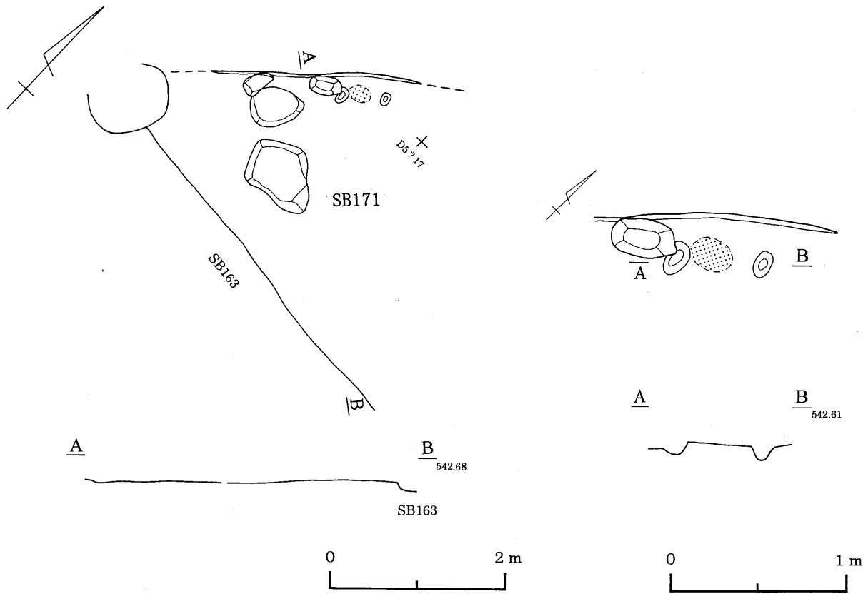
第169図 171号住居跡
