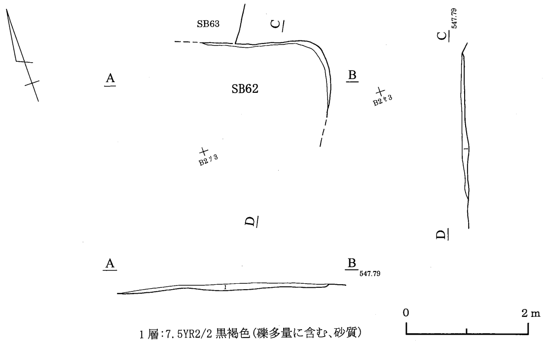
第139図 62号住居跡
