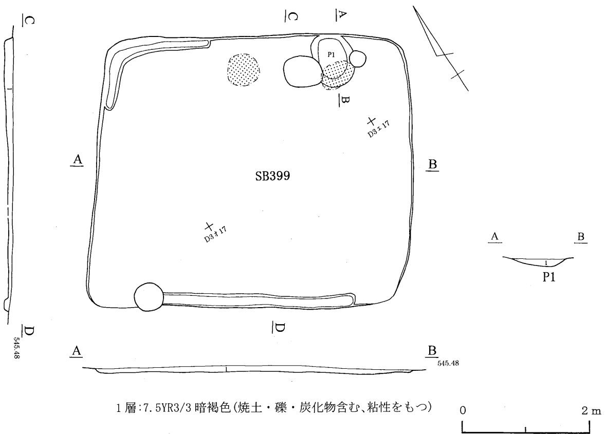
第63図 399号住居跡
