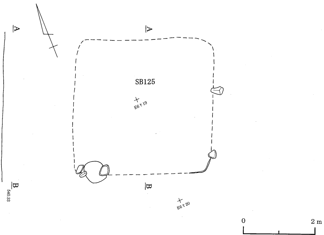
第159図 125号住居跡
