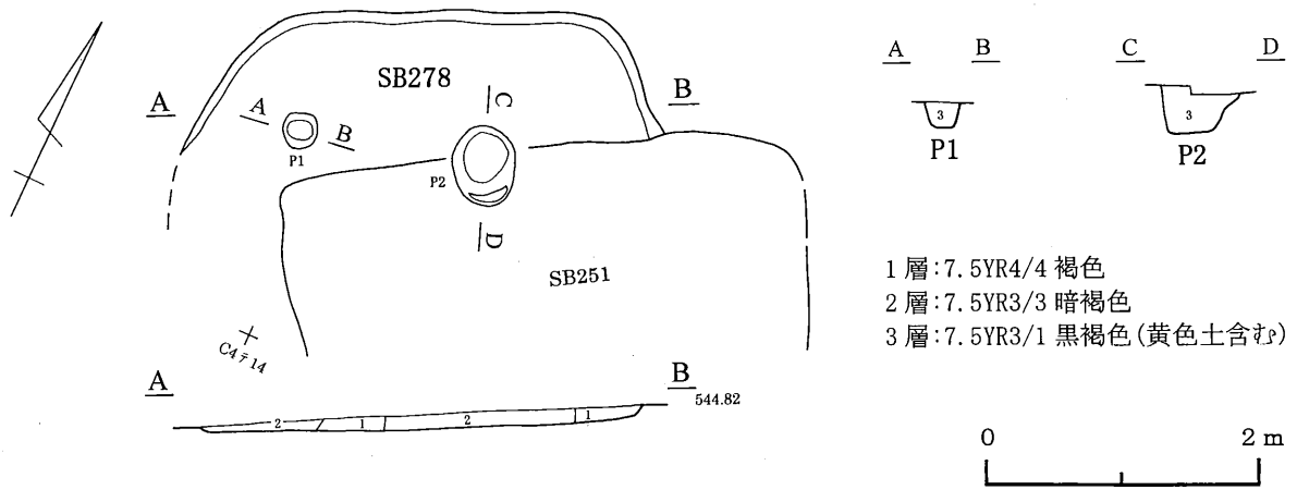
第188図 278号住居跡
