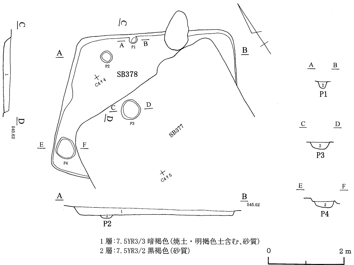
第57図 378号住居跡
