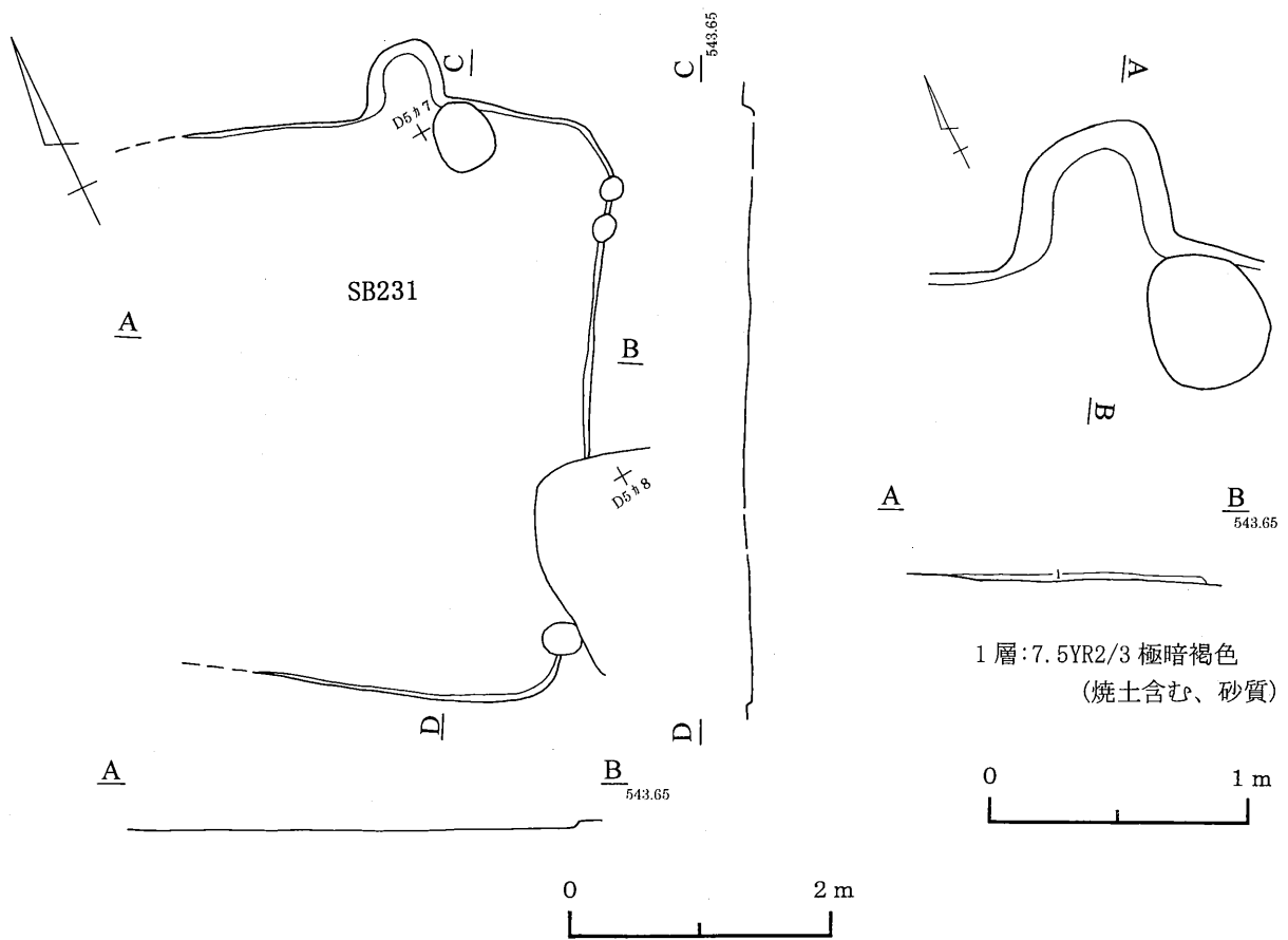
第8図 231号住居跡
