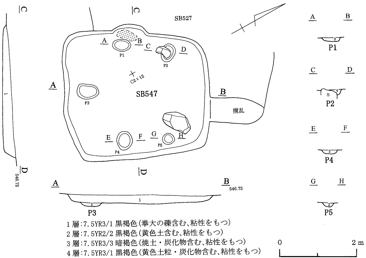
第122図 547号住居跡
