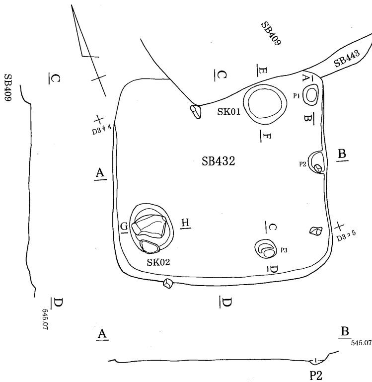
第82図 431号住居跡
