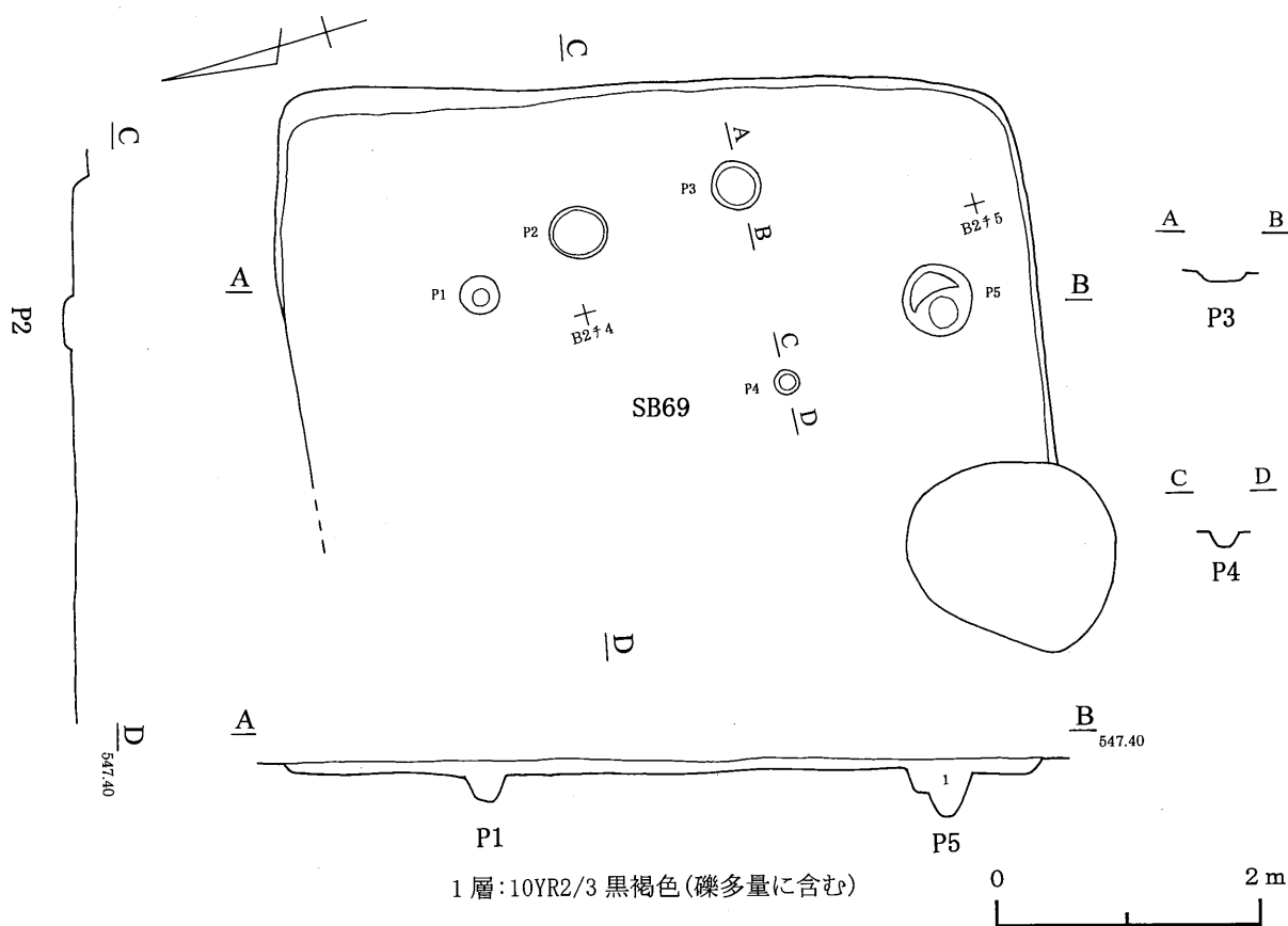
第143図 69号住居跡
