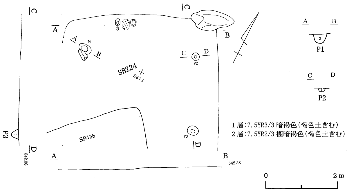
第180図 224号住居跡①
