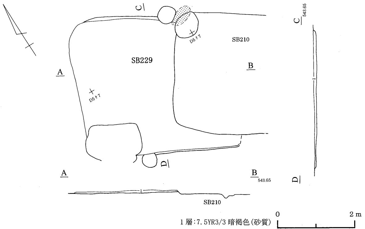
第7図 229号住居跡
