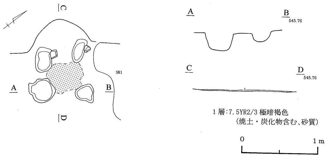
第217図 390号住居跡
