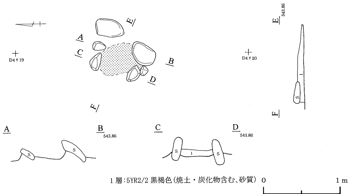
第10図 239号住居跡 (カマド)
