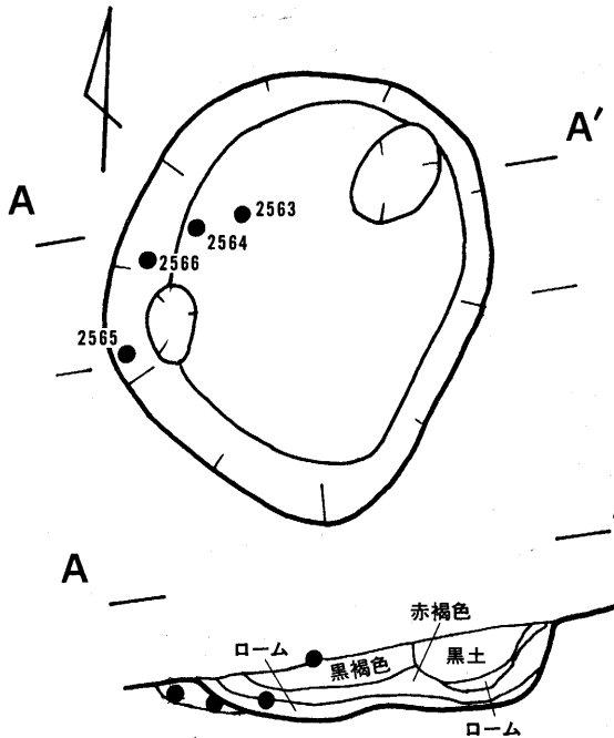
図9. 第1号土壇 S=40
