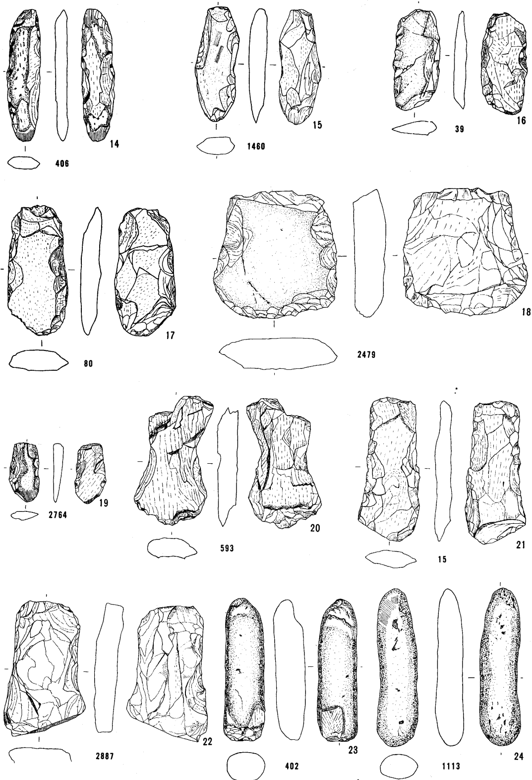
图18 打製石斧·磨製石斧实测图(1/3)
