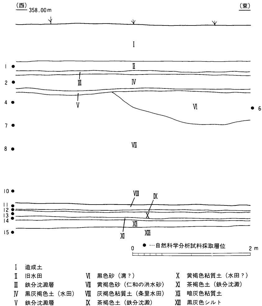
第3図 基本層序
