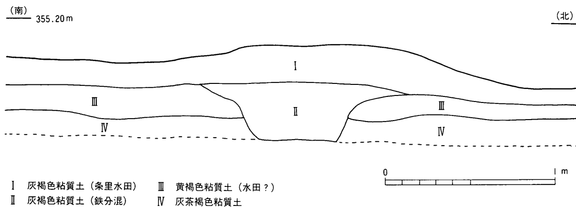
第5図 1号畦畔断面
