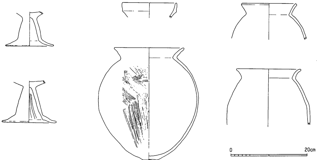
第10図 自然流路内出土遺物 (平成9年調査)
