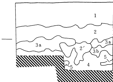
第30図 KRD245～247グリッド土層断面図
