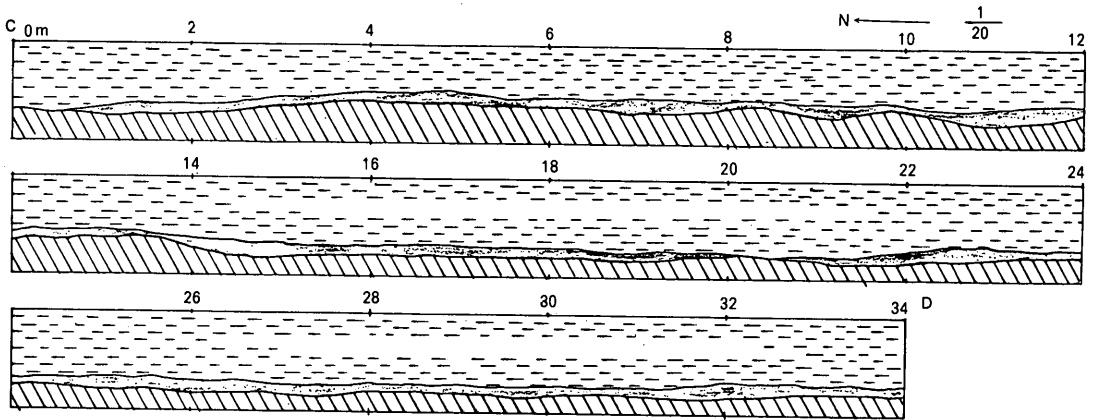
C 地点 (上段) E ←→ F 断面图
