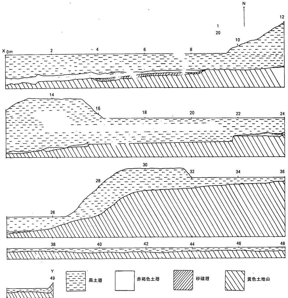
ABC地点(下·中·上段) G←→H断面图
