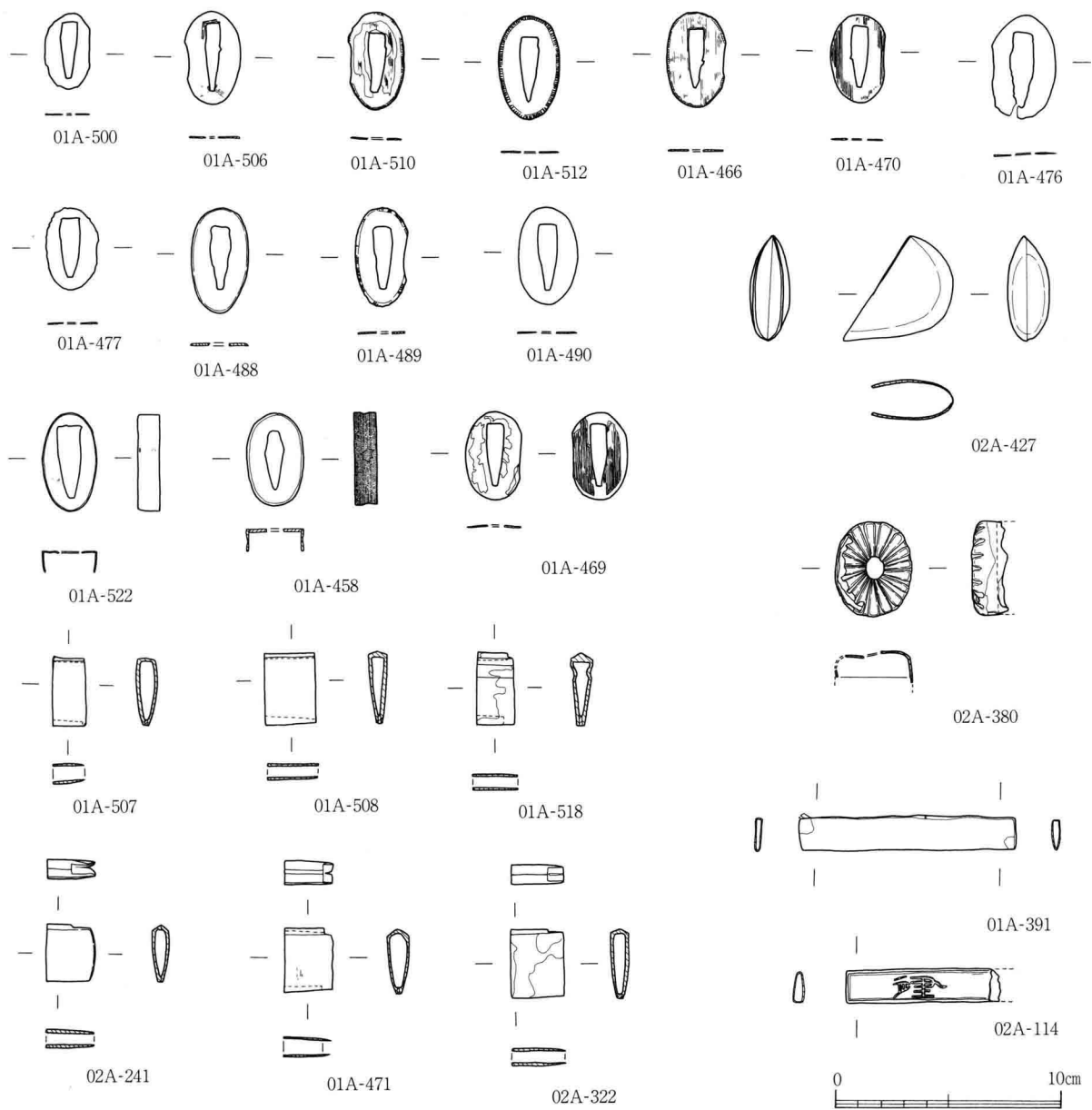
第86图 刀装具实测图 (S=1/3)
