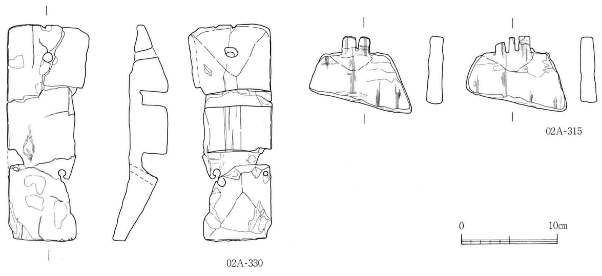
第95図 木製品実測図③ (S=1/4)
