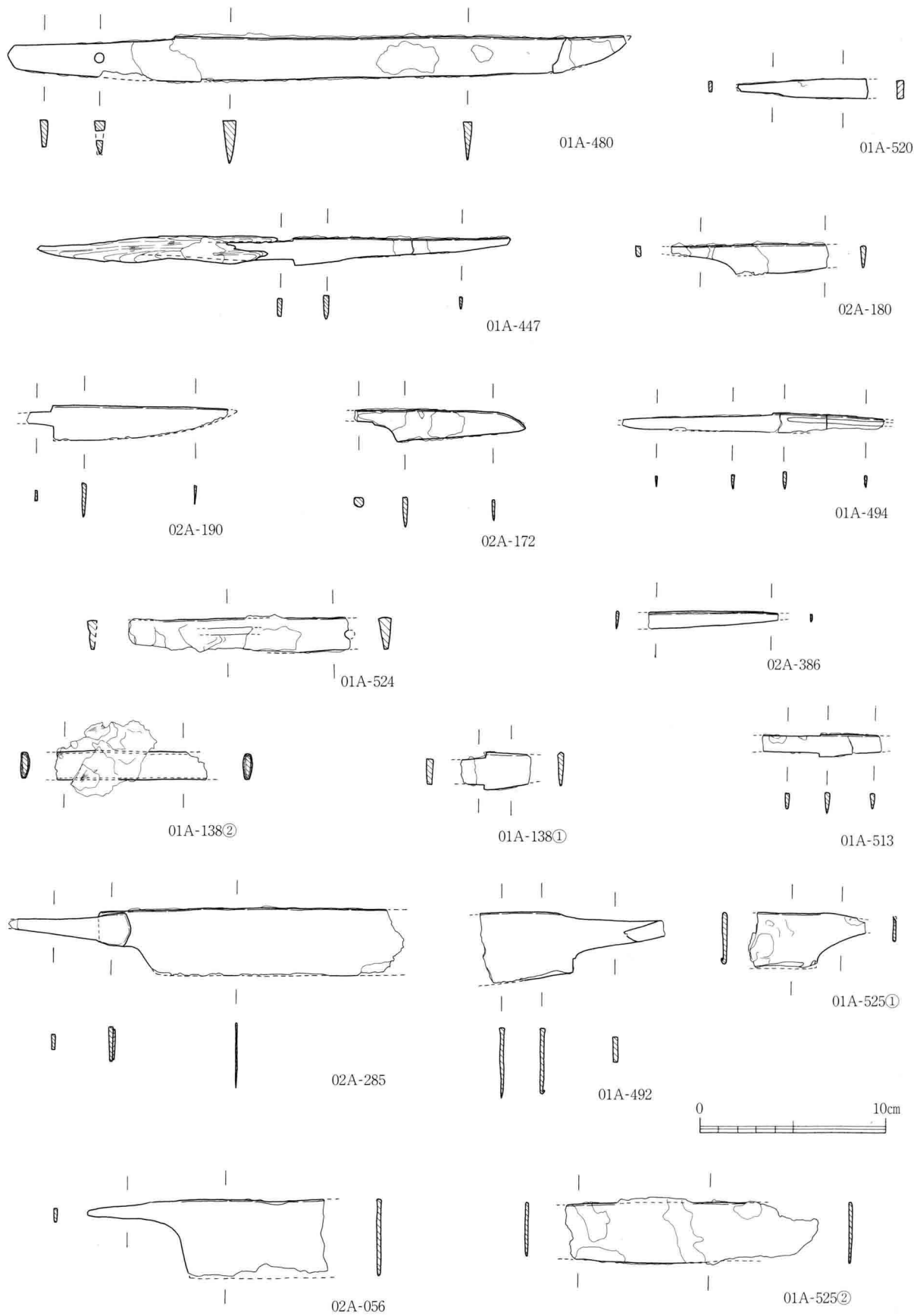
第83図 鉄製品実測図① (S=1/3)
