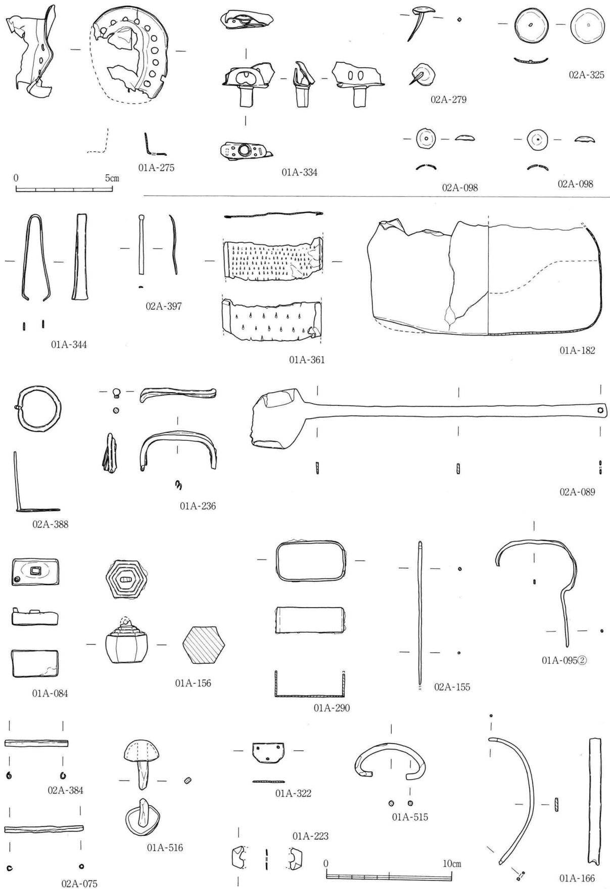
第89図 銅製品実測図② (S=1/2,1/3)
