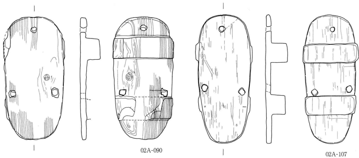
第93図 木製品実測図① (S=1/4)
