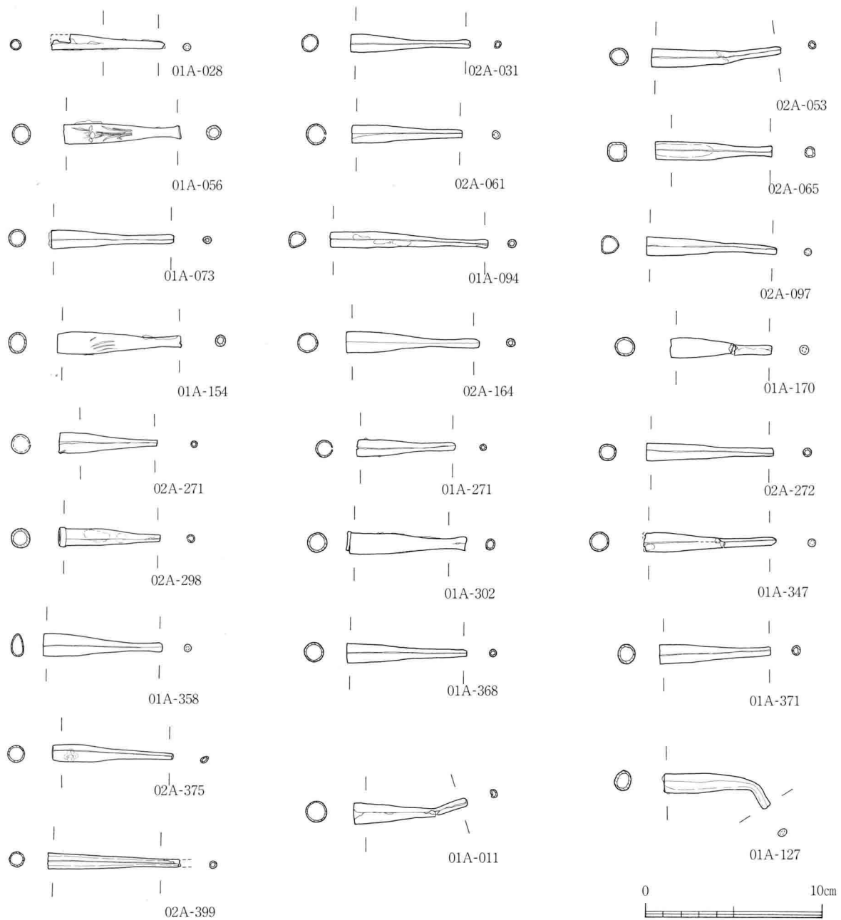
第92図 煙管実測図② (S=1/3)
