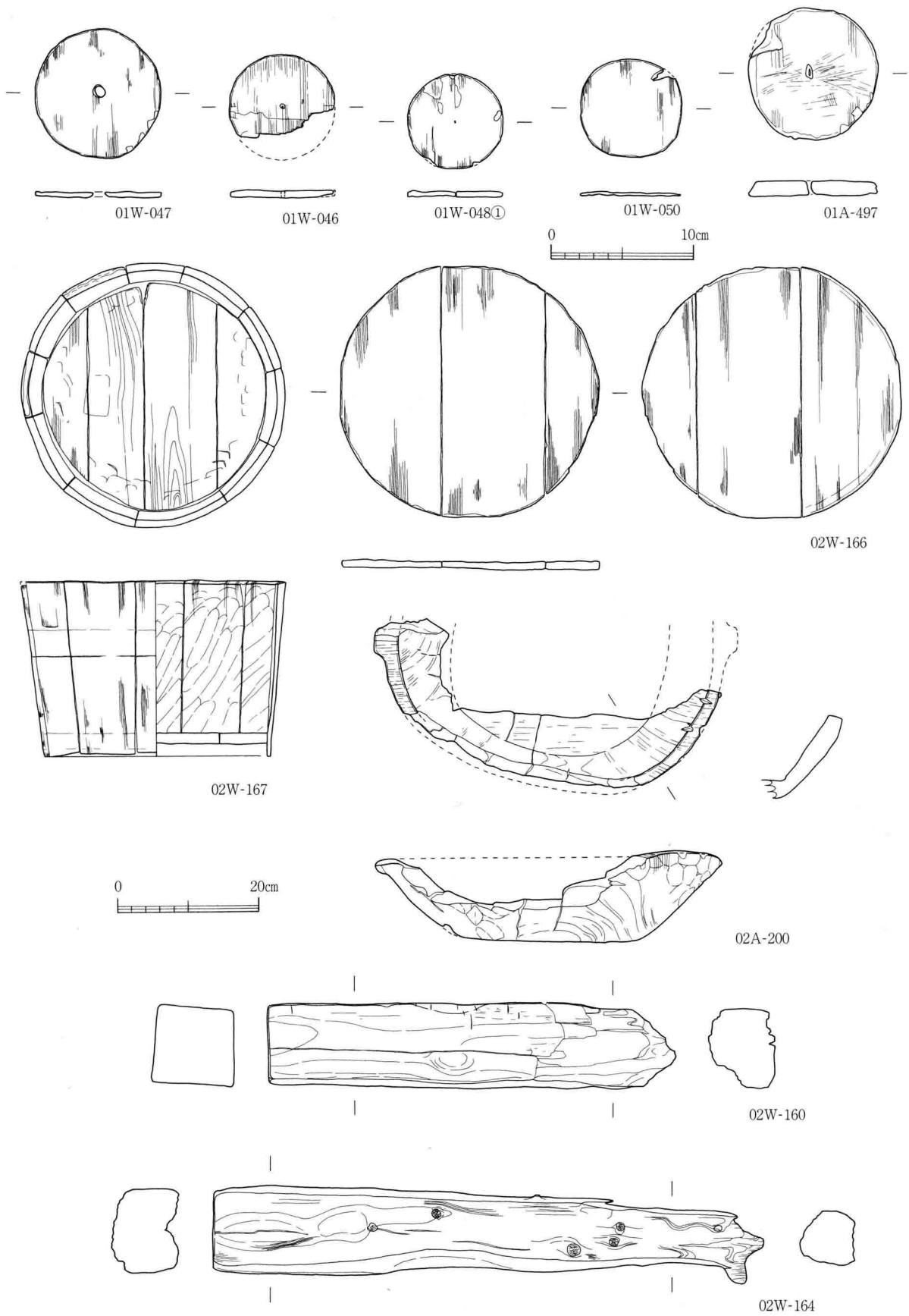
第98図 木製品実測図⑥ (S=1/4, 1/8)
