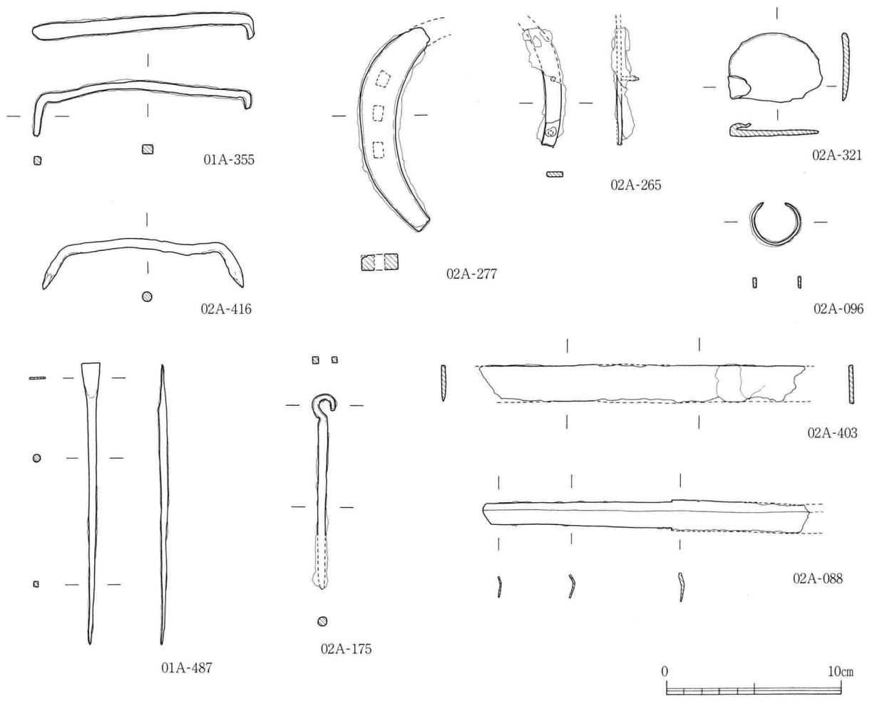
第85図 鉄製品実測図③ (S=1/3)
