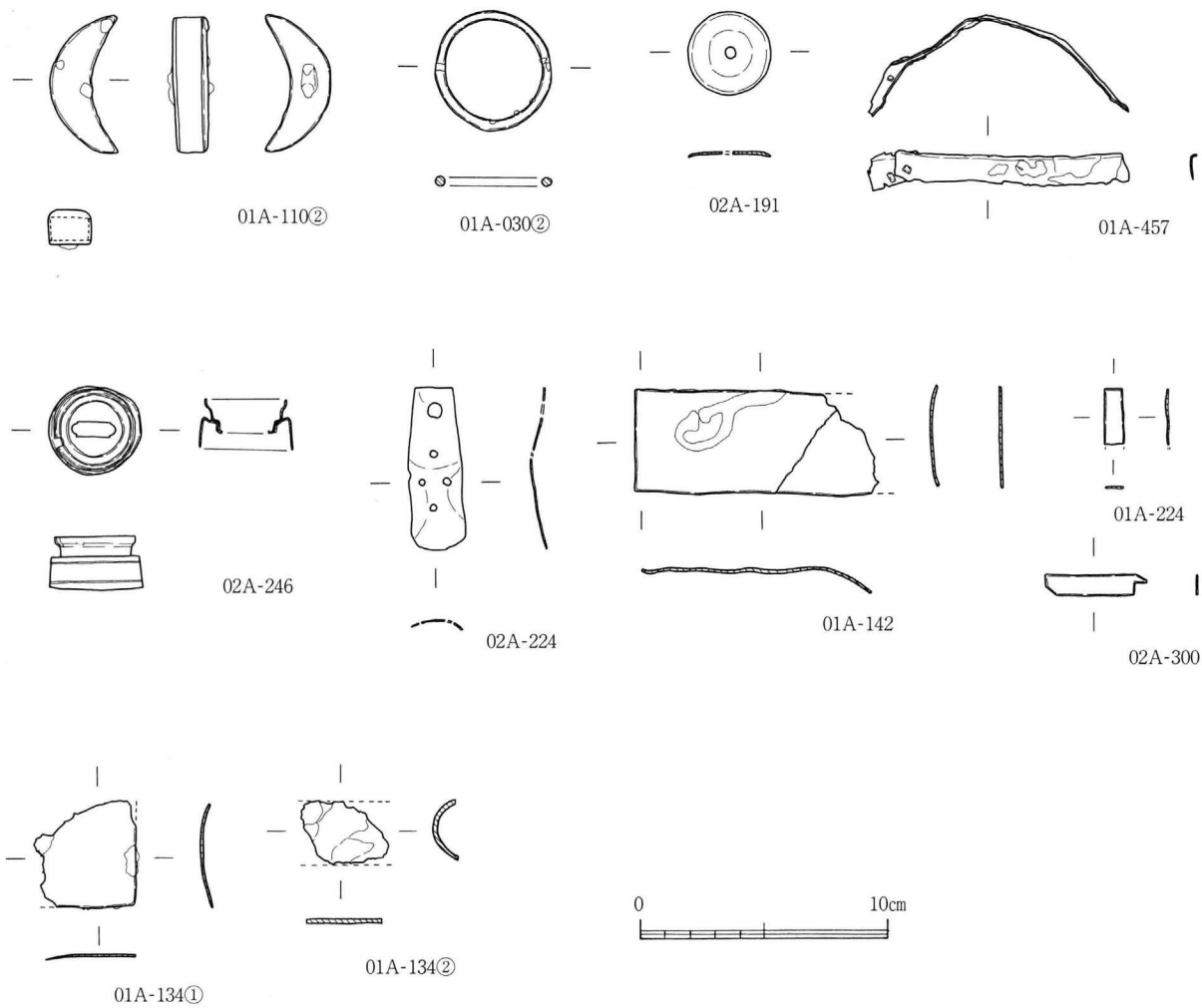
第90図 銅製品実測図③ (S=1/3)
