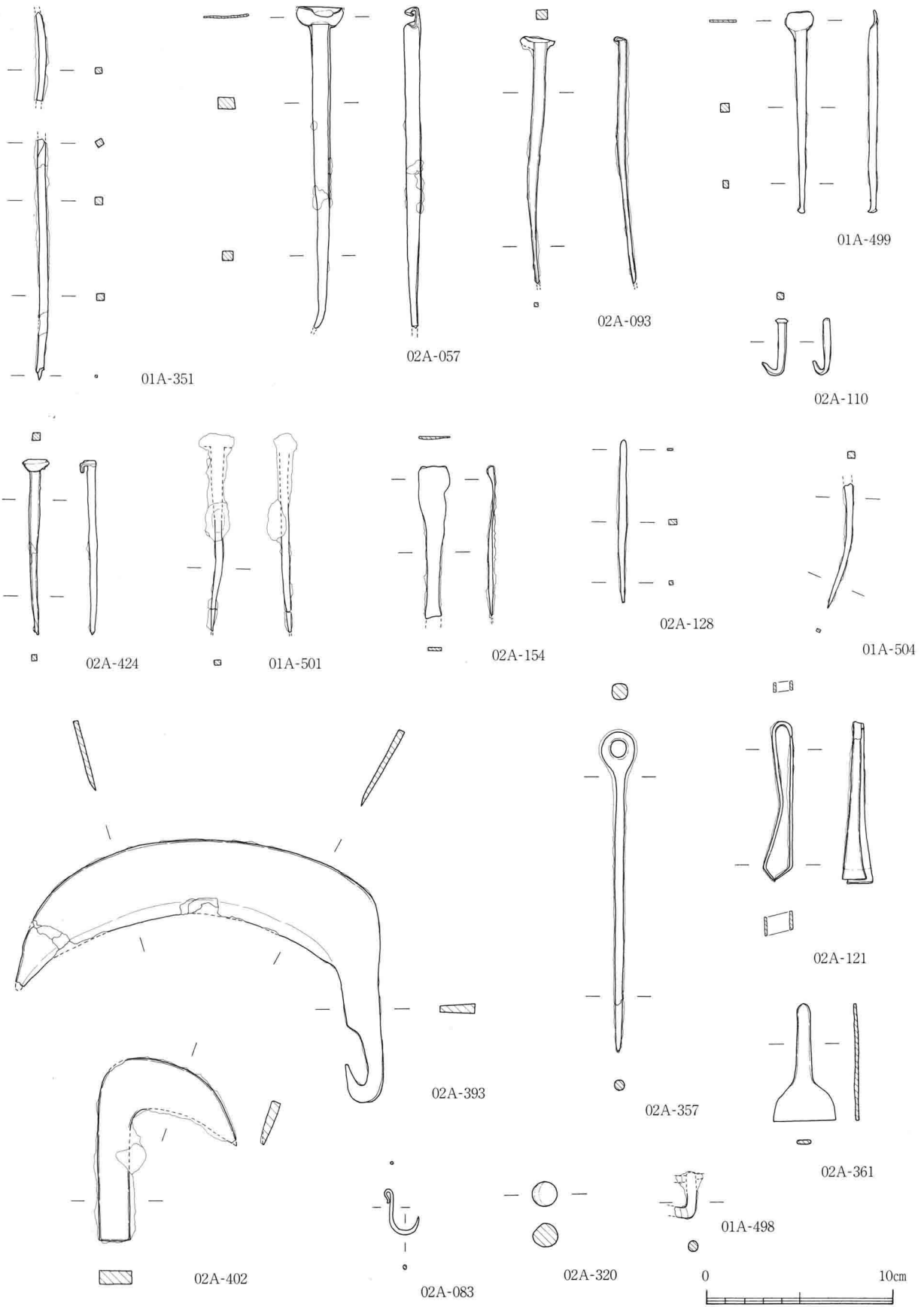
第84図 鉄製品実測図② (S=1/3)
