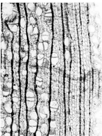
16. KK-640 下駄 ハンノキ属 x75
