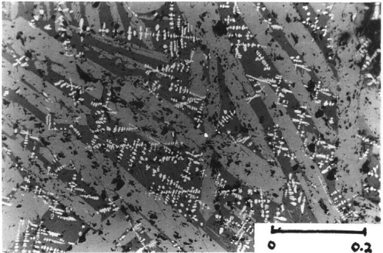
微細組織 金属鉄 (中央白点) ファイヤライト (灰色) マグネタイト (白色)
