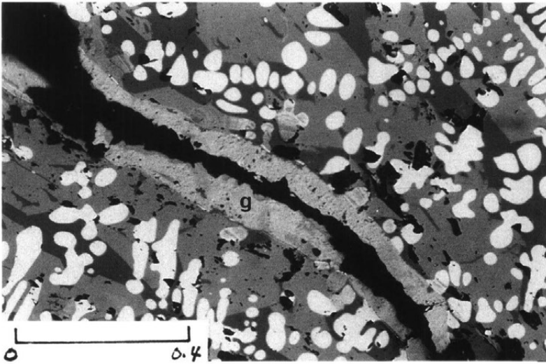
空隙部 針鉄鉱 \delta ウスタイト (白玉) ファイヤライト (灰色)
