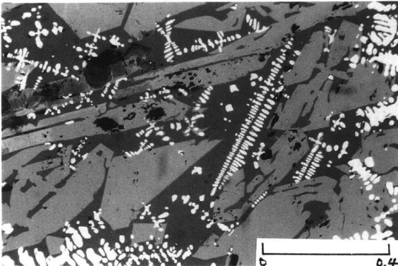
微細組織 ファイヤライト (灰色) マグネタイト (白色)
