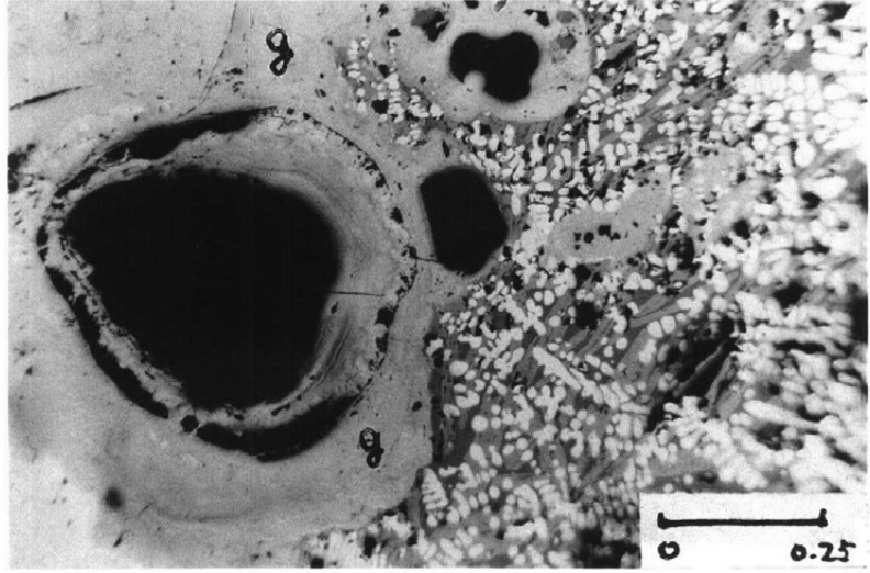
空隙部 針鉄鉱 g ウスタイト (白玉) ファイヤライト (灰色)
