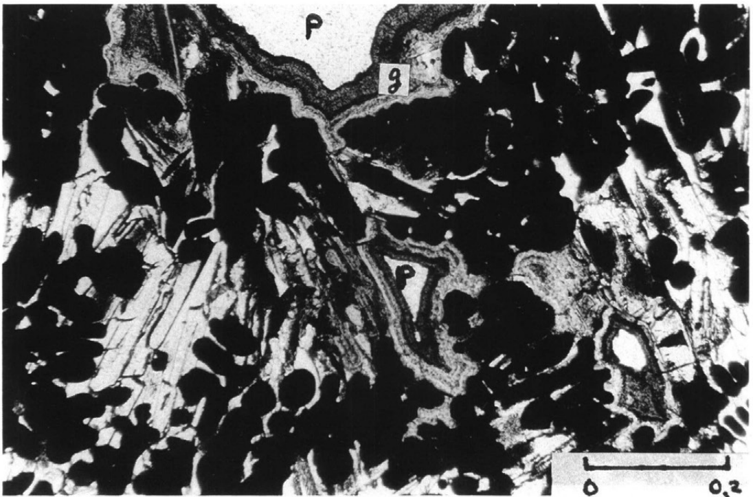
空隙部 空隙 (P) 針鉄鉱 (g)
