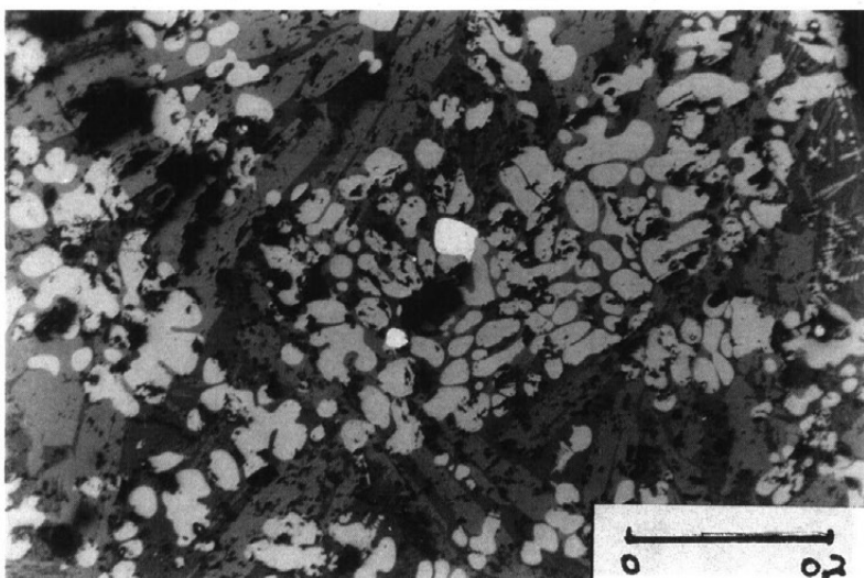
微細組織 金属鉄 (中央白色) ウスタイト (白玉) ファイヤライト (灰色) マグネタイト (右)
