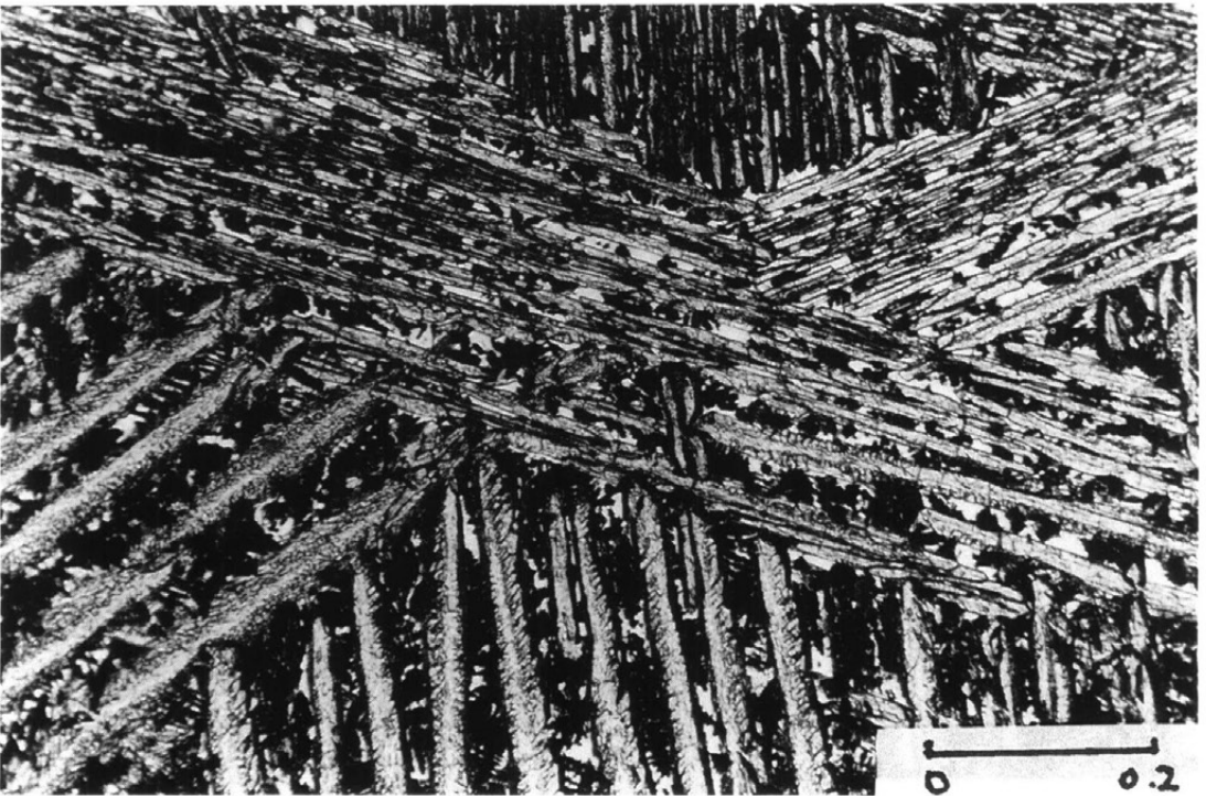
一般組織 ファイヤライトの間にウスタイト・マグネタイトがわずかに主成
