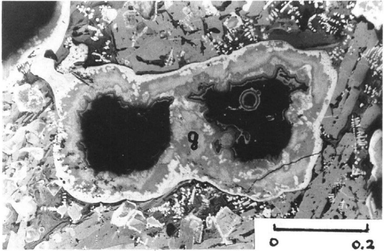
空隙部 針鉄鉱 g ファイヤライト (灰色) マグネタイト (小白点)
