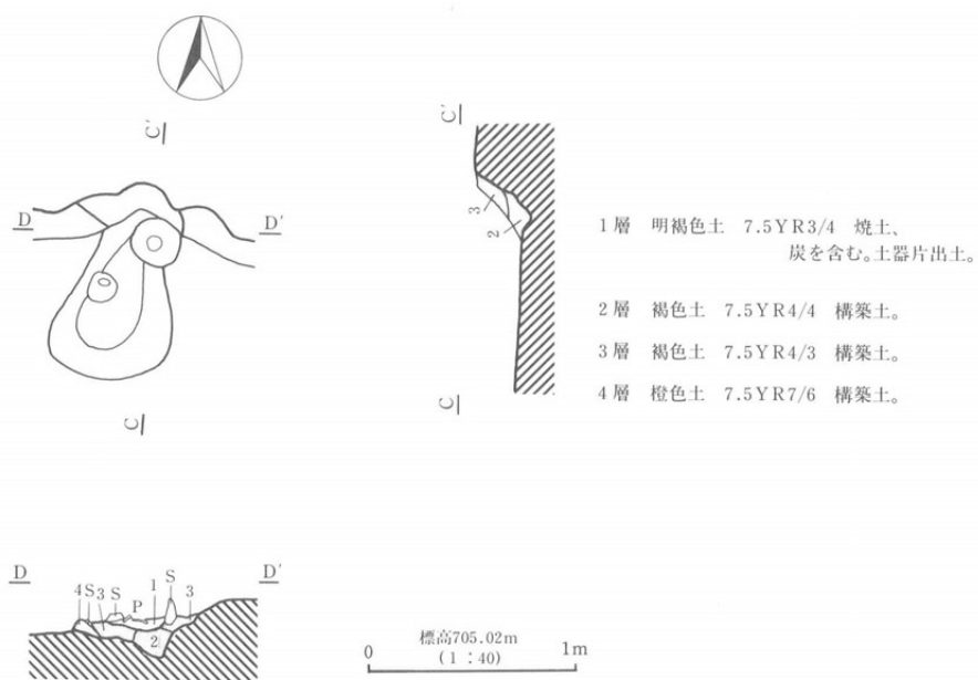
第19図 H5号住居址カマド実測図
