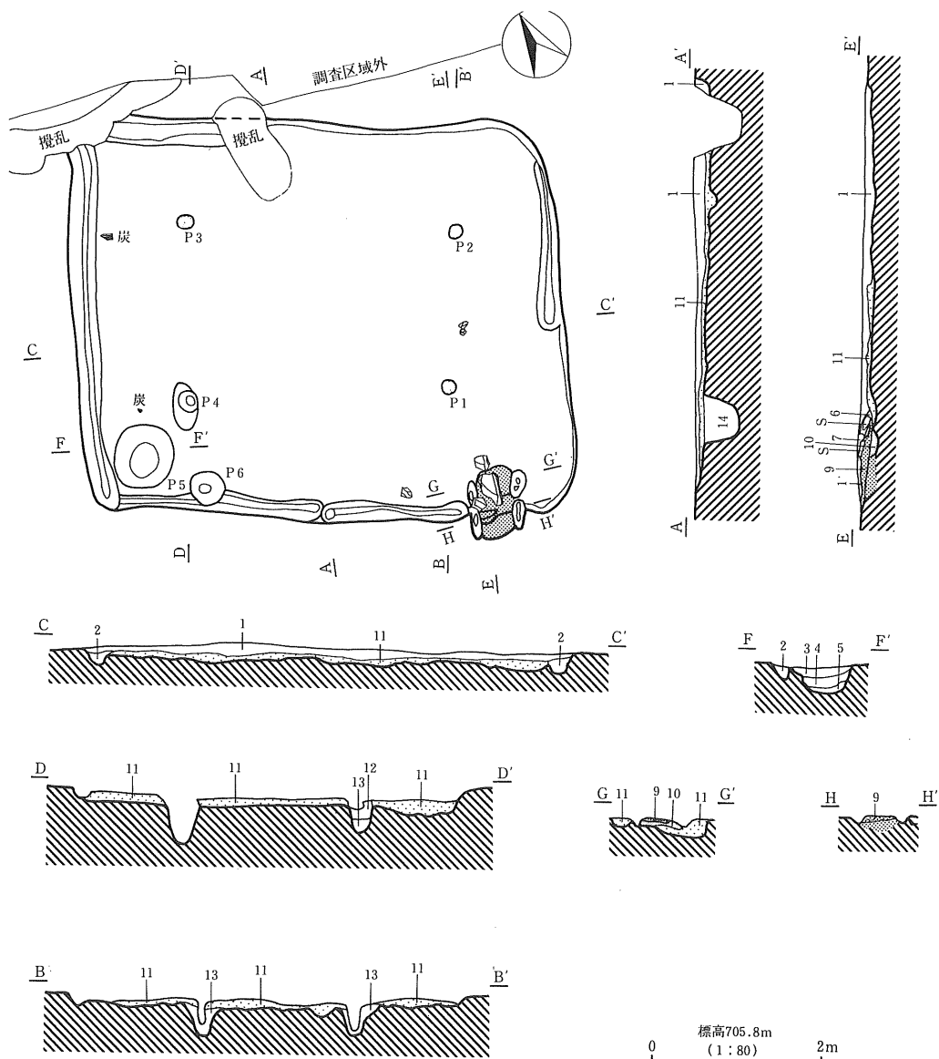
第5図 H1号住居址実測図
