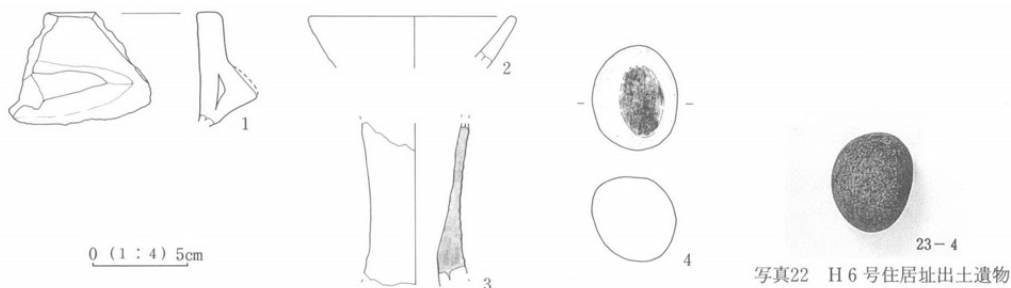
第23図 H6号住居址出土遺物実測図
