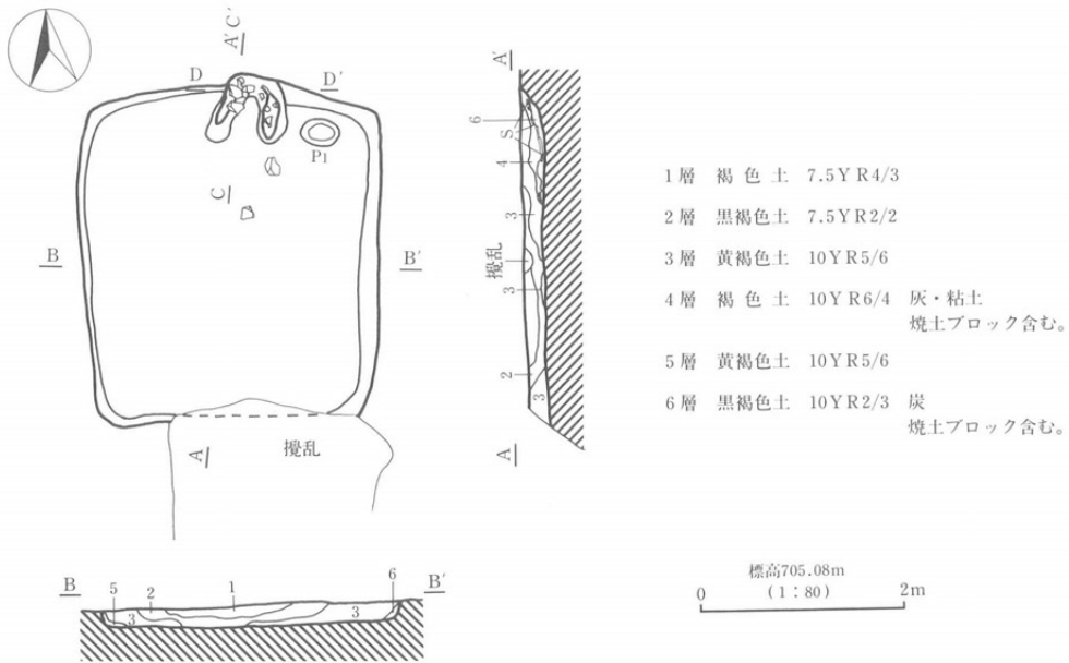
第18図 H5号住居址実測図
