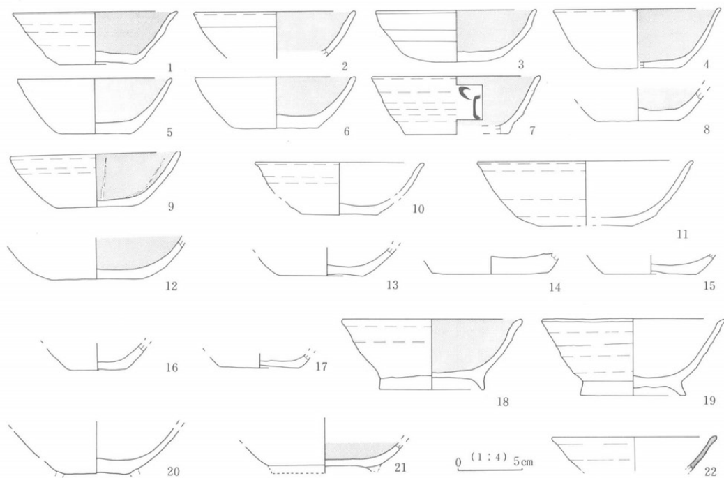
第12图 H3号住居址出土遺物実測図
