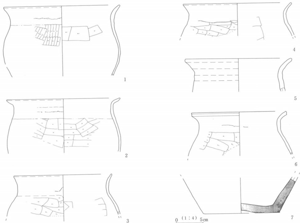
第13图 H3号住居址出土遺物実測図
