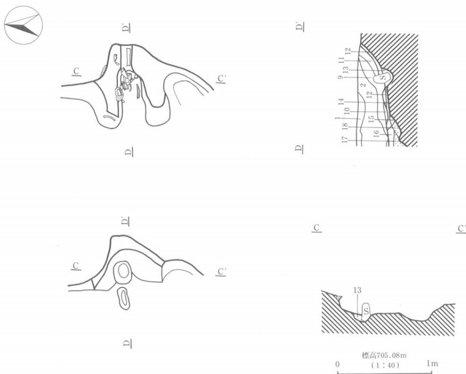
第24図 H7号住居址カマド実測図
