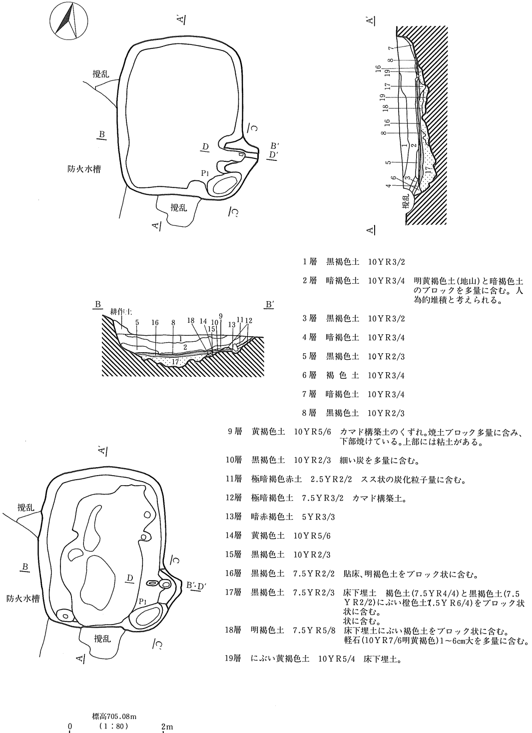
第26図 H7号住居址実測図
