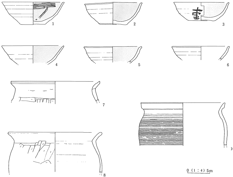
第16図 H4号住居址出土遺物実測図
