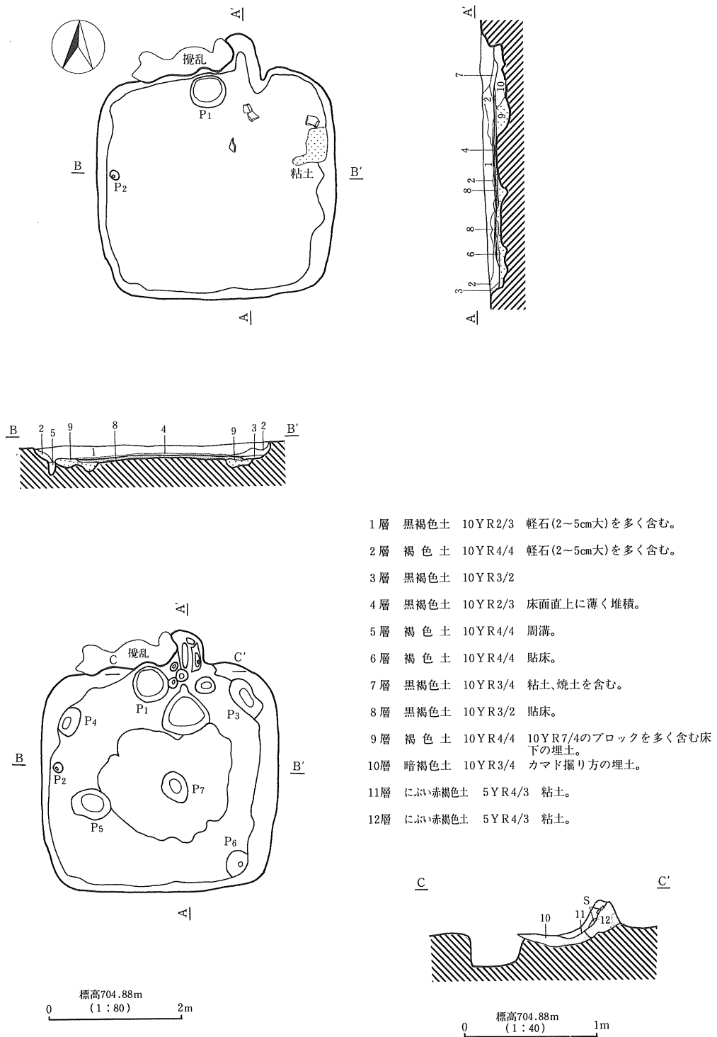
第15図 H4号住居址実測図
