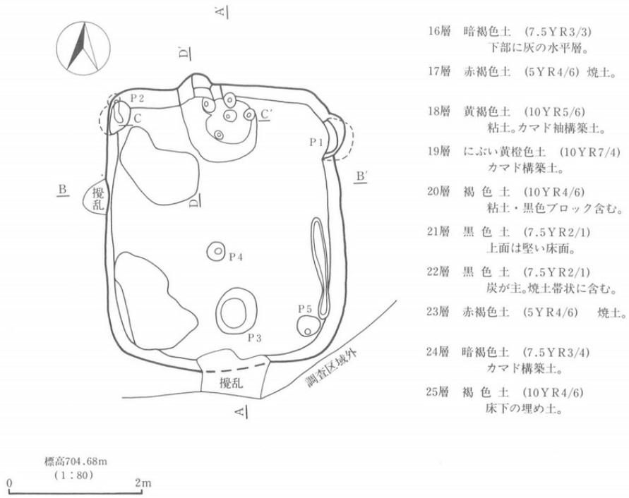
第10図 H3号住居址掘り方実測図
