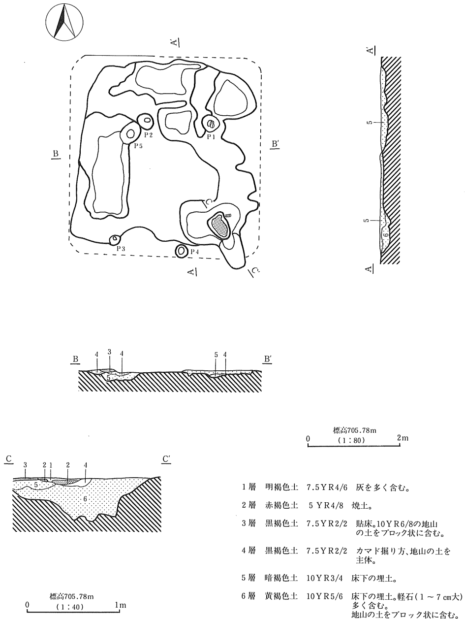
第8図 H2号住居址実測図
