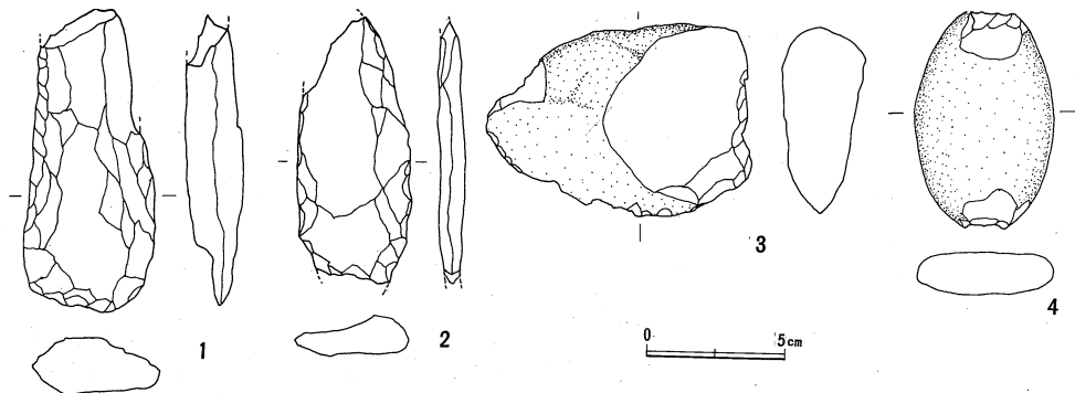
第14図 石器実測図(1:3)
