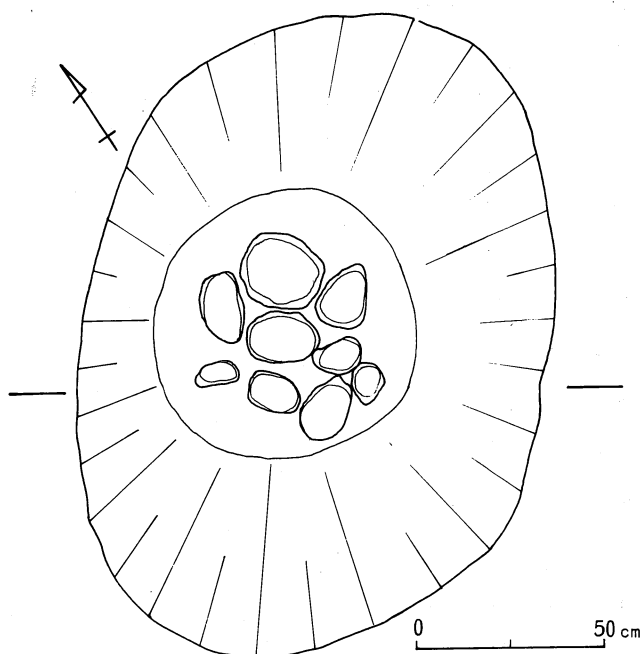
第13図 焼石炉底部
