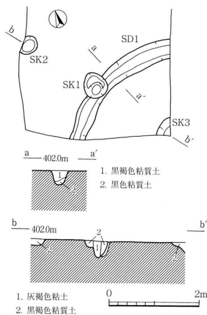
図7 1号溝・土坑 (1:80)
