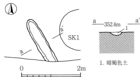
図7 1号溝 (1:80)
