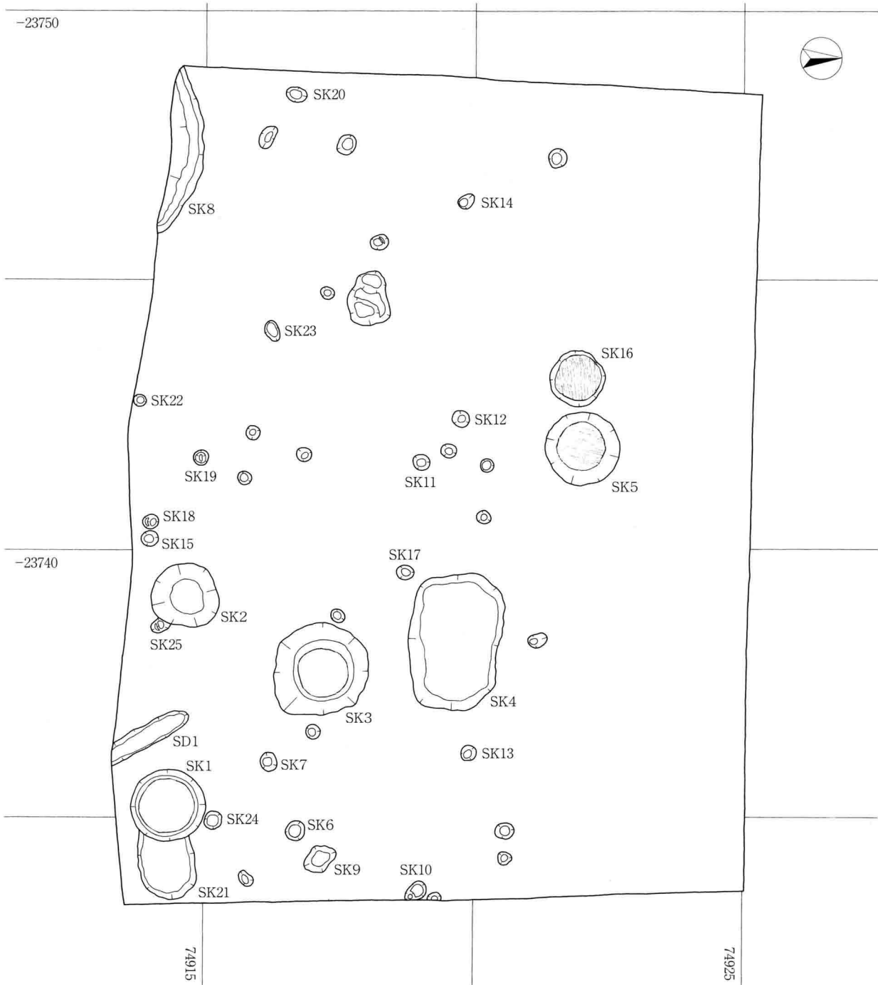
図5 遺構分布図 (1:100)
