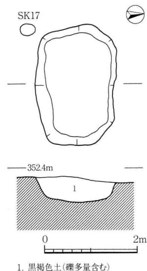
図9 4号土坑 (1:80)
