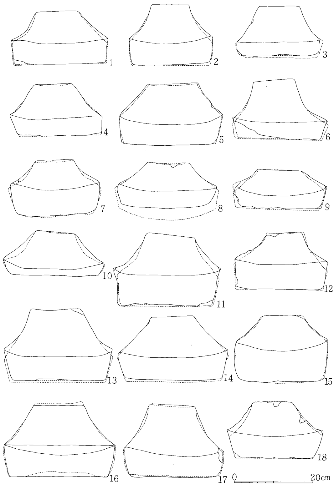
第30图 火輪実測図(1)
