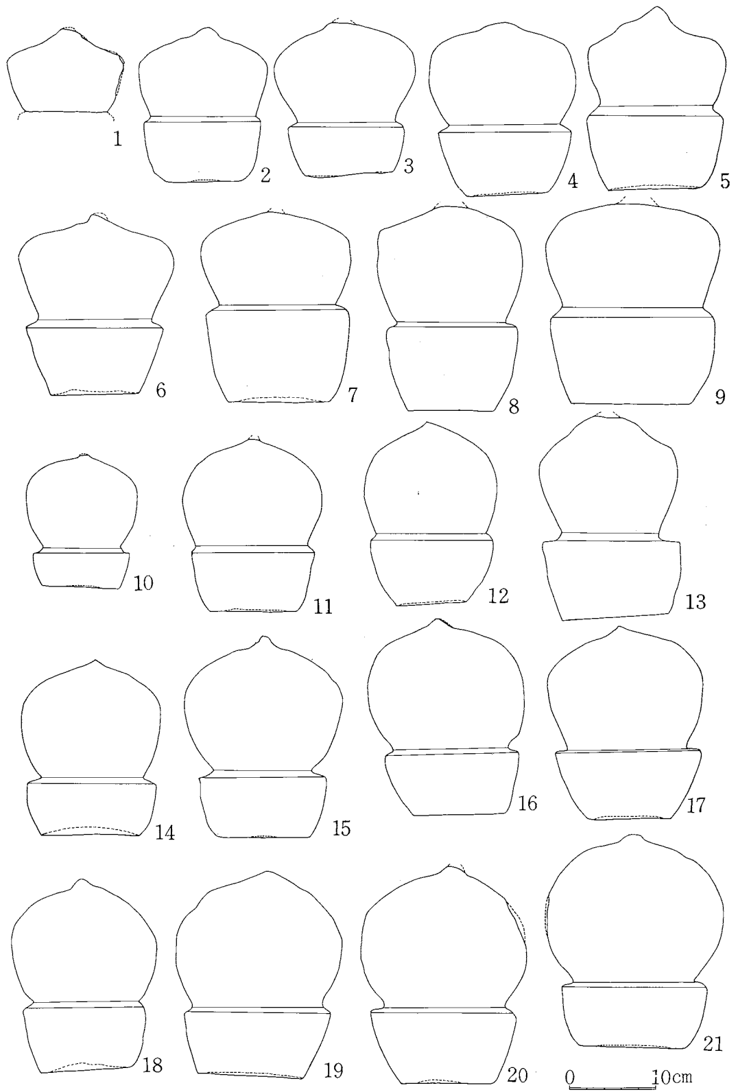
第32図 空・風輪実測図(1)
