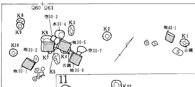
第18図 第IV群支群10実測図
