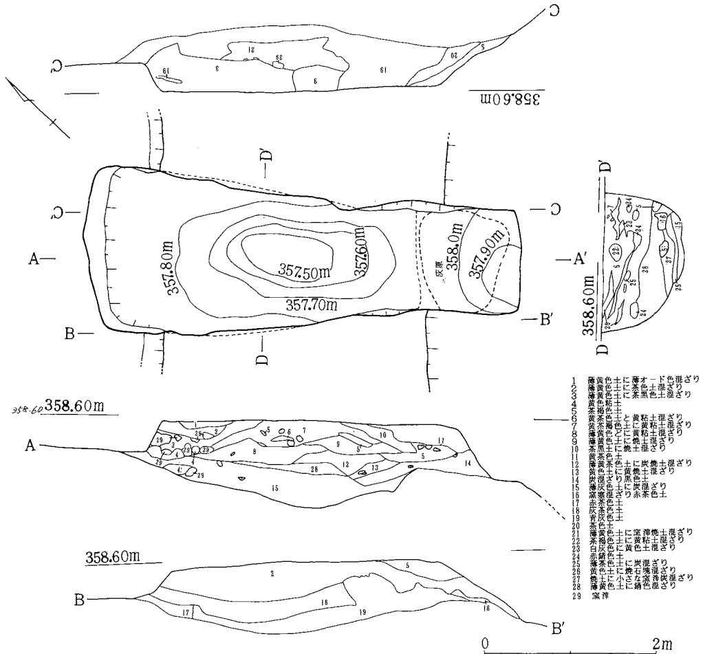
第3図 1号窯址ペルト断面図
