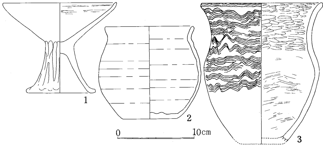
第41図 がまん淵遺跡表採土器実測図
