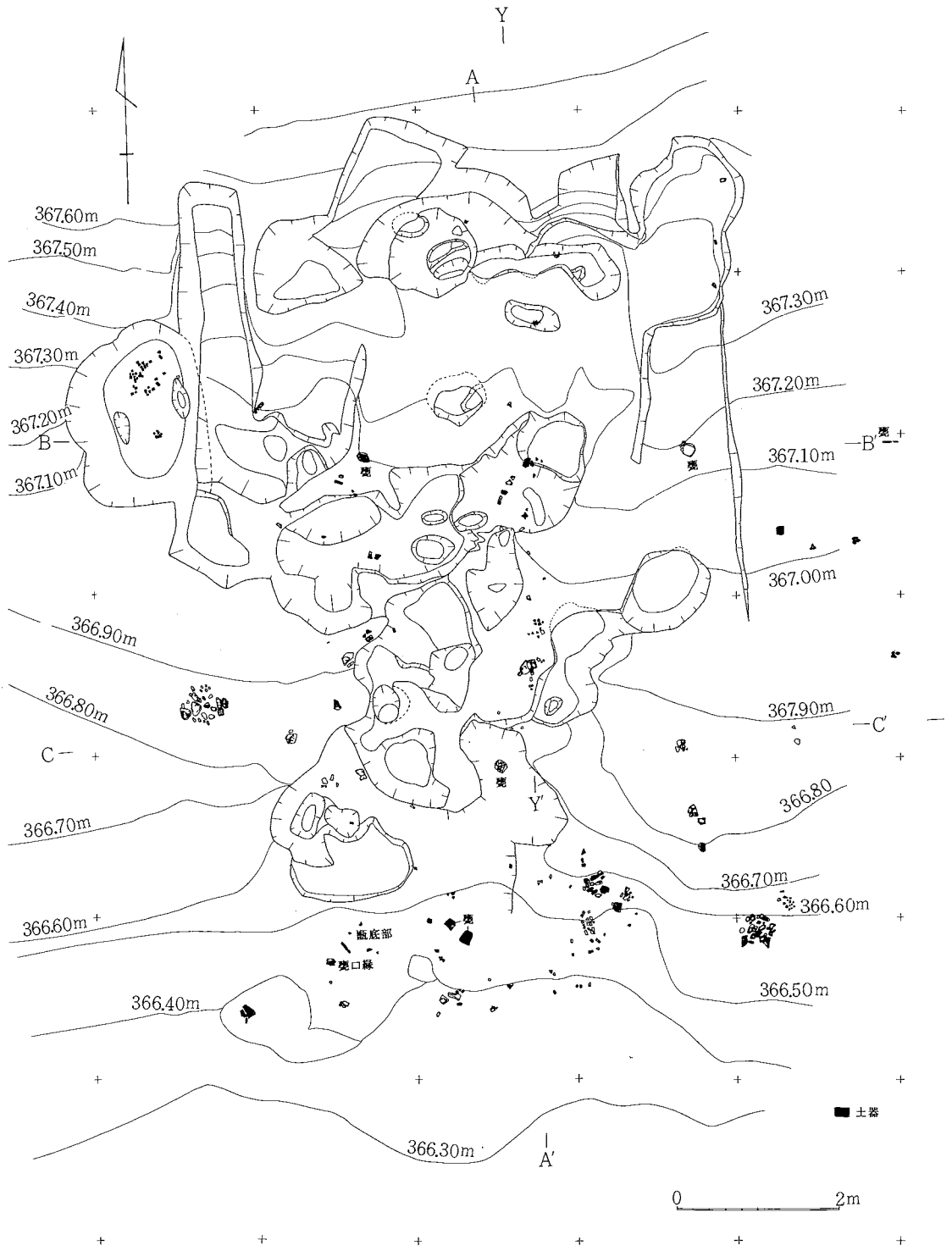
第43図 上の山遺跡遺構・遺物実測図
