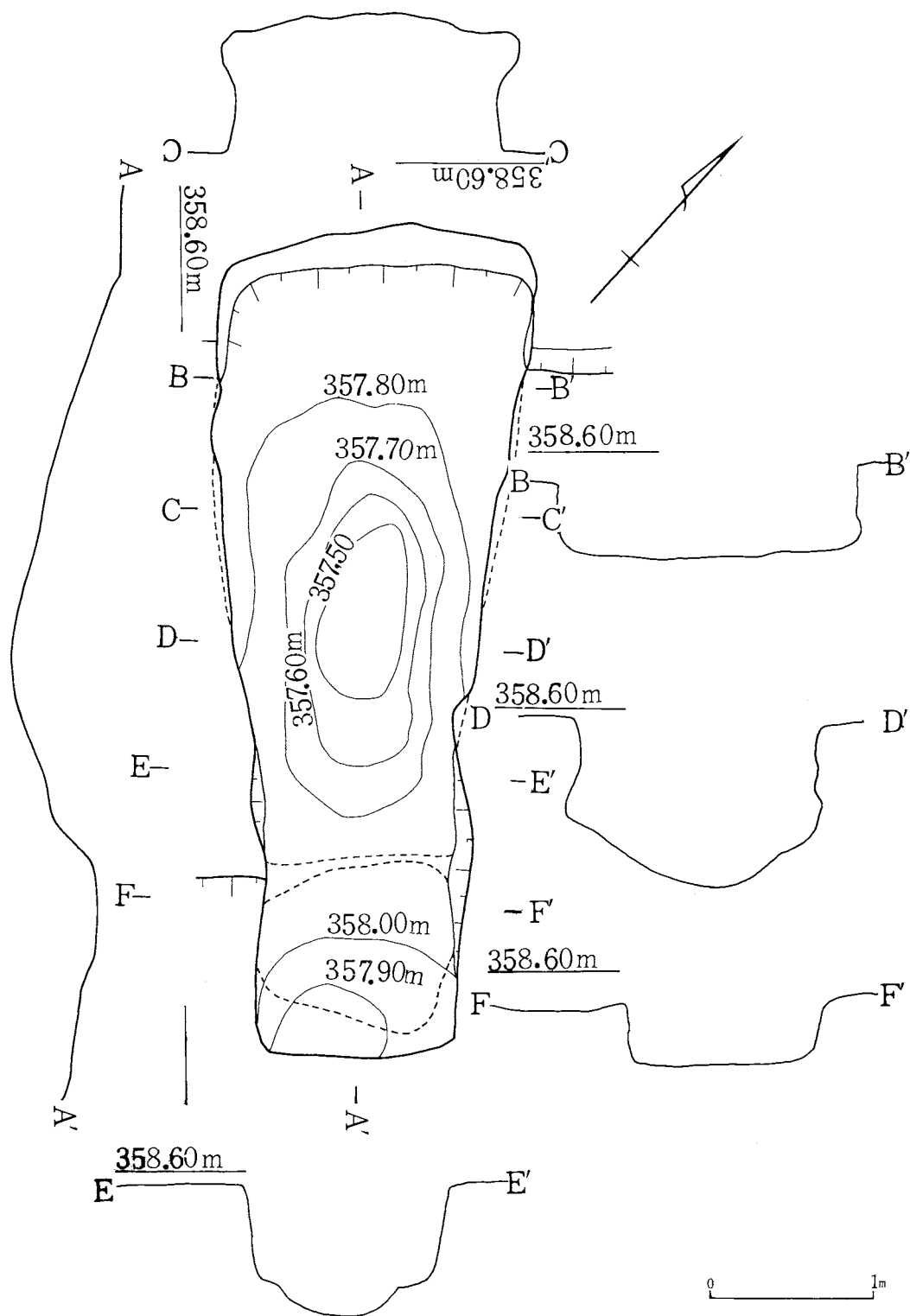
第4图 1号寨址平面·断面图
