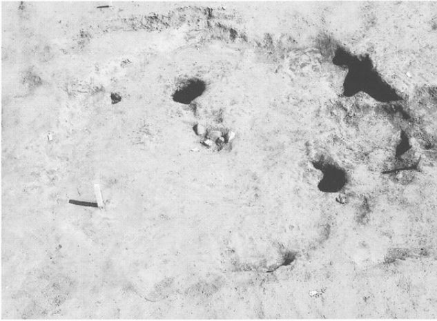
へ号住居址
