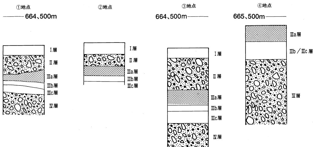
図4 土層柱状図（1：30）
