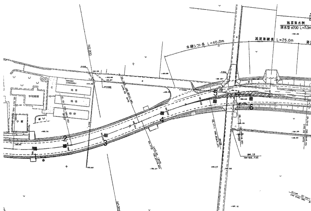
女橋遺跡トレンチ配置図
