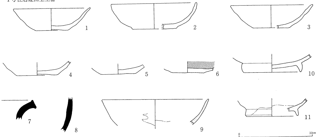
第17图 羨道部・1号住居址出土遺物
