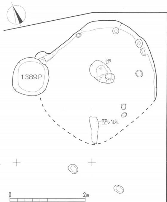
第15図 201号住居跡、1389P平面図 (1:60)
