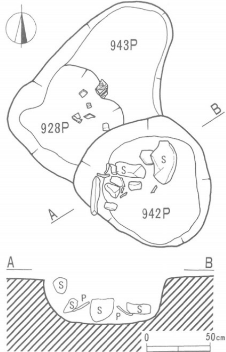
第4図 928・942・943P 平・断面図 (1:30)
