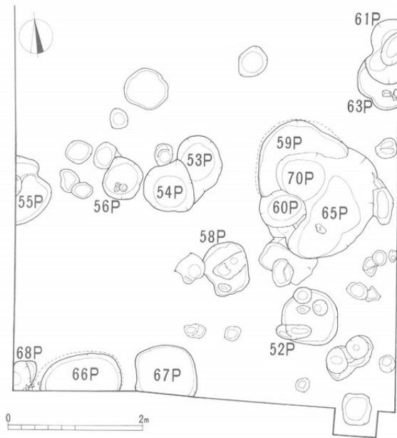
第27図 小竪穴平面図 (1:80)
