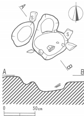
第9図 935P 平・断面図 (1:30)
