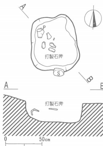
第6図 940P 平・断面図 (1:30)
