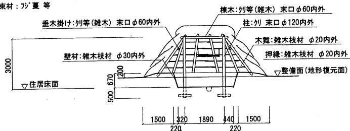
第23図 住居復元検討図
