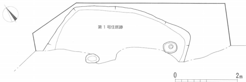
第17図 1号住居跡 平面図 (1:60)
