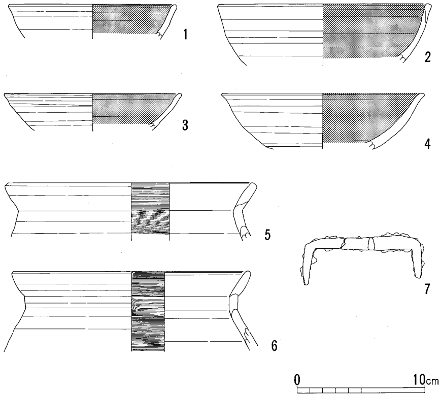
第18図 出土土器実測図 (1:3)
