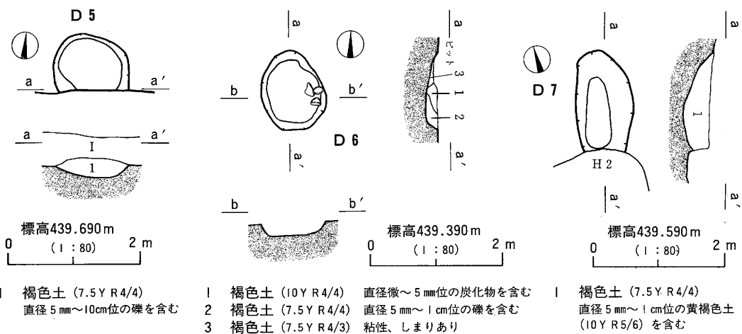
第15図 D5・6・7号土坑址実測図
