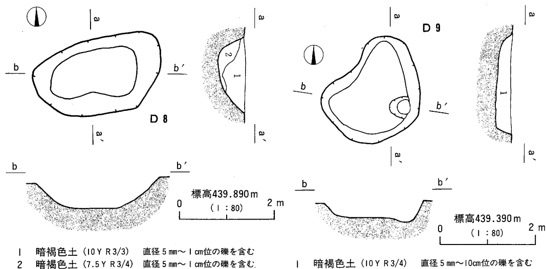
第16図 D8・9号土坑址実測図
