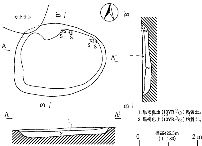
第15図 T a 1号竪穴状遺構
