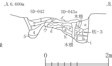
⑦4 SD-042・043aセクション
