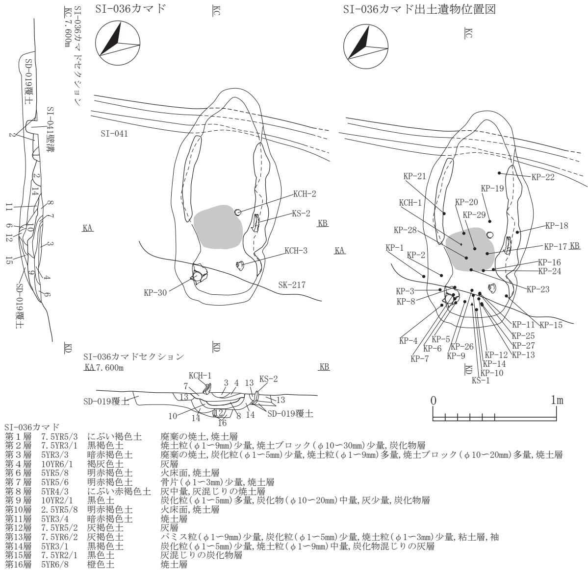
SI-036カマド焼土範囲1面目 KC
