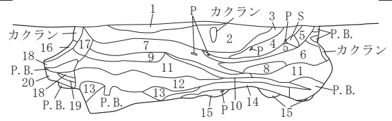
SX-016セクション
