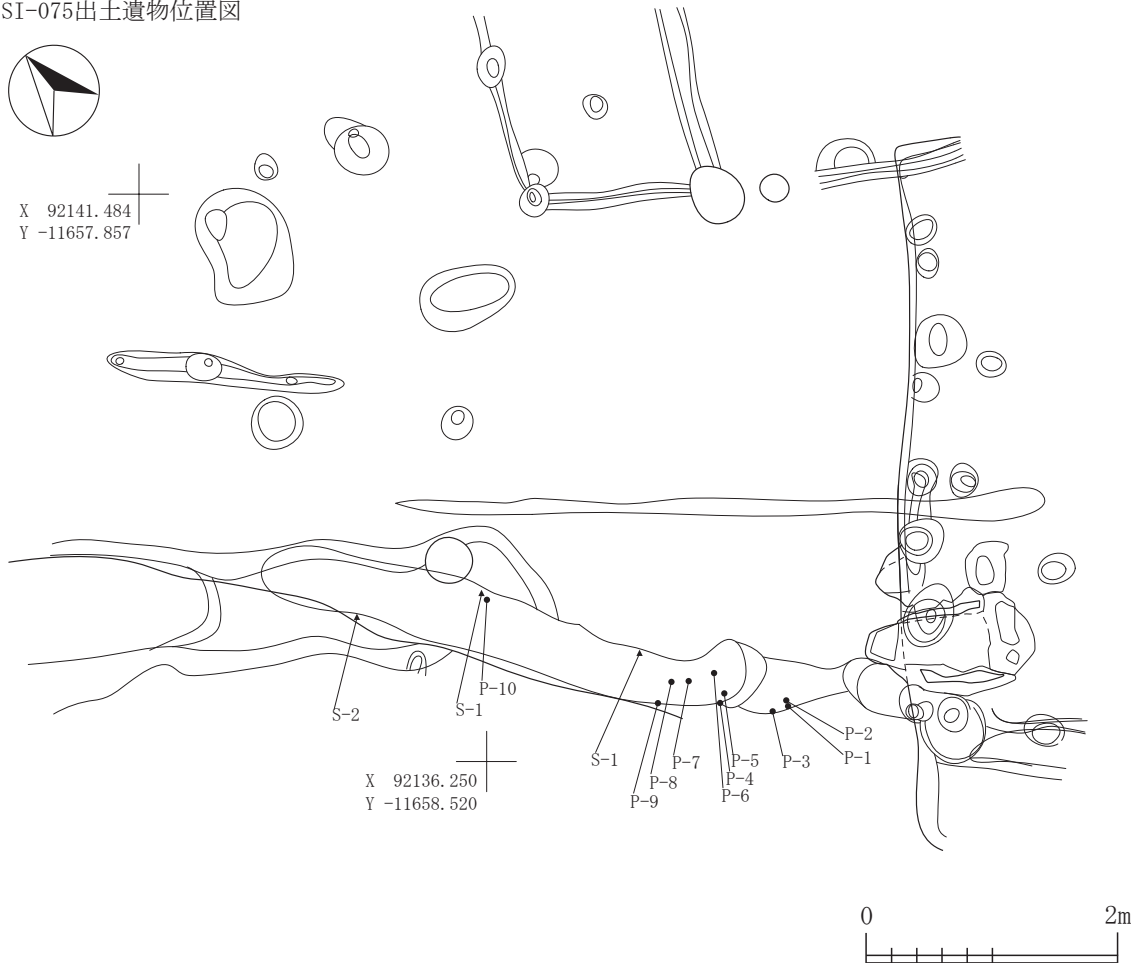
SI-075出土遺物位置図
