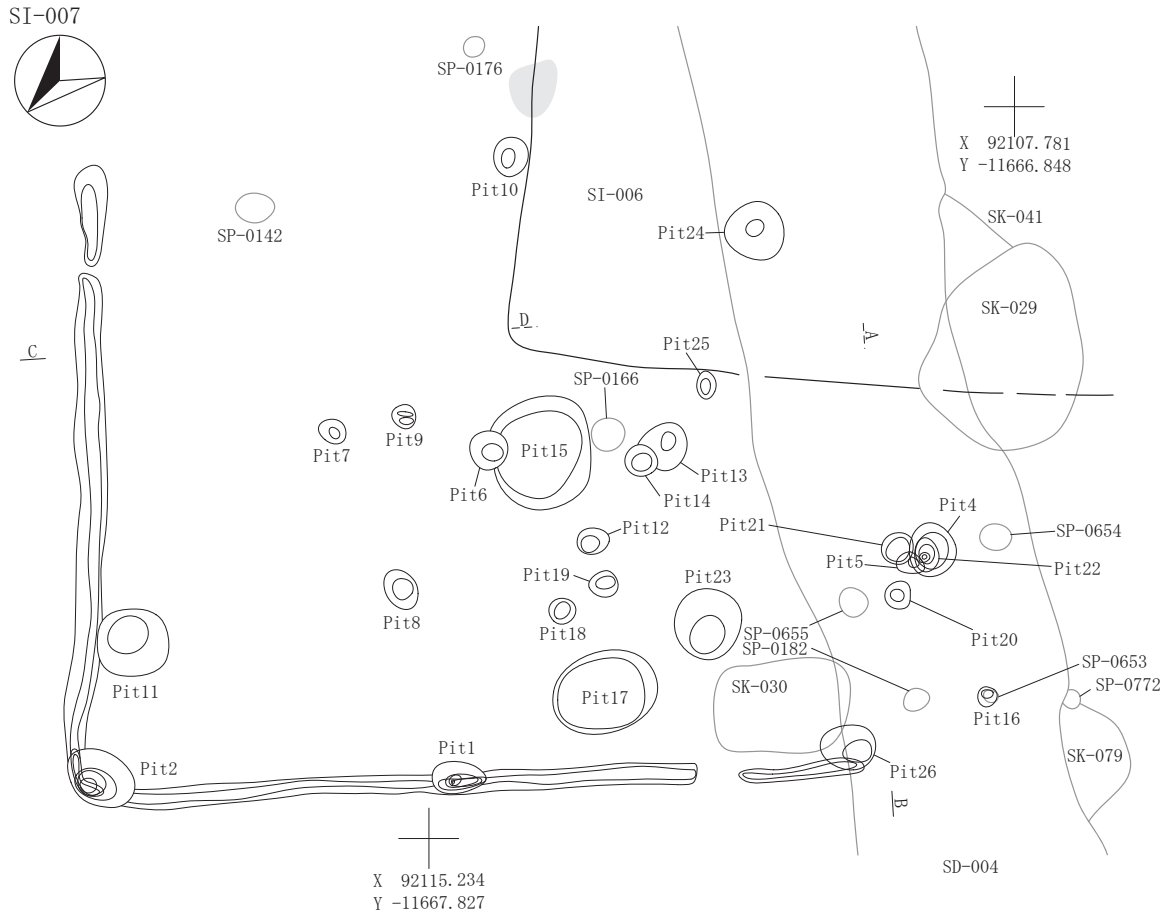
SI-006・007セクション
