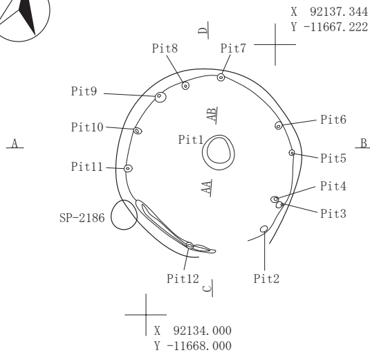
SI-073セクション・SI-073Pit1エレベーション A. 8.600m
