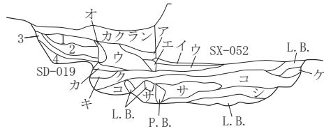
⑥⑥ SX-052・SD-019セクション A 7.700m
