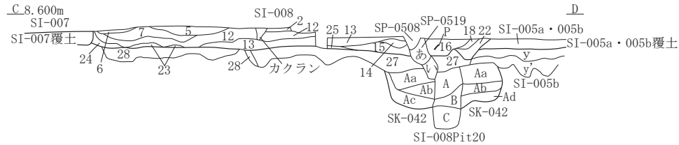
SI-005a・005b・SI-008・SI-008Pit21セクション E. 8.900m
