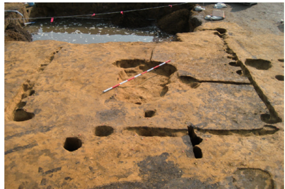
写真2-137 SI-079・080完掘(NW→)
