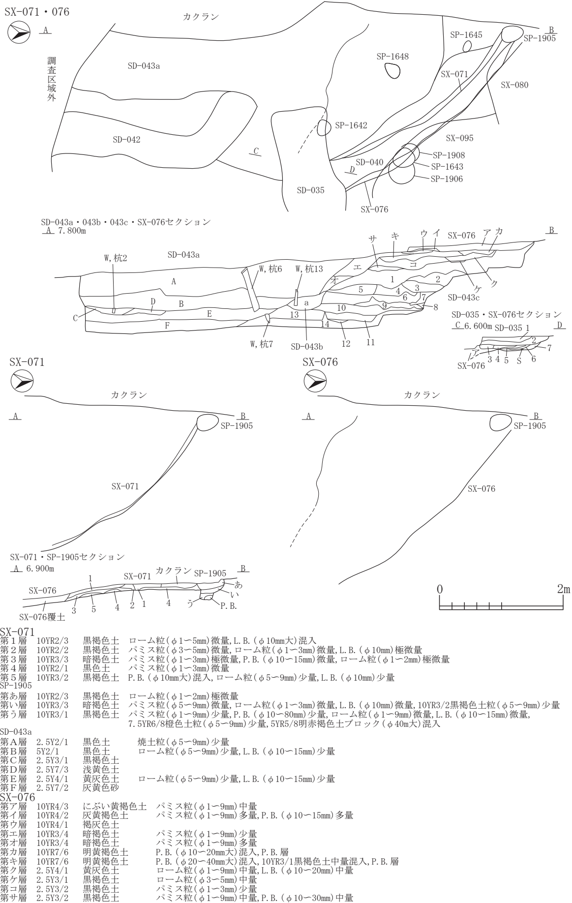
図 2-401 その他の遺構 -20
