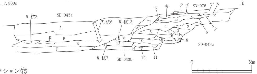
⑦⑤ SD-043a・043b・043c・SX-076セクション A. 7.800m
