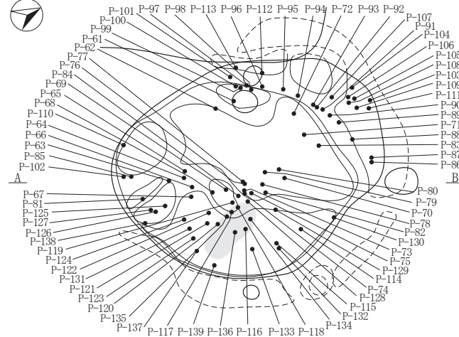
SX-016(土器)出土遺物位置図2
