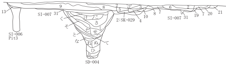
SI-006・007・SK-029・SD-004セクション・SI-006Pit3エレベーション A 8.700m
