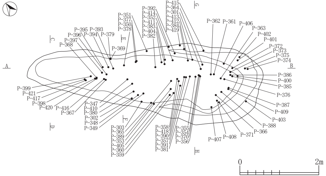
SN-002②(土器)出土遺物位置図3
