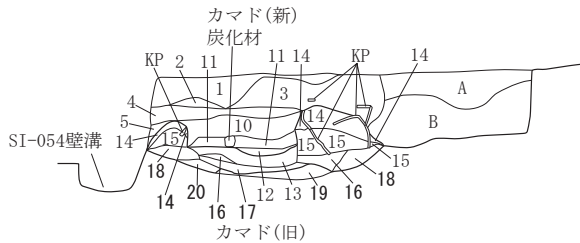
SI-059カマド新・旧南北セクション2 KC 8.800m
