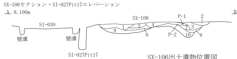
SX-106出土遺物位置図
