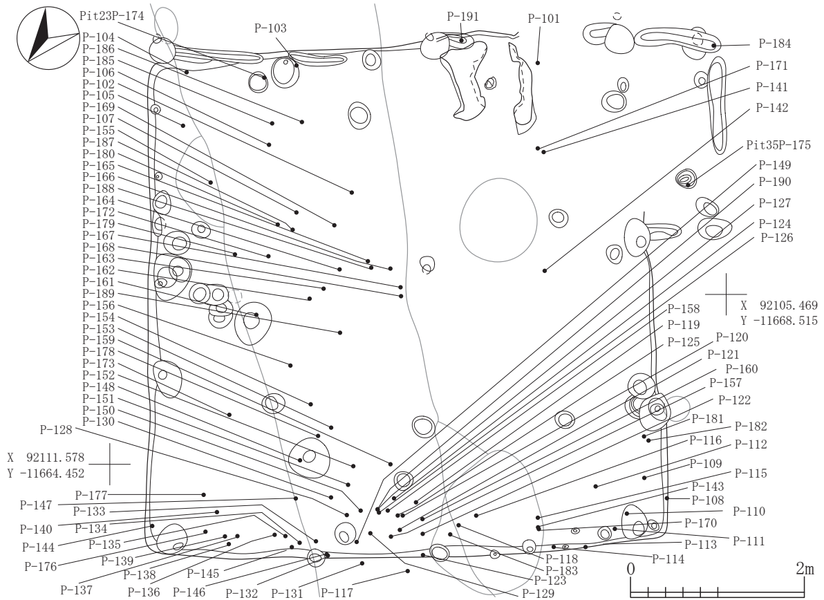
SI-006出土遺物位置图2(土器)
