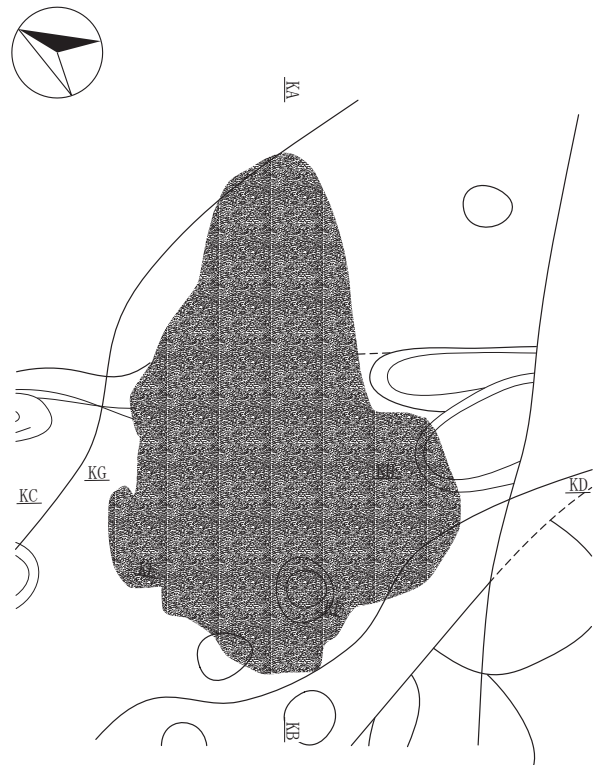
SI-032カマド粘土範囲
