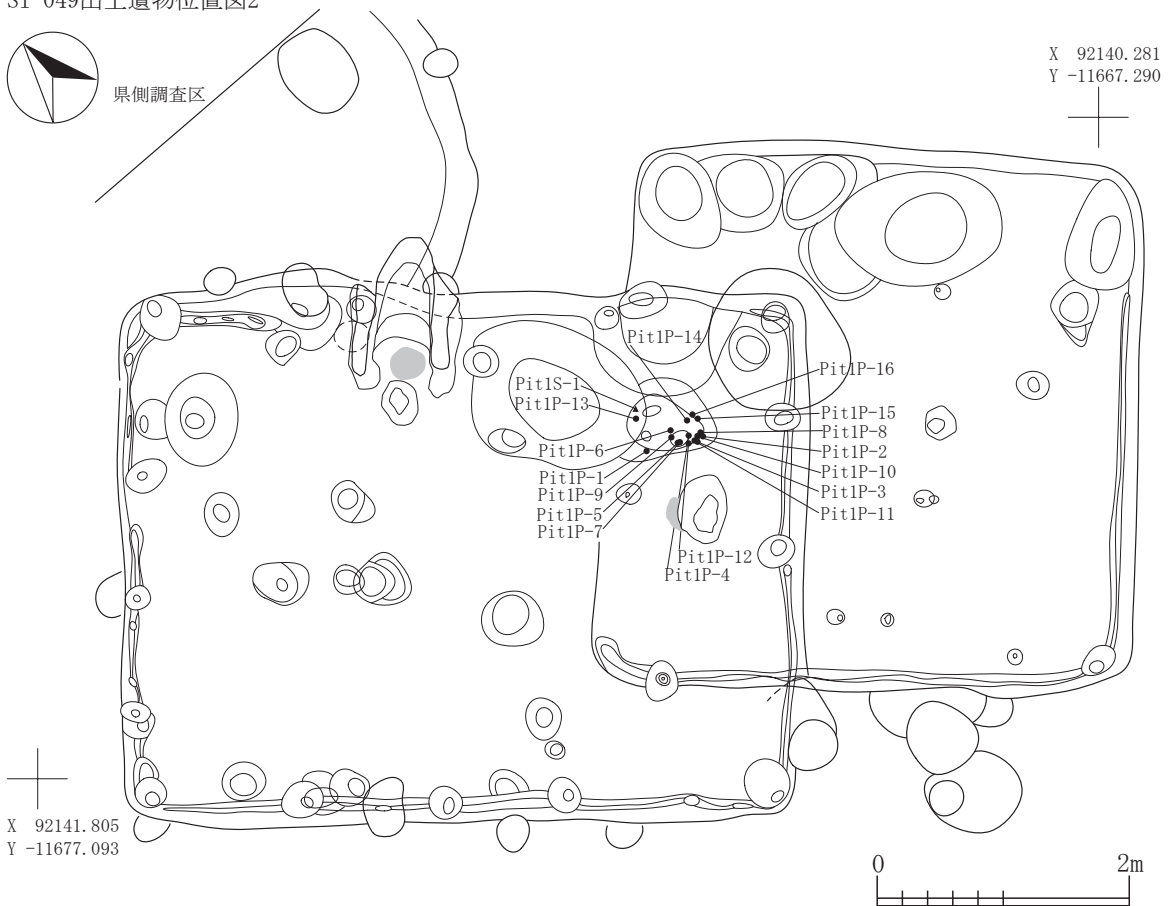
SI-049出土遺物位置図2
