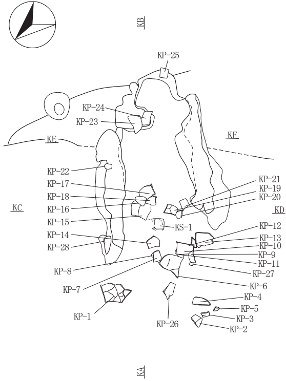
SI-010カマド出土遺物位置図
