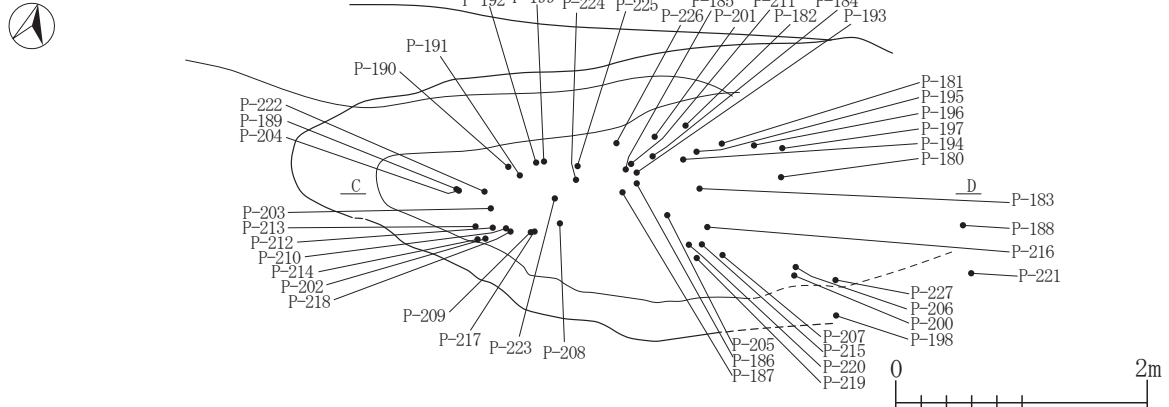
SN-011(土器)出土遺物位置図4
