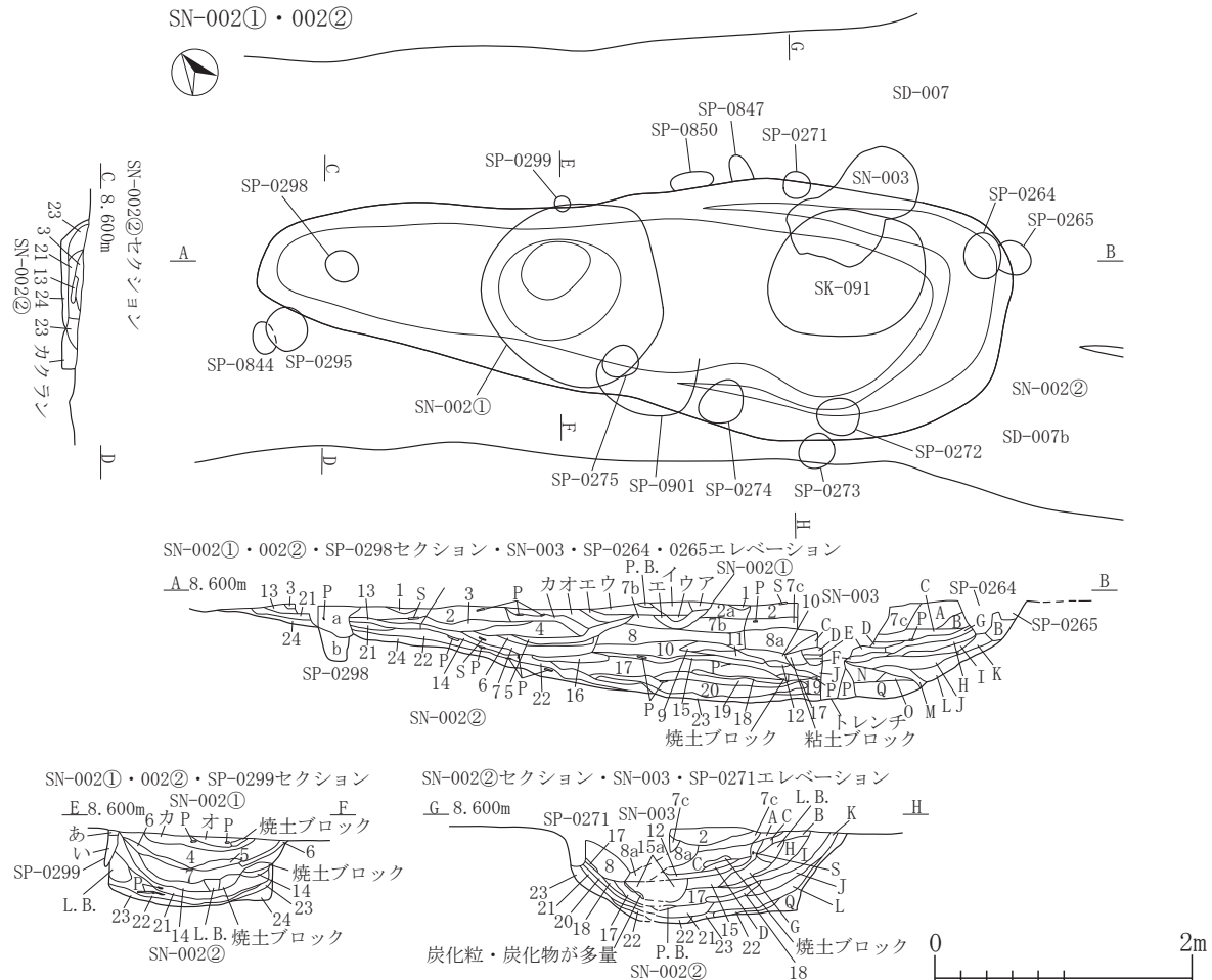
図 2-350 焼成関連遺構 -1
