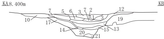
SI-060カマド2セクション
