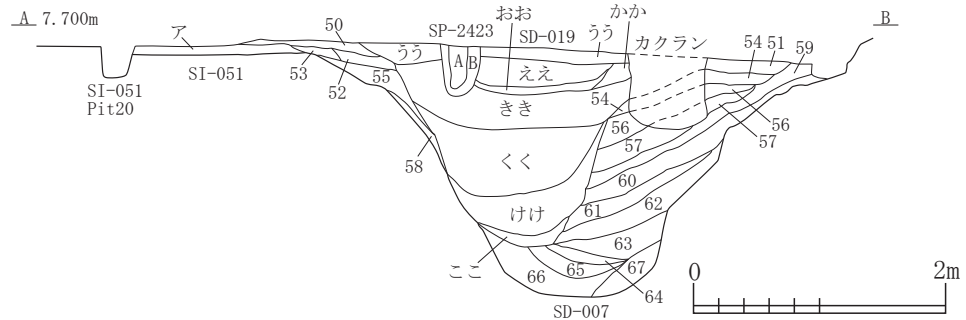
SI-051・SD-007・019・SP-2423セクション・SI-051Pit20エレベーション
