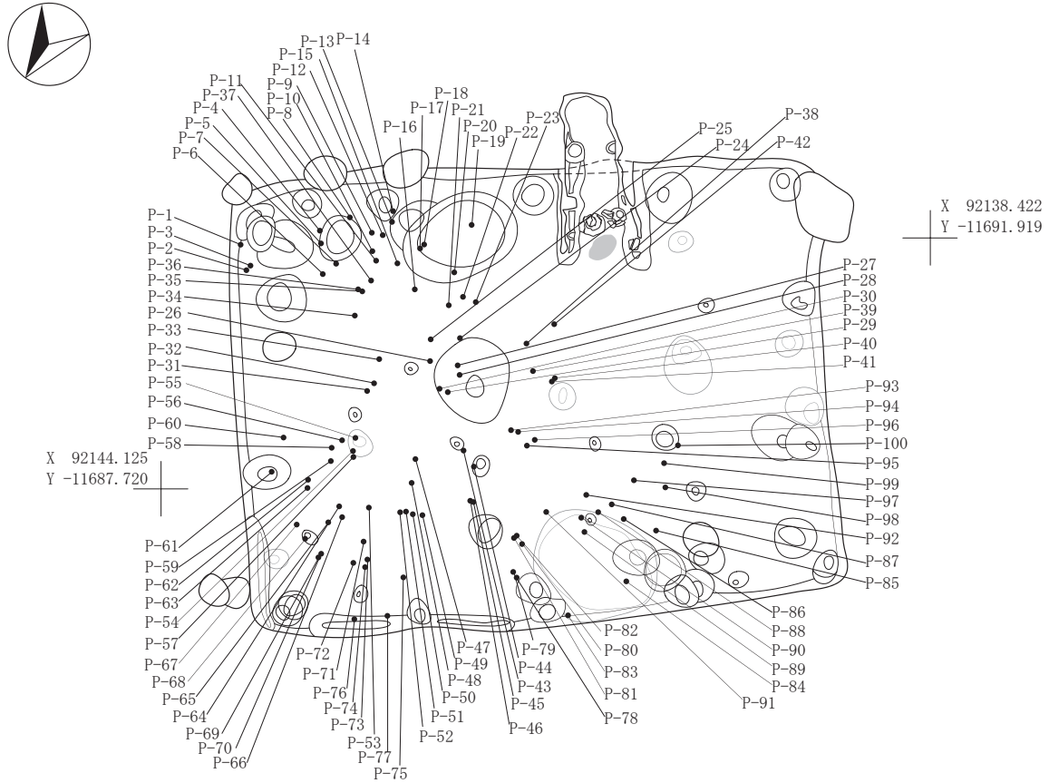
SI-023出土遺物位置図2
