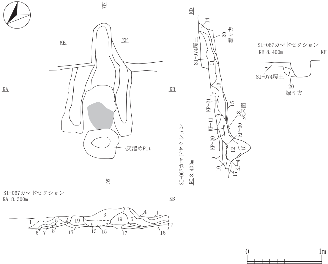
SI-067カマド平面
