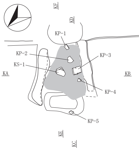
SI-008カマド焼土・出土遺物位置図1
