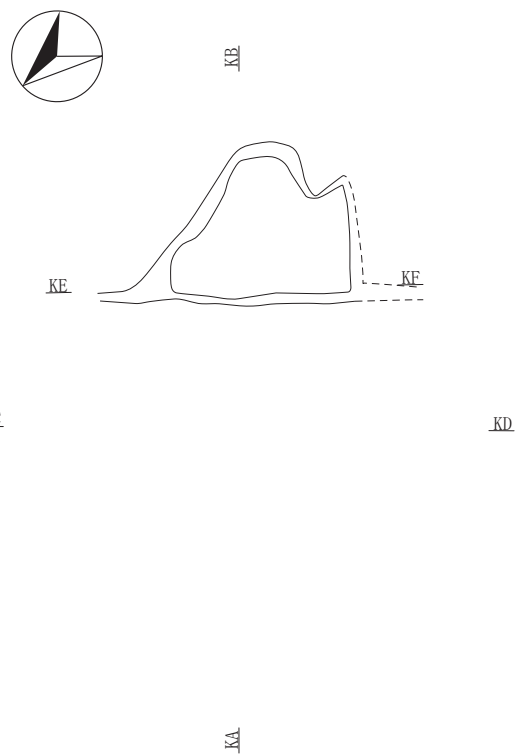
SI-010カマド掘り方
