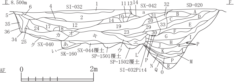
SI-032・032Pit4・SK-160・SX-040・042・SD-020セクション
