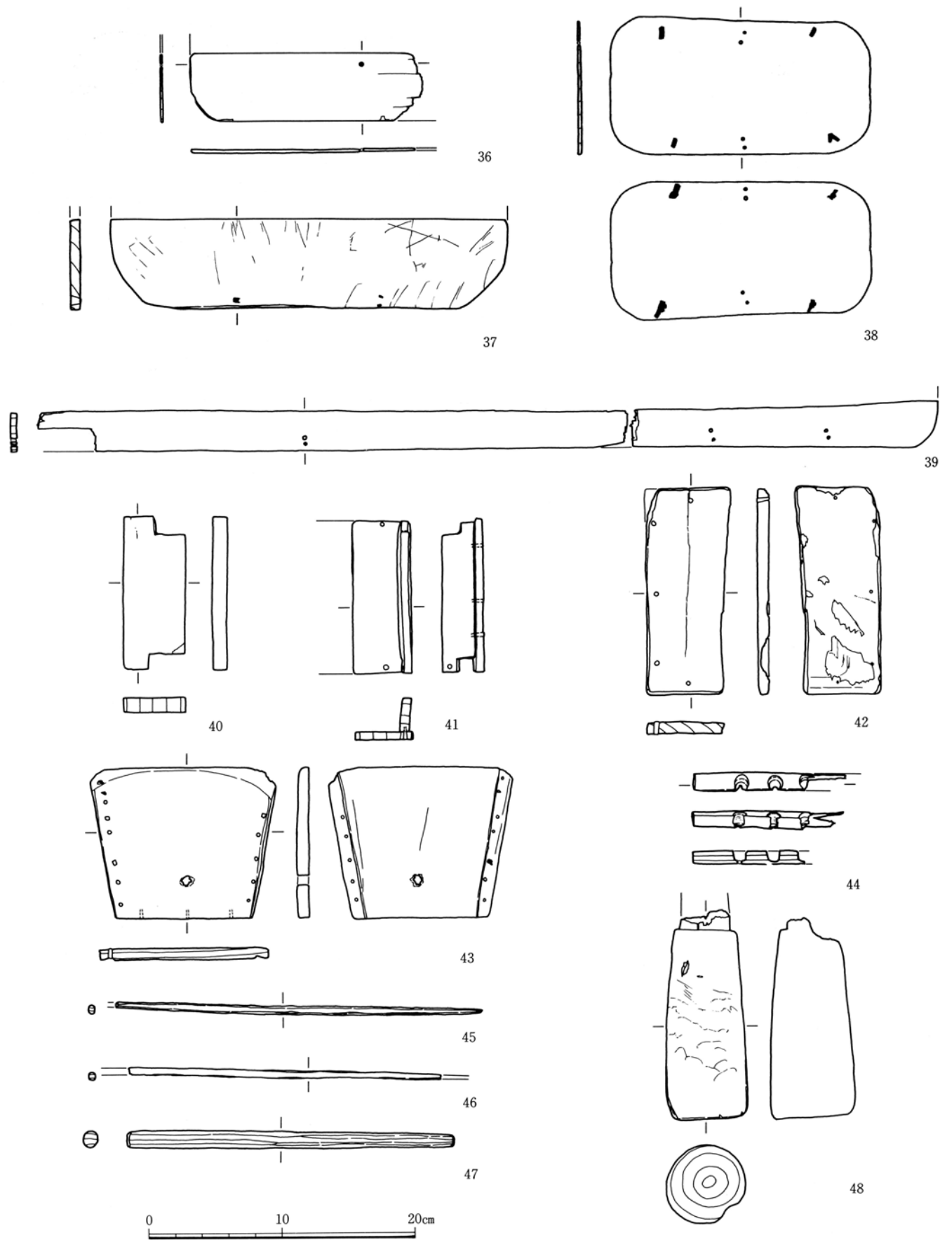
第48図 遺物実測図 (22) (木製品)
