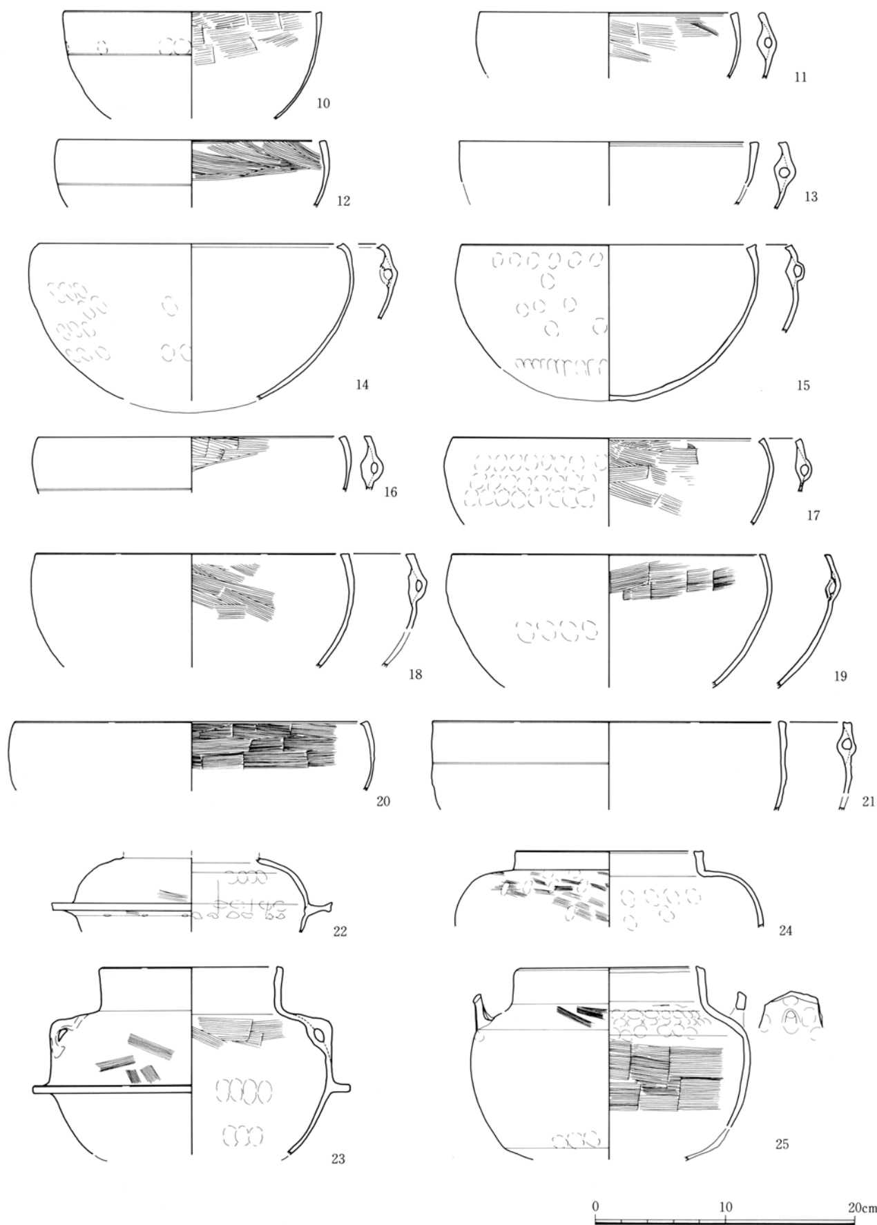
第37図 遺物実測図 (11) (SD01土師器鍋・釜)
