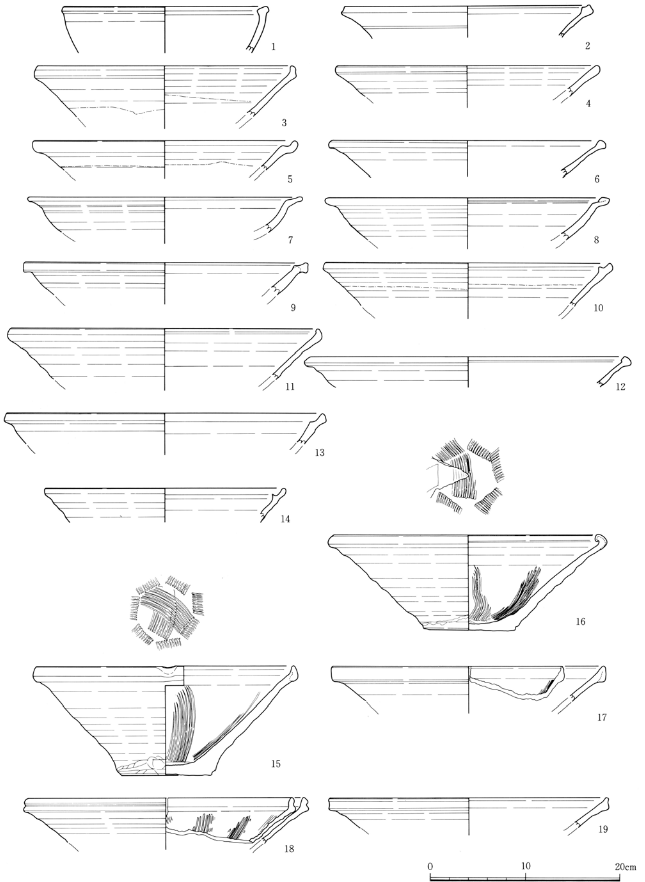
第20図 遺物実測図(3) (SD01瀬戸美濃窯産陶器平鉢・大皿・擂鉢)
