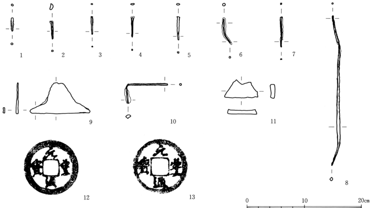
第51図 遺物実測図 (25) (金属製品) (12・13はS = 1 : 1)
