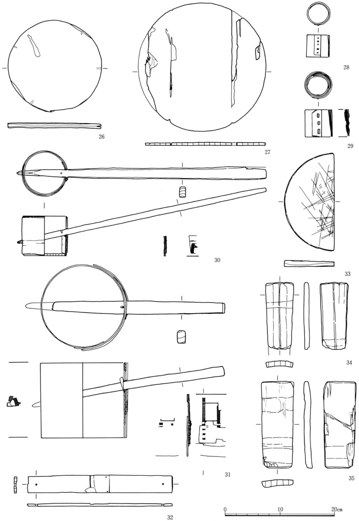
第47図 遺物実測図 (21) (木製品)
