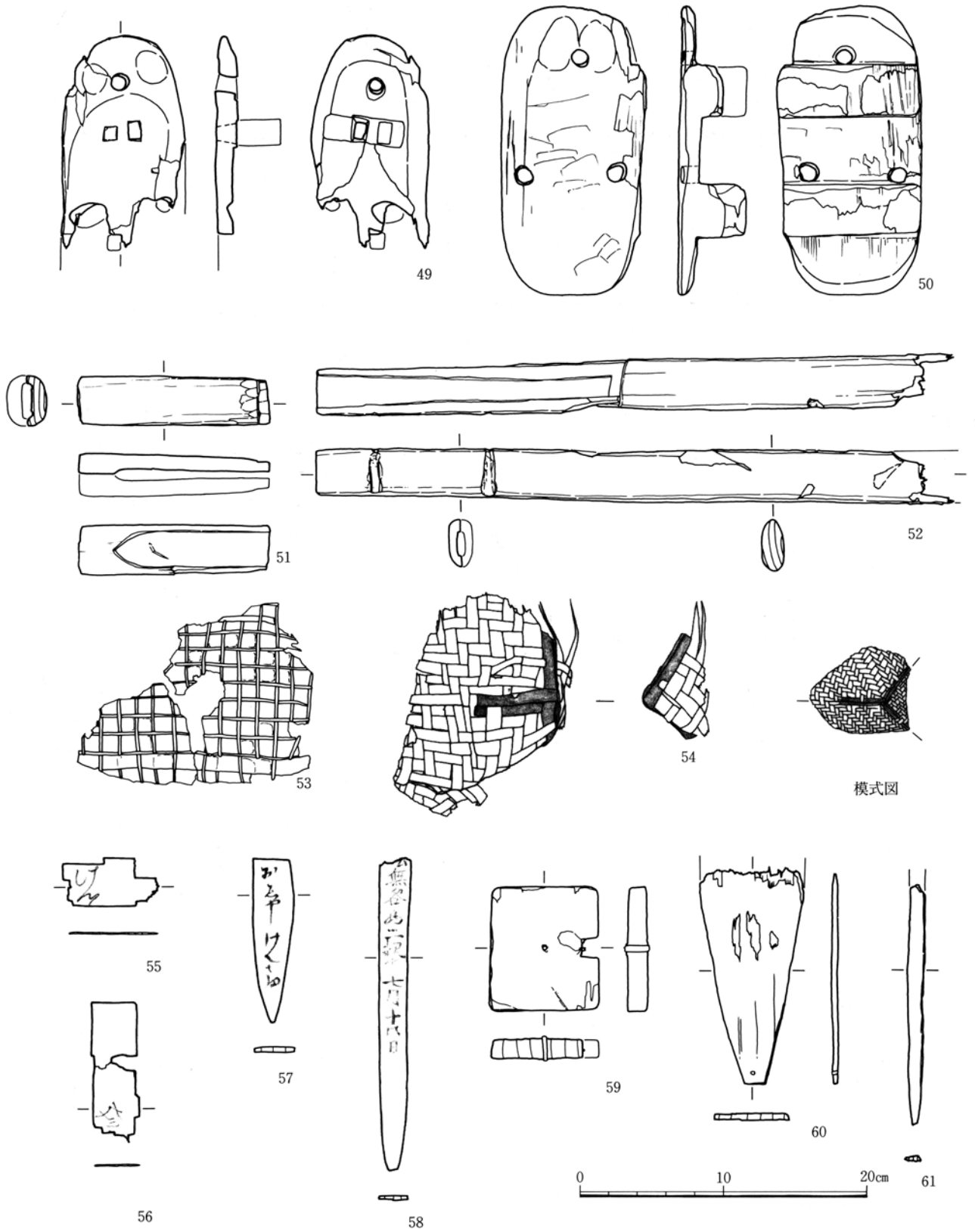
第49図 遺物実測図 (23) (木製品)
