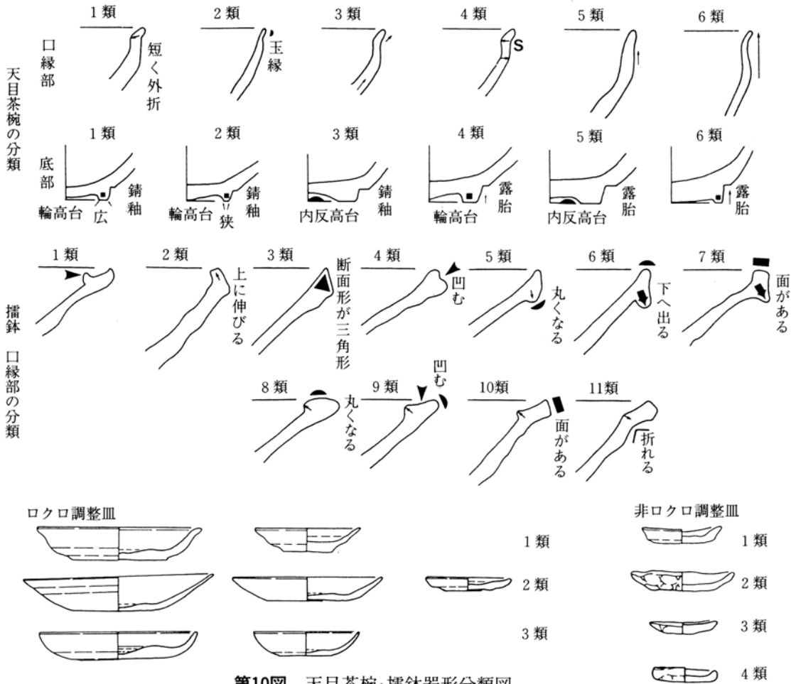
第10図 天目茶碗・搦鉢器形分類図
