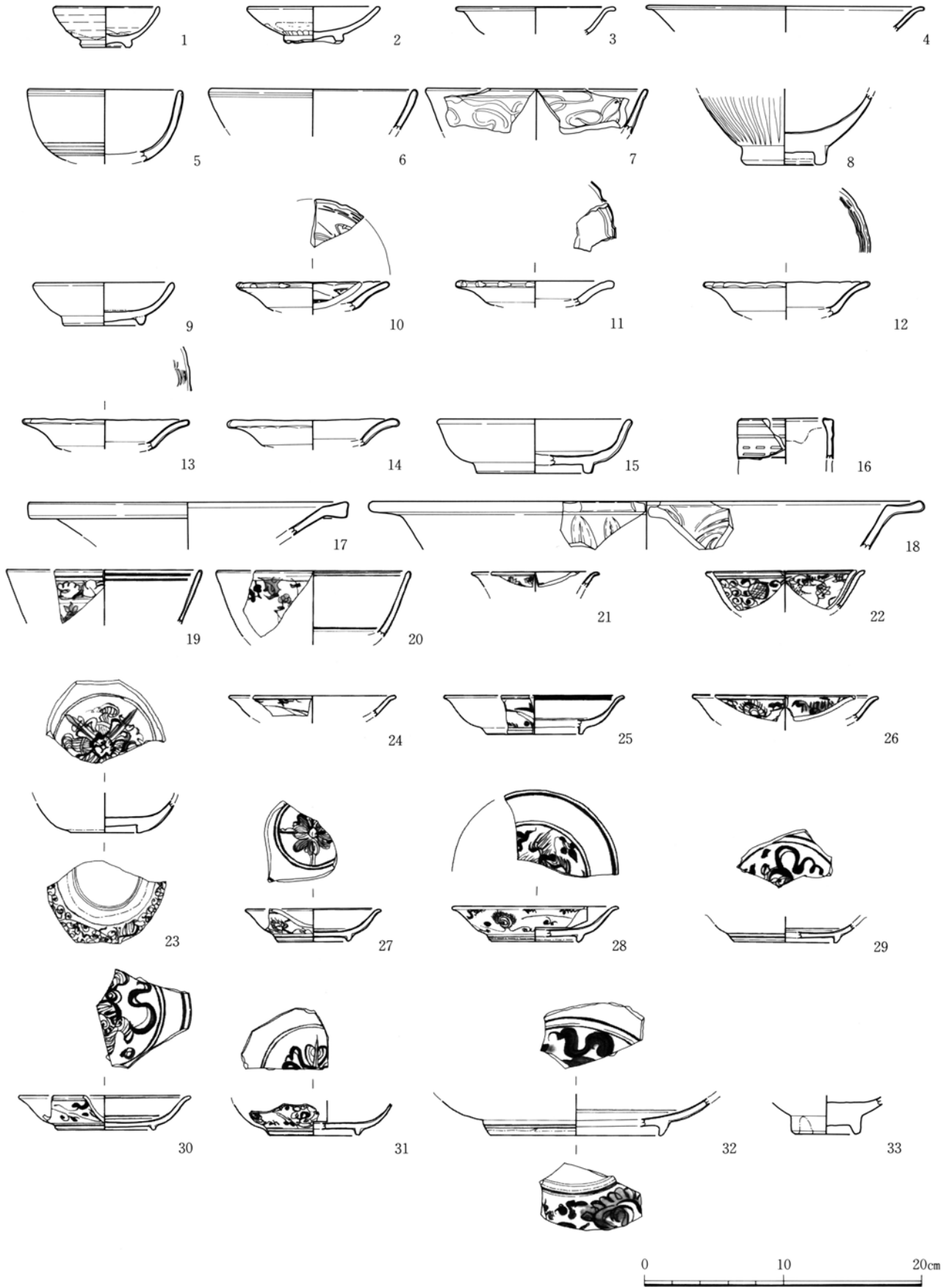
第39図 遺物実測図 (13) (SD01中国窯産陶磁器・その他)
