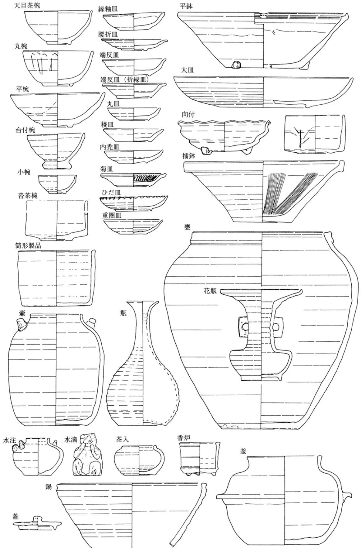
第9図 瀬戸美濃窯産陶器器種分類図
