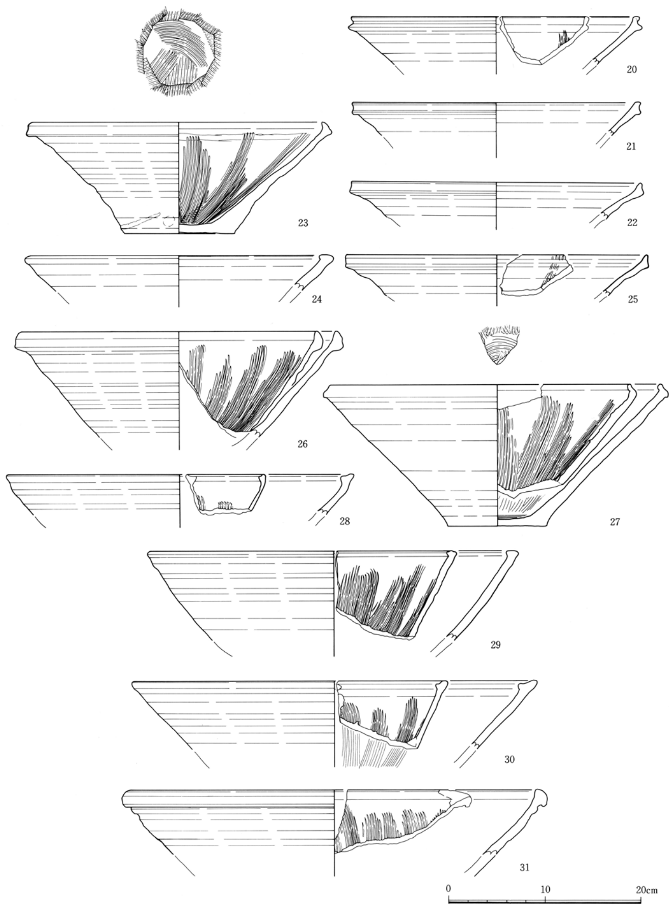
第21図 遺物実測図(4) (SD01瀬戸美濃窯産陶器搦鉢)
