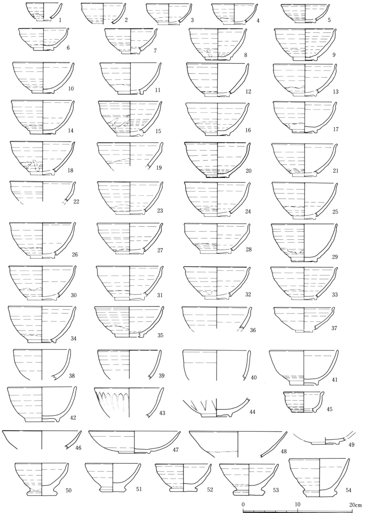
第16図 遺物実測図(1) (SD01瀬戸美濃窯産陶器碗)
