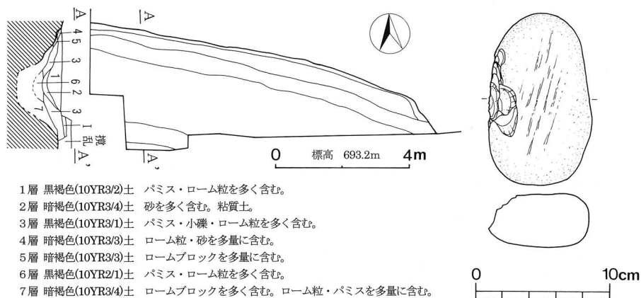
第4図 M2号溝址 (1:160) とその遺物 (1:4)
