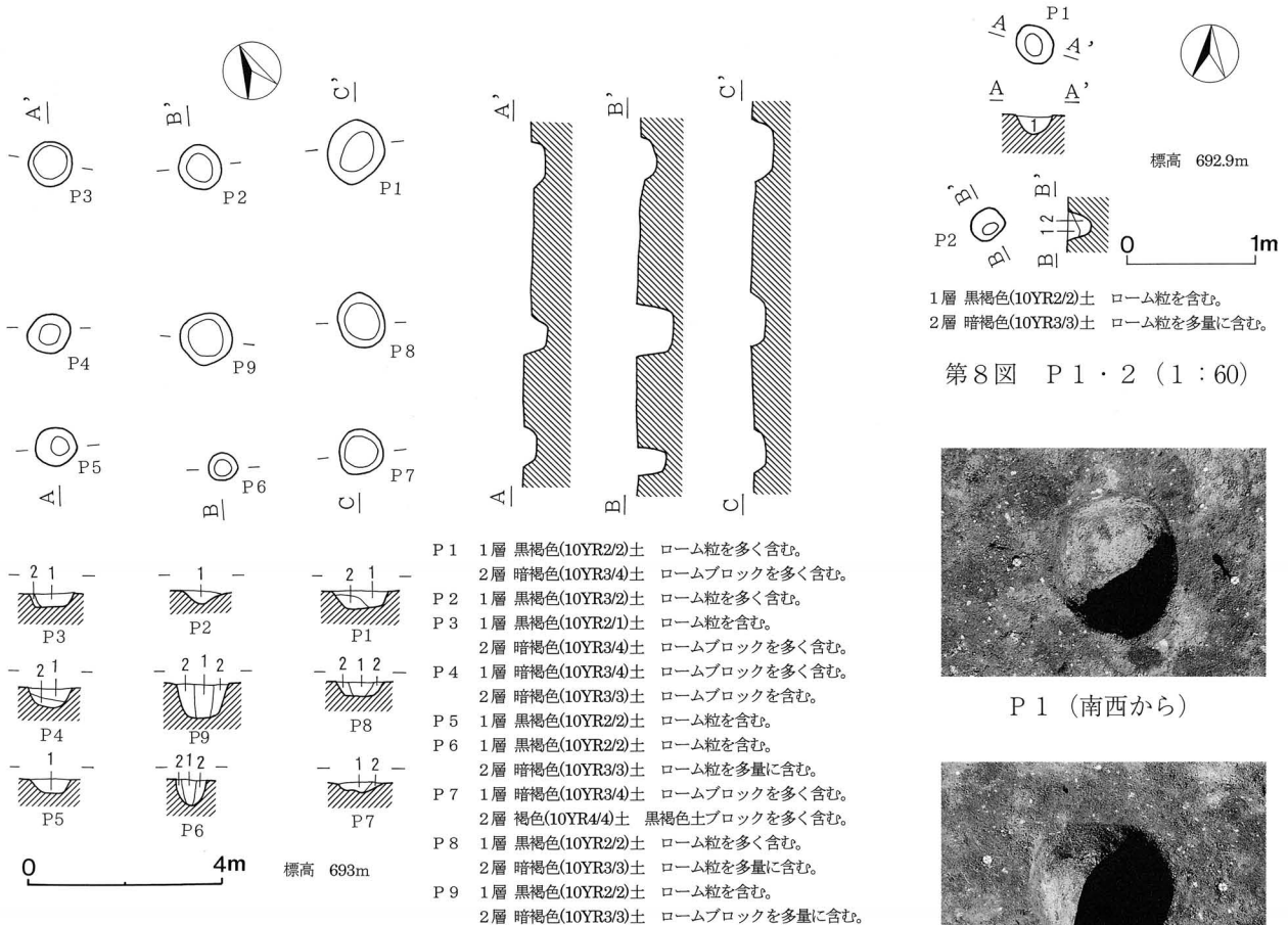
第7図 F1号掘立柱建物址 (1:80)
