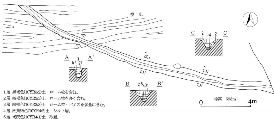
第3図 M1号溝址 (1:160)
