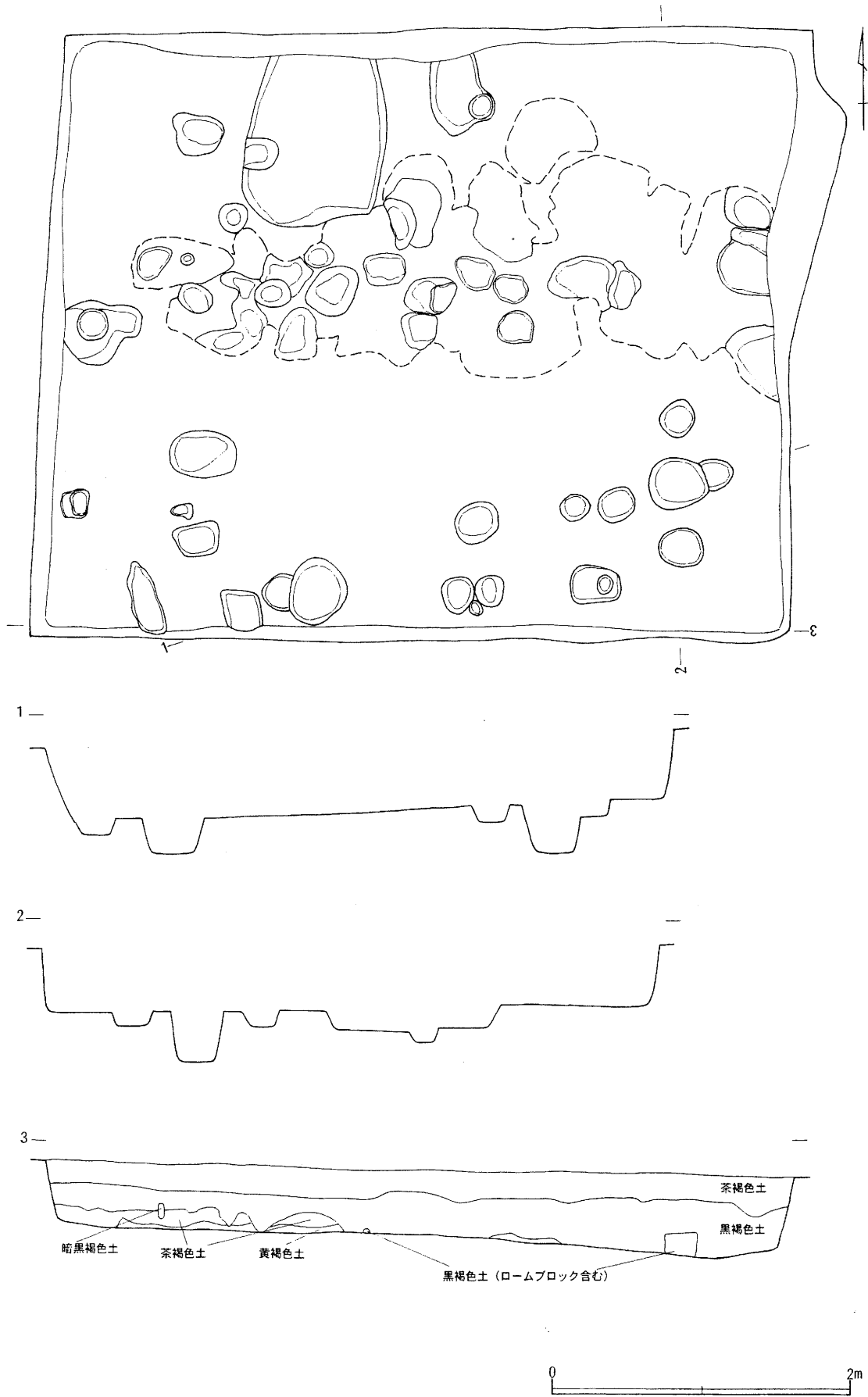
図4 調査区違構分布図 (1:40)
