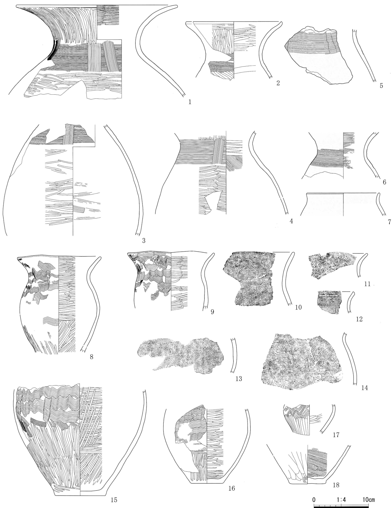
第 11 图 H2 号住居址遺物实测图
