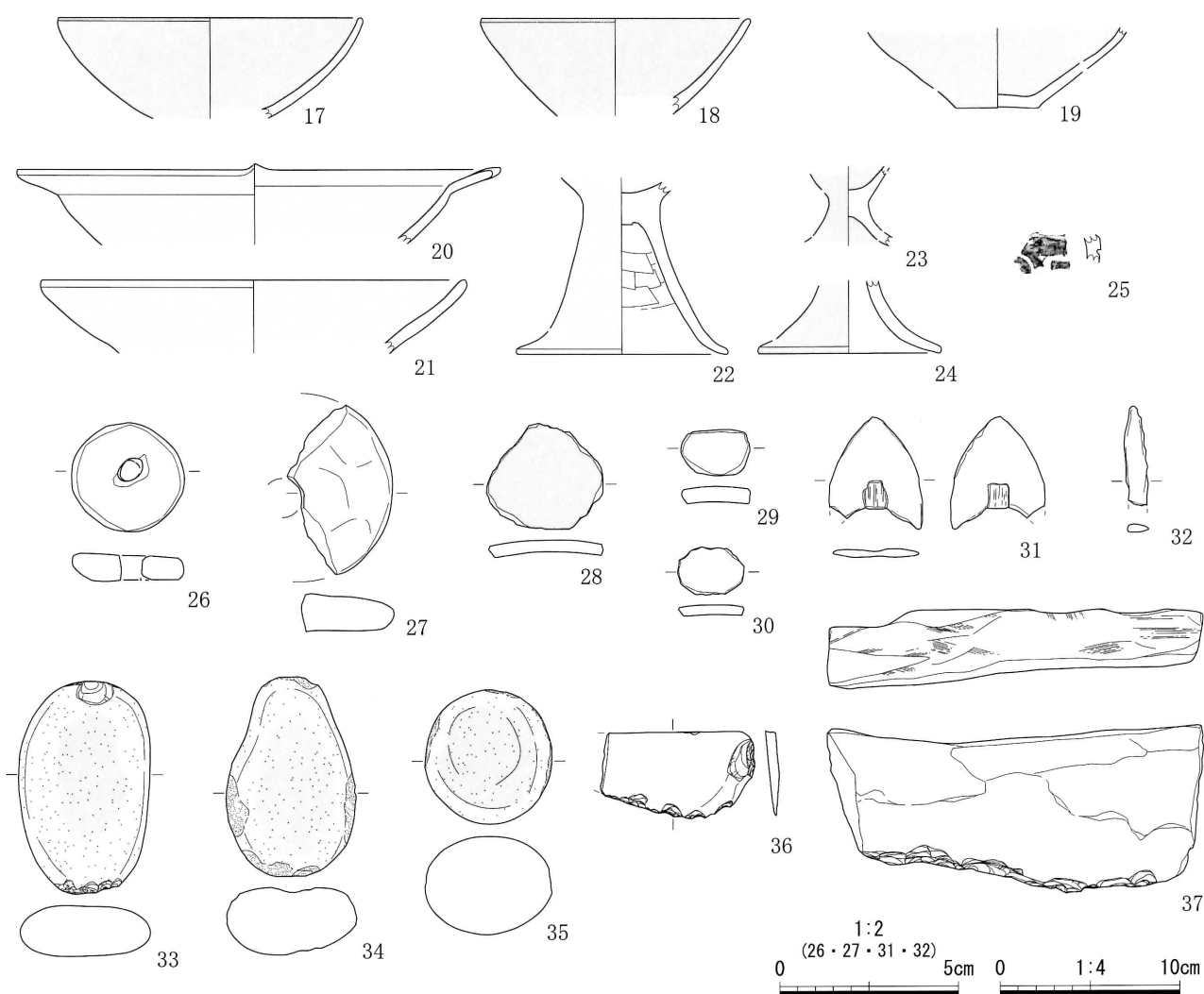
第9図 H1号住居址遺物実測図(2)
