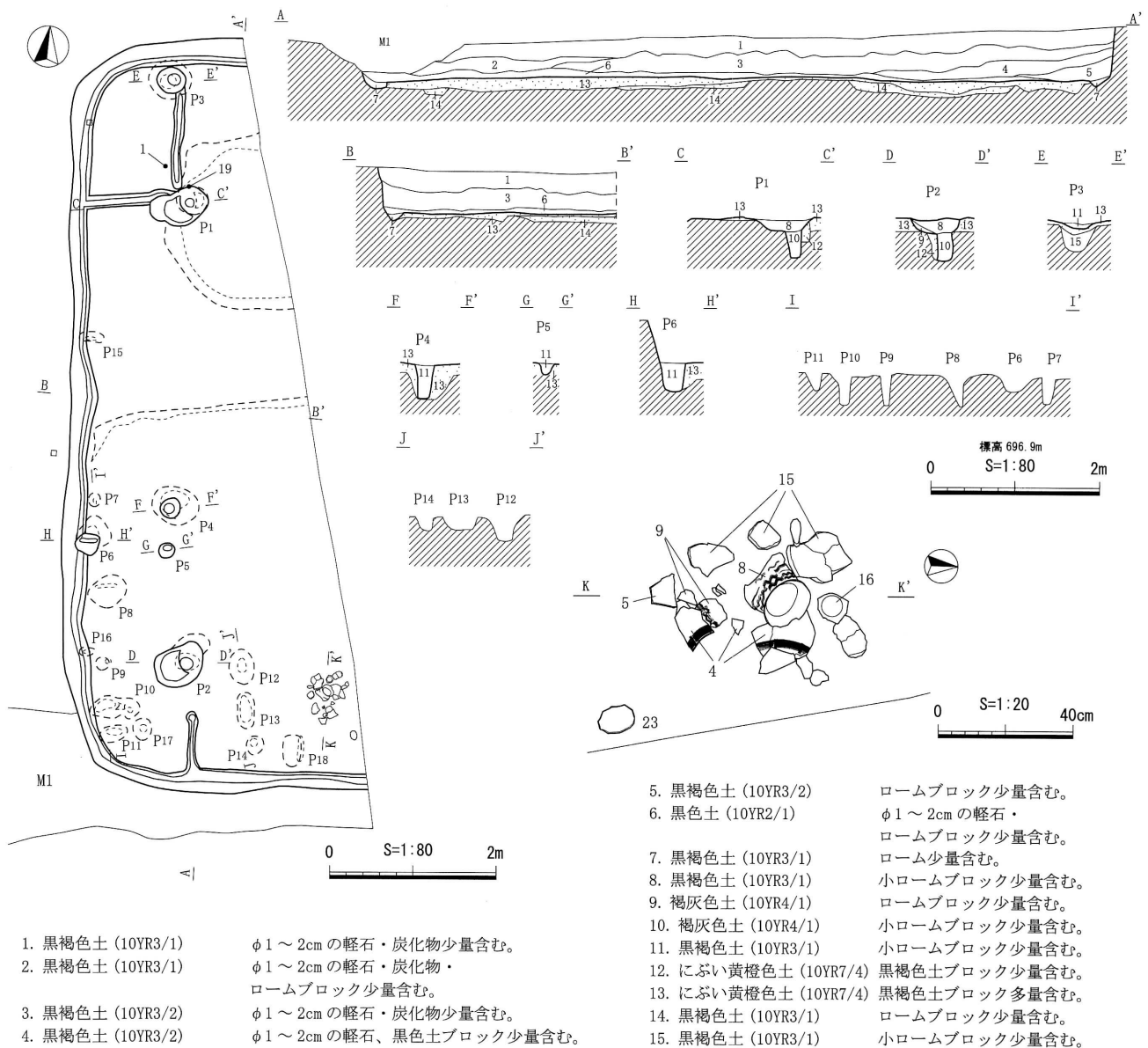
第10図 H2号住居址遺構実測図
