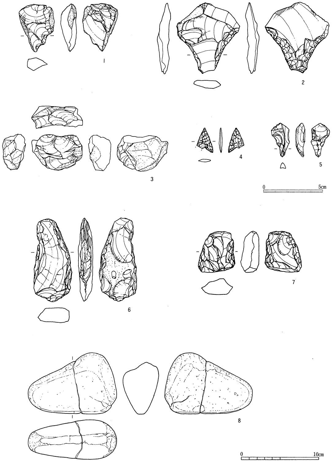
第3図 石器実測図 (1~5=1:2、6~8=1:3)
