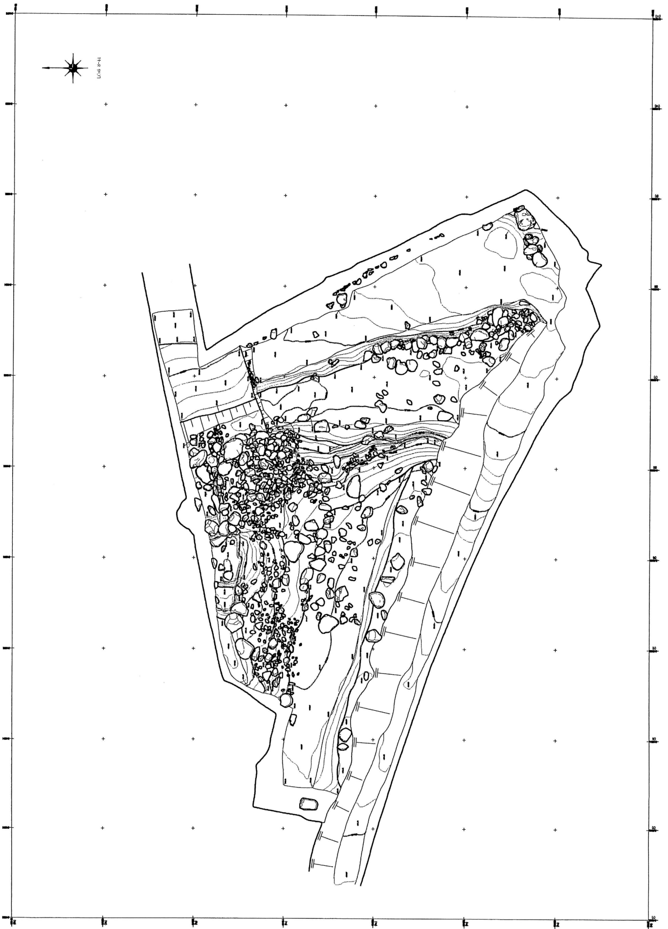
第 21 图 堀切1 平面图
