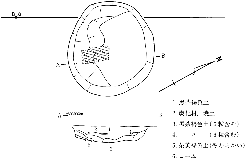
第5図 土坑1実測図 (S = 1 : 40)
