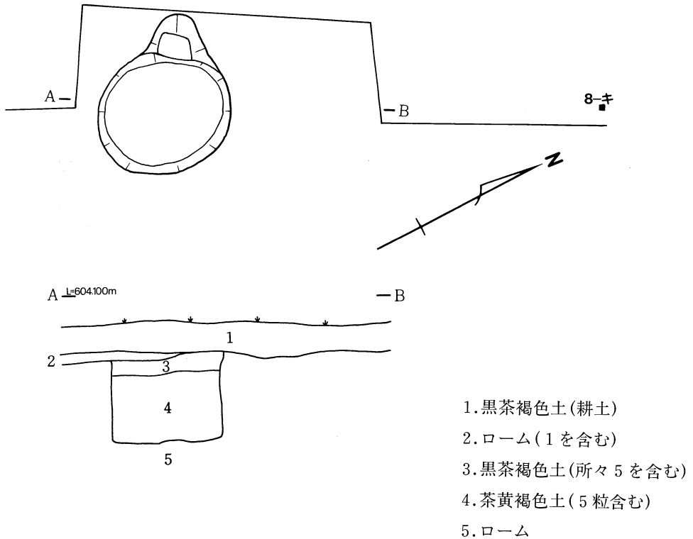
第6図 竪穴1実測図 (S = 1 : 40)
