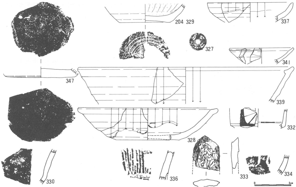
第9図 北の堀及び周辺出土遺物実測図 (S = \frac{1}{3} )
