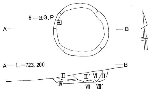
第11図 第1号土壇実測図(S = \frac{1}{60} )
