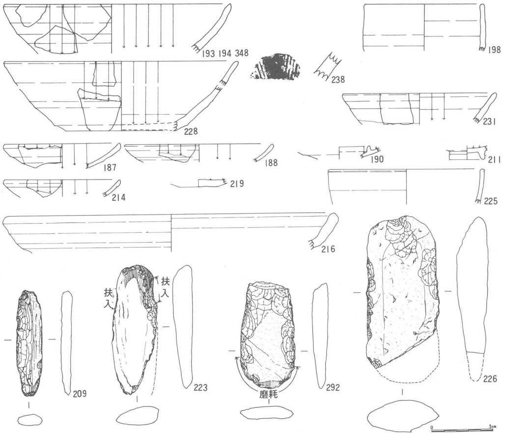
第13図 北の堀及び南の堀周辺出土遺物実測図 (S = \frac{1}{3} )
