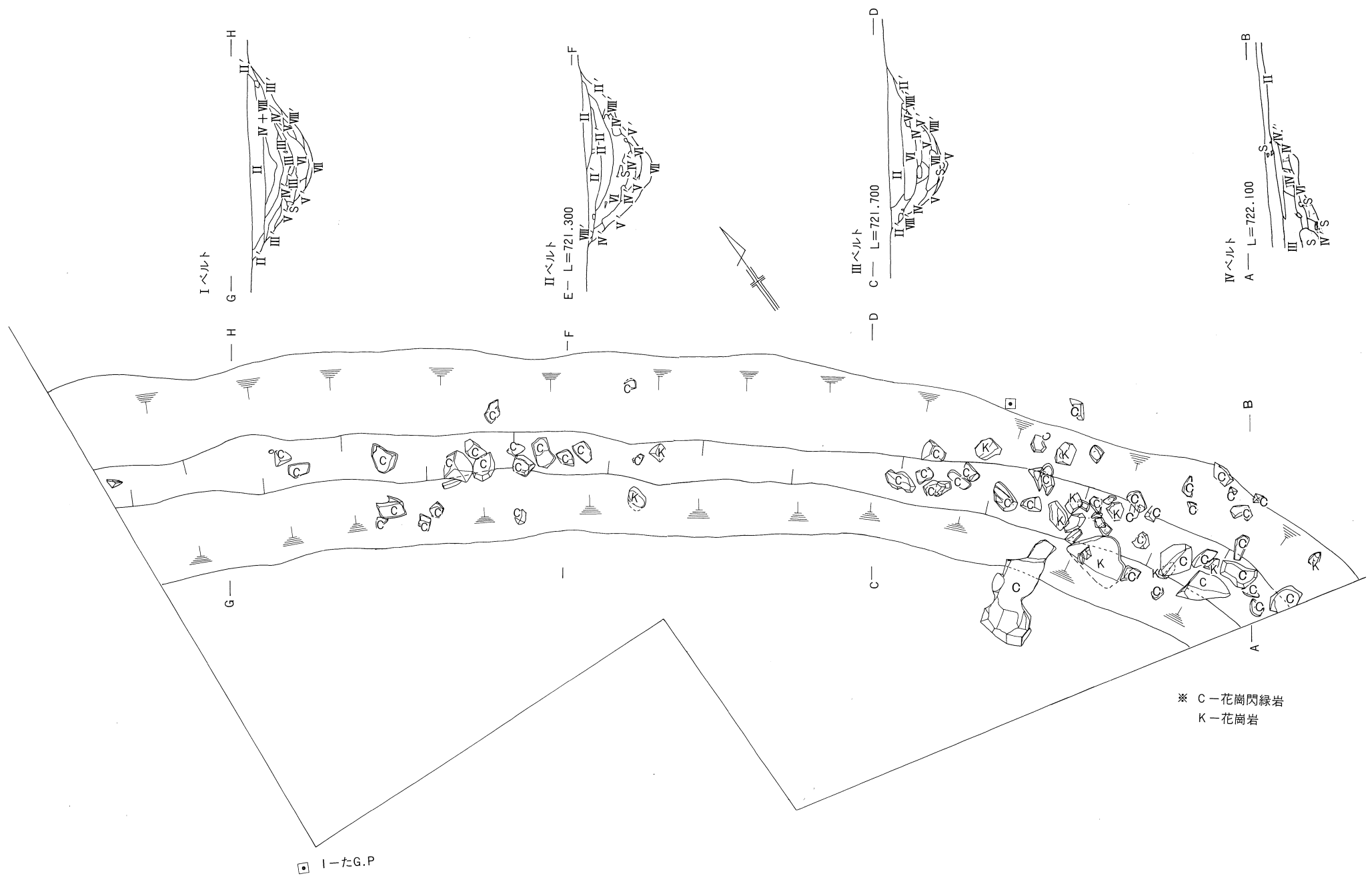
第10図 南の堀実測図 (S = \frac{1}{60} )
