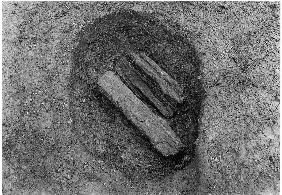
3. Pit-203 上位礎板 検出状況 (北西から)
