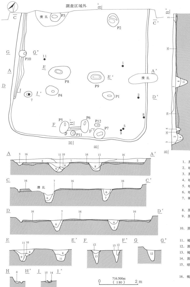
H 2 号住居址実測図
