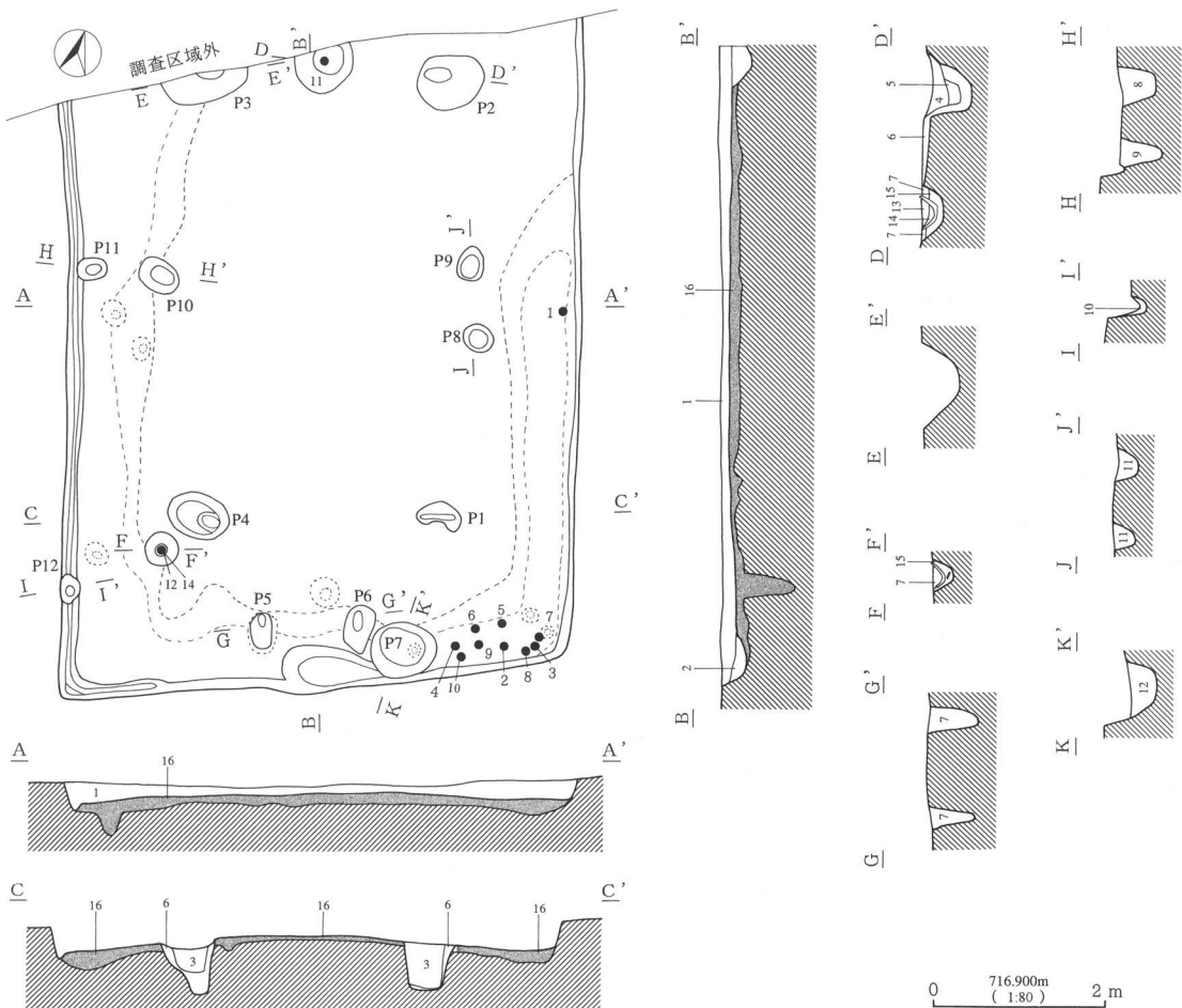
H 1 号住居址実測図(1)
