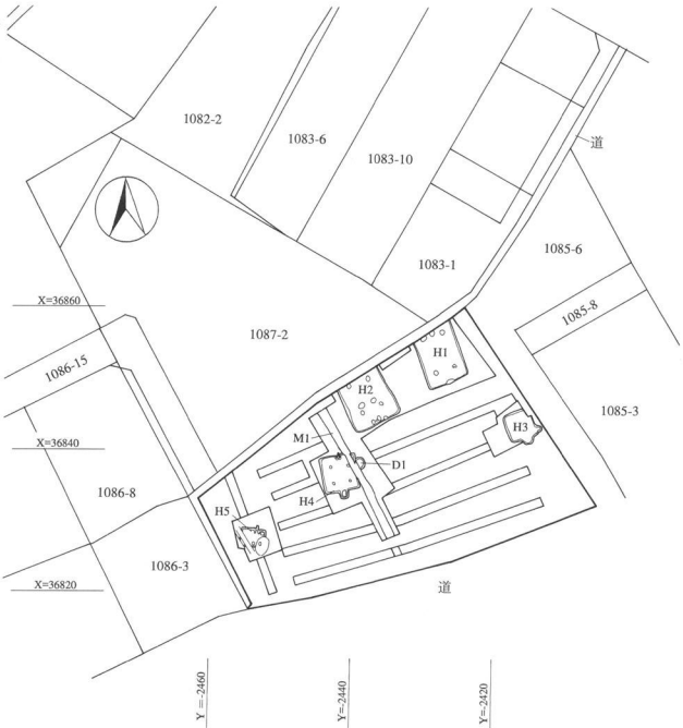
試掘トレンチ・遺構配置図(1:1,000)
